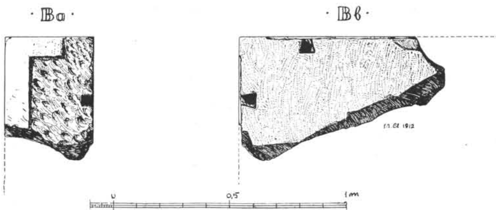
BLOCS DU SOUBASSEMENT.
