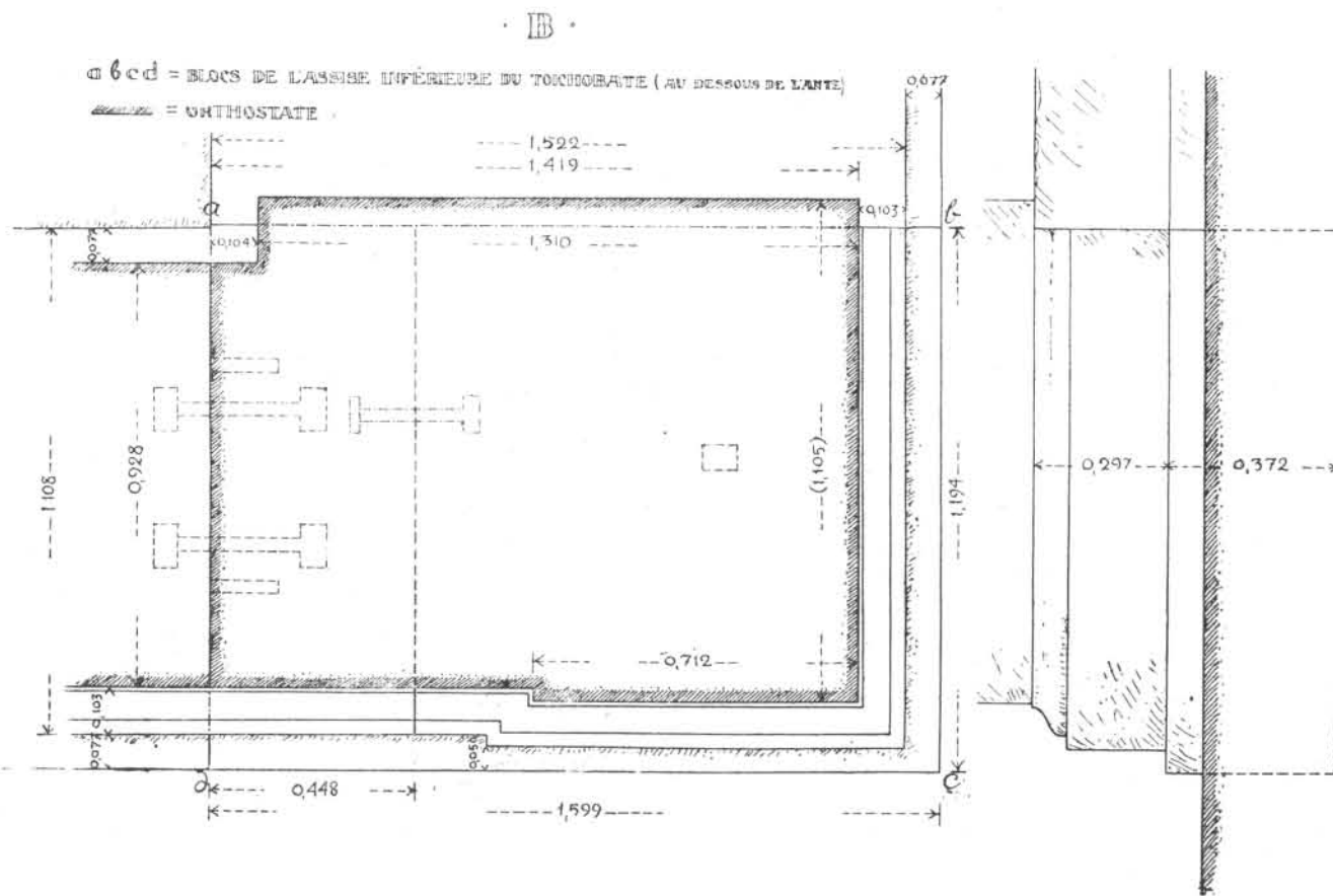
BLOC ET PLAN DU TOICHOBATE.
