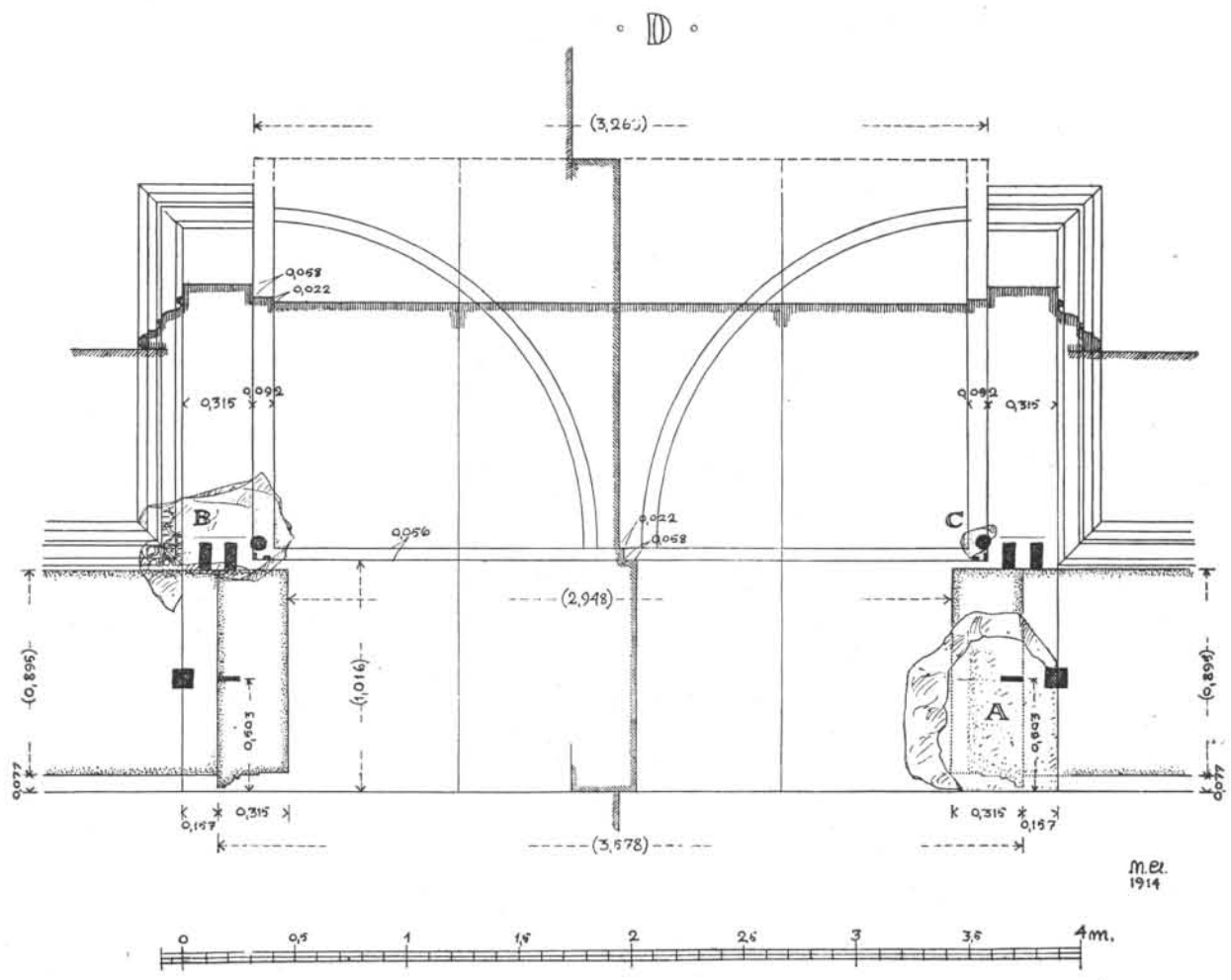
BLOCS DU TOICHOBATE ET PLAN DE LA PORTE.
