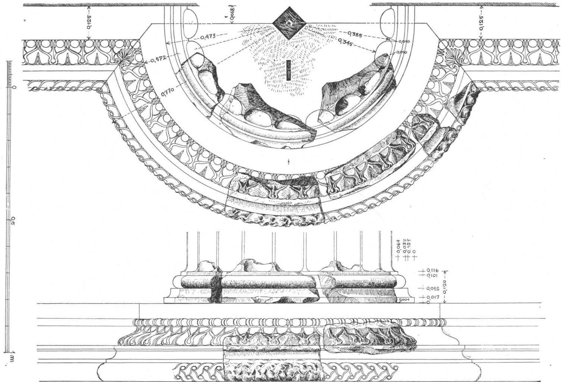
FRAGMENTS DE LA DEMI-COLONNE INTÉRIEURE ET DE L'ASSISE SUPÉRIEURE DU TOICHORATE.
