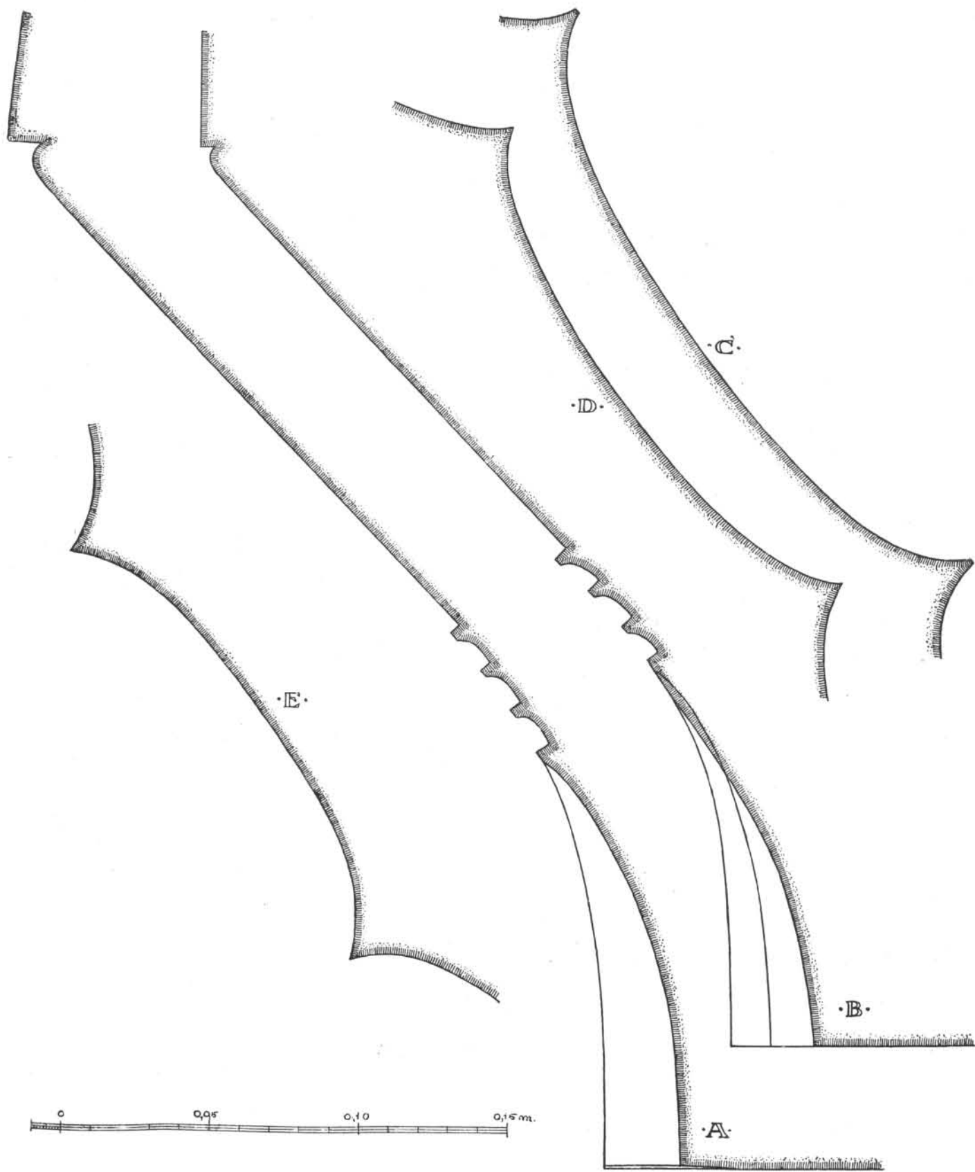
PROFILS DES CHAPITEAUX ET DES CANNELURES DES DEUX ORDRES DORIQUES.
