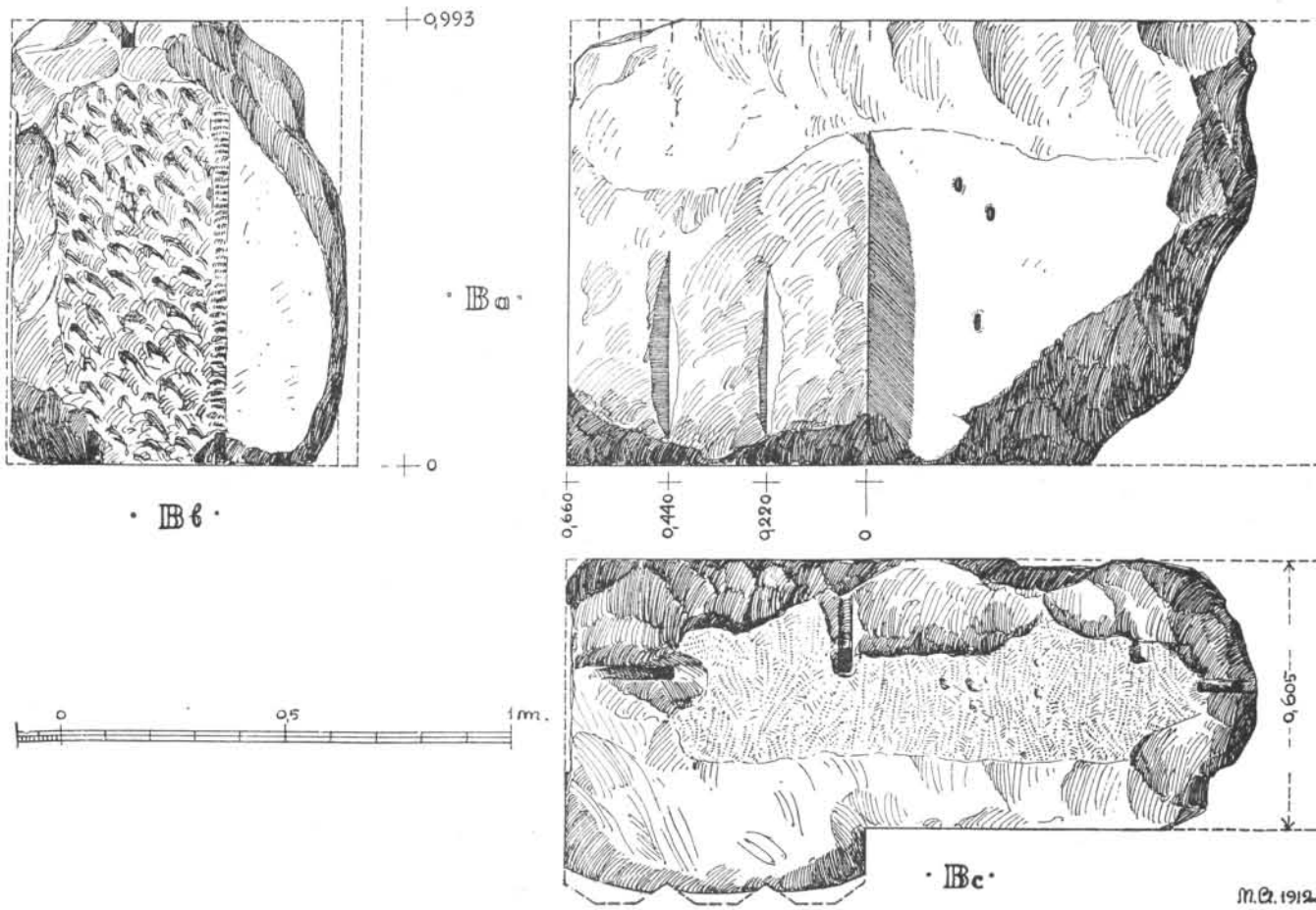
BLOCS DES FRISES DE L'OPISTHODOME ET DU PRONAOS.
