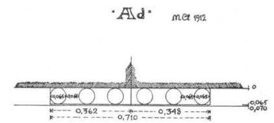
BLOCS DE L'ARCHITRAVE ET DE LA FRISE DE L'ORDRE EXTÉRIEUR.
