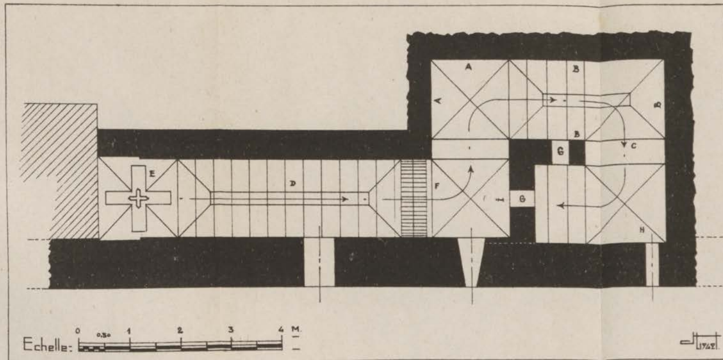
Fig. 85. — Qasba des Oudaia. Escalier des Pirates. Plan du départ et de la partie supérieure.
