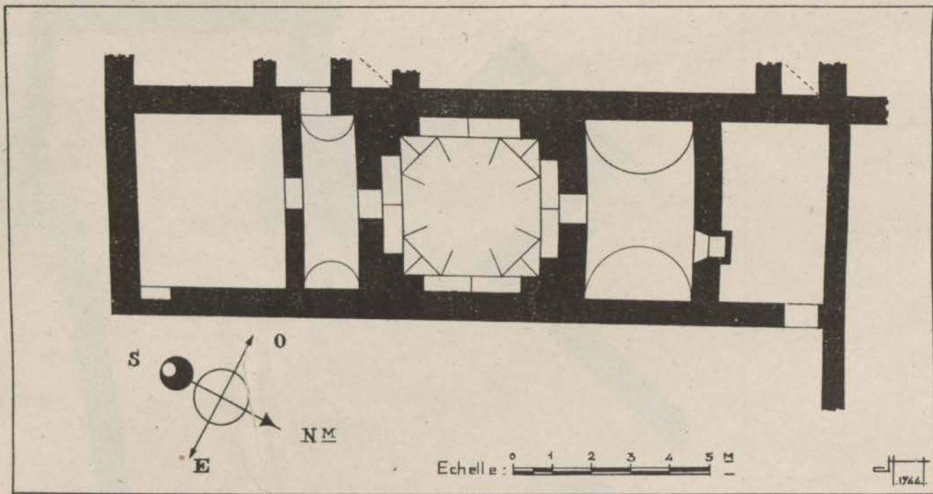
FIG. 109. — Qasba des Oudaia. Bâtiment du musée. Plan du hammam, dans son état primitif.
