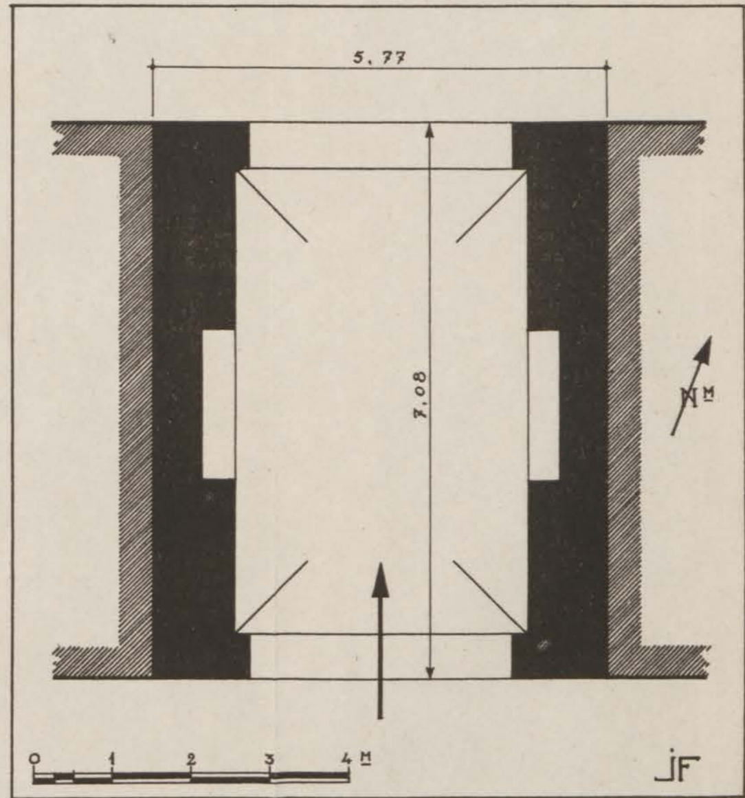
FIG. 131. — Porte du marché, dite Tequisset Dar er-Raf. Plan.
