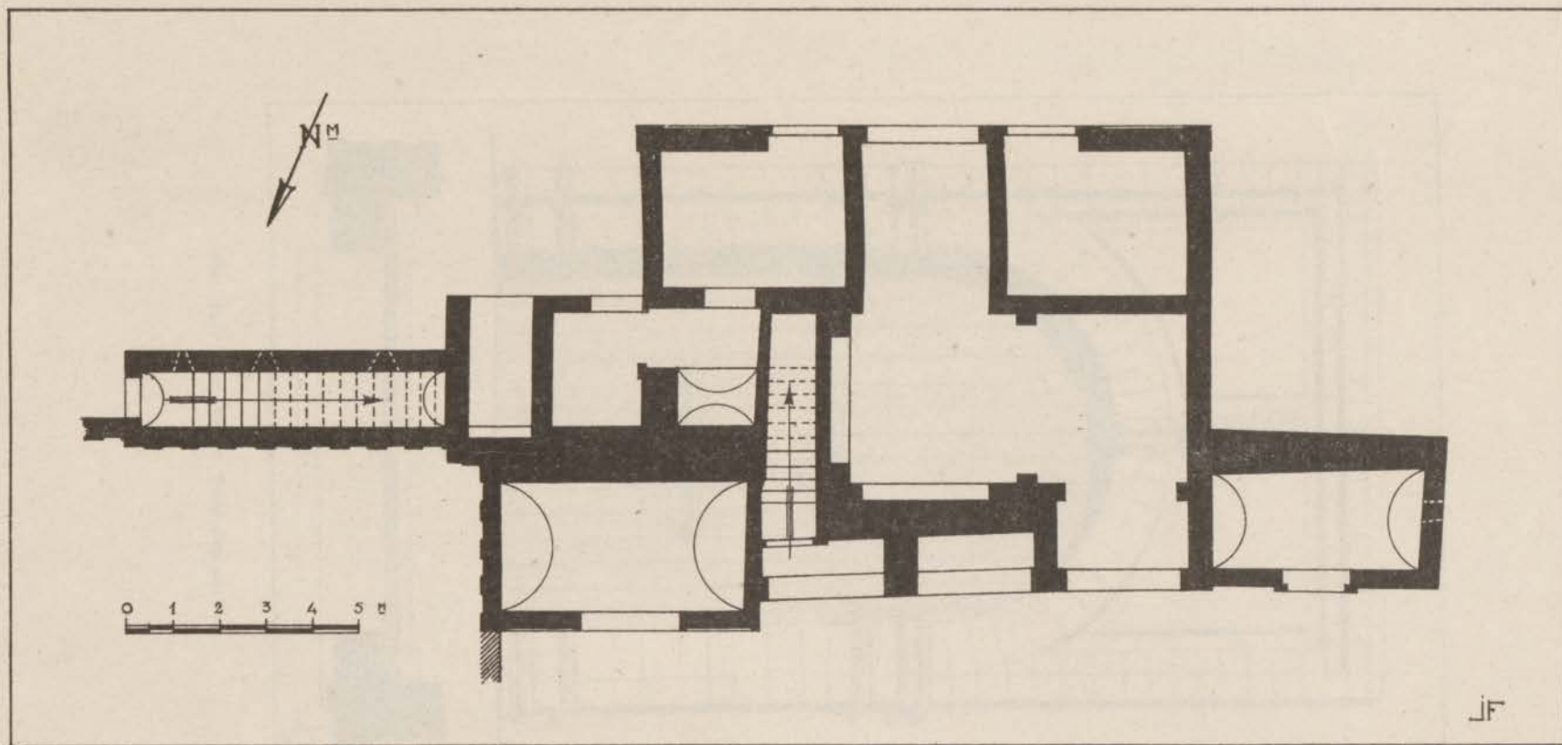
FIG. 173. — Dar Qebibat. Plan du rez-de-chaussée d'un pavillon.
