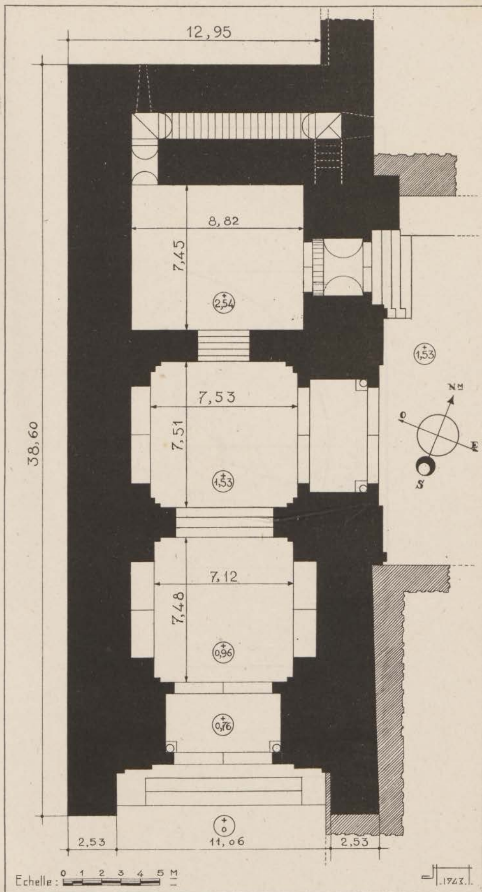
FIG. 11. — Qasba des Oudaia. Grande Porte. Plan du rez-de-chaussée.
