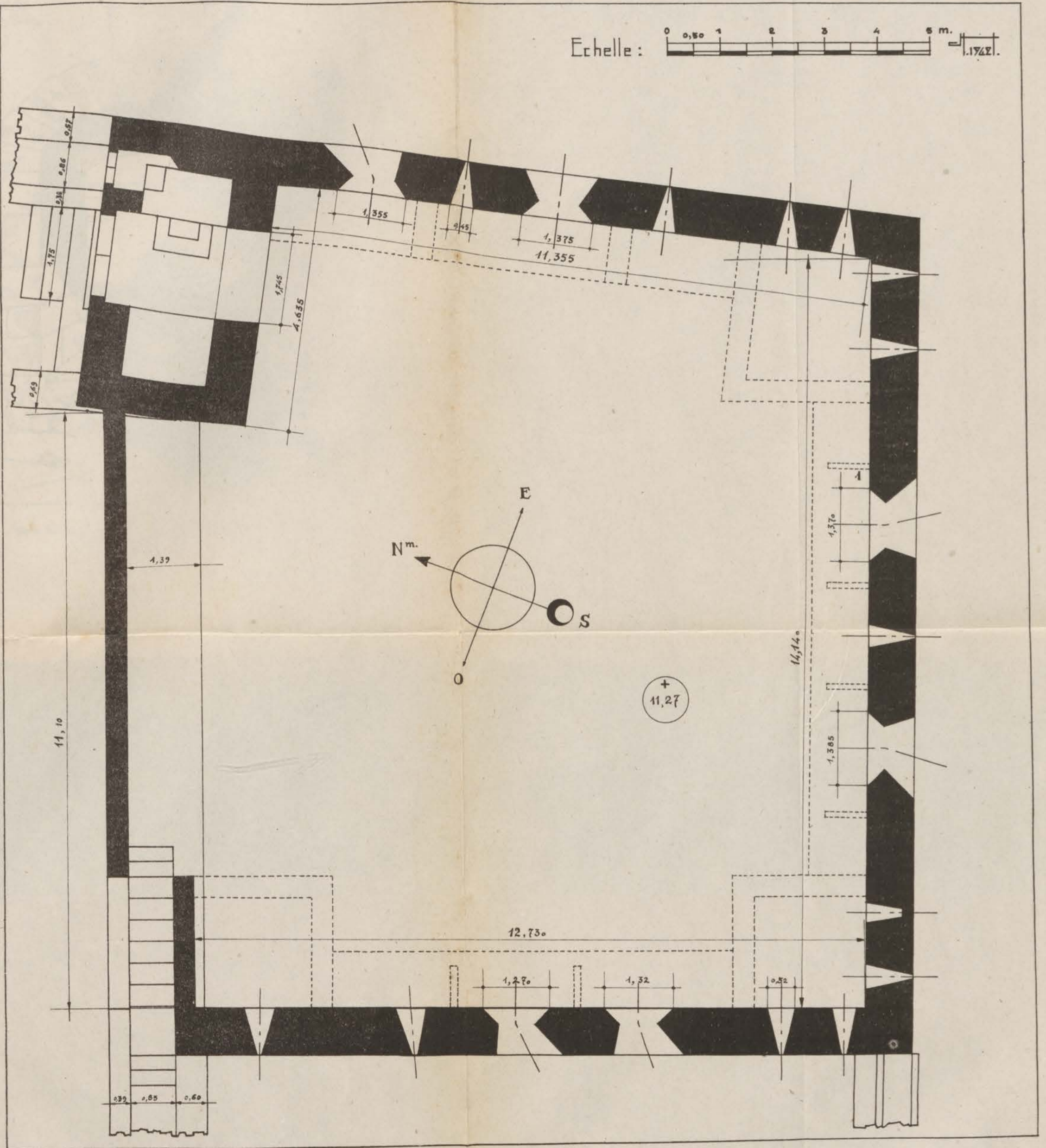
FIG. 105. — Qasba des Oudala. Enceinte de Moulay er-Rechid. Bastion trapézoïdal. Plan.
