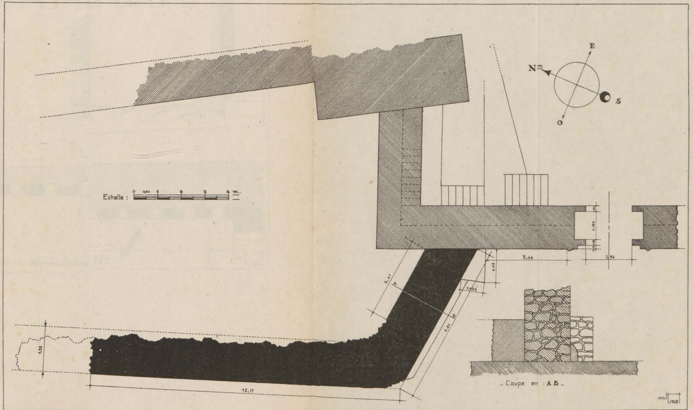
FIG. 2. — Mur en ruines, présumé almoravide, place du Souq el-Ghezal. Plan et coupe.
