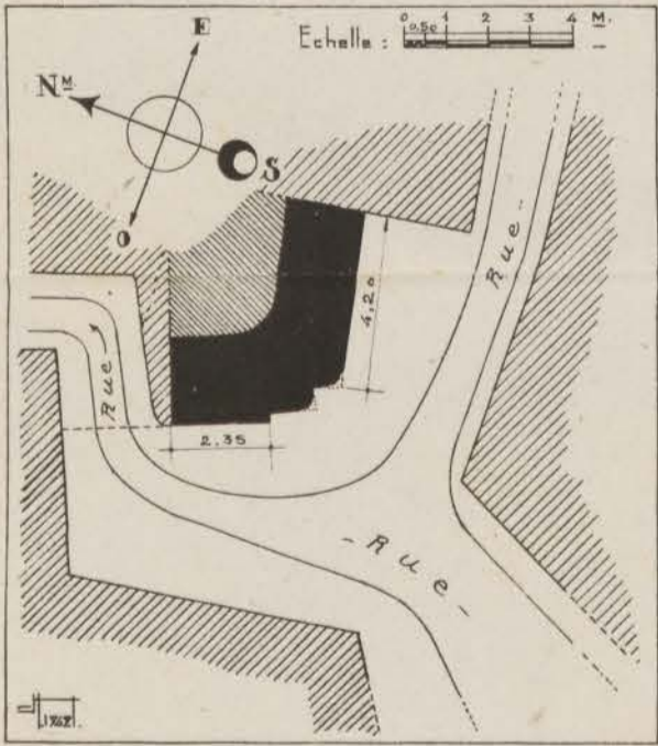
FIG. 29. — Qasba des Oudaïa. Vestiges almohades, rue Bazzo. Plan.
