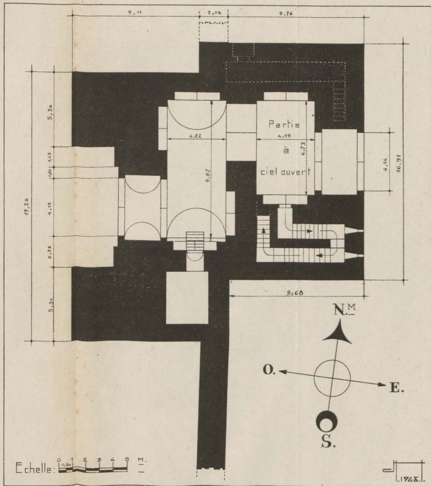
FIG. 33. — Enceinte almohade de la ville de Ribat el-Fath. Bab el-Alou. Plan du rez-de-chaussée.
