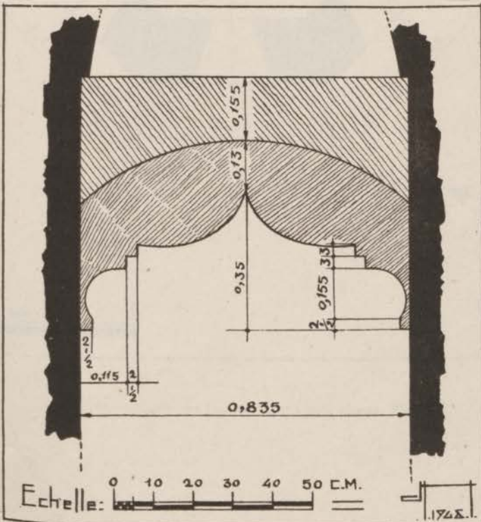
FIG. 81. — Qasba des Oudaïa. Tour des Pirates. Arc en accolade de l'escalier intérieur.
