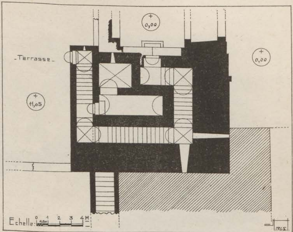
FIG. 39. — Enceinte almohade de la ville de Ribat el-Fath. Bab er-Rouah. Plan des pièces intermédiaires.
