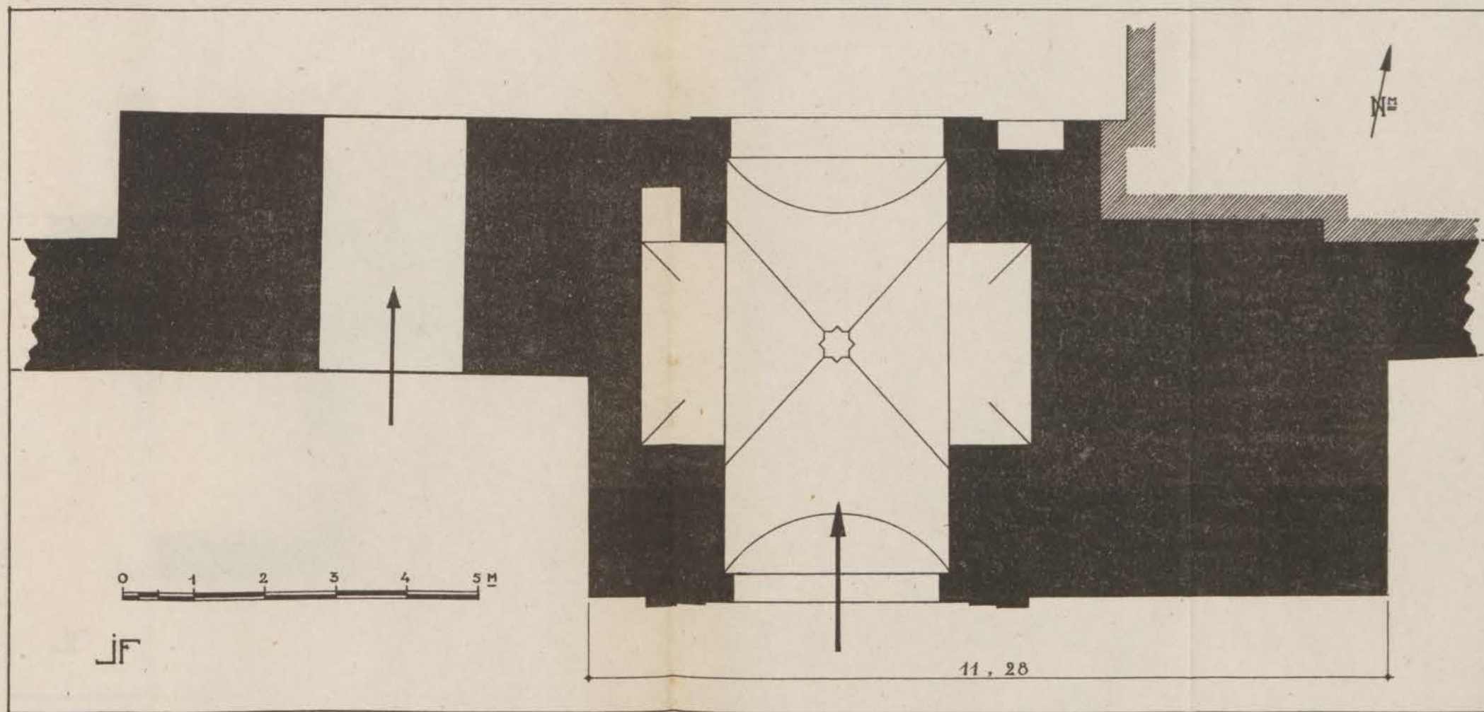
FIG. 133. — Bab Chella, porte alaouite de l'enceinte andalouse de la médina. Plan du rez-de-chaussée.
