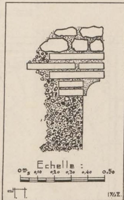
FIG. 148. — Jama Molina. Corniche des murs de l'oratoire: Détail de la bâtisse.
