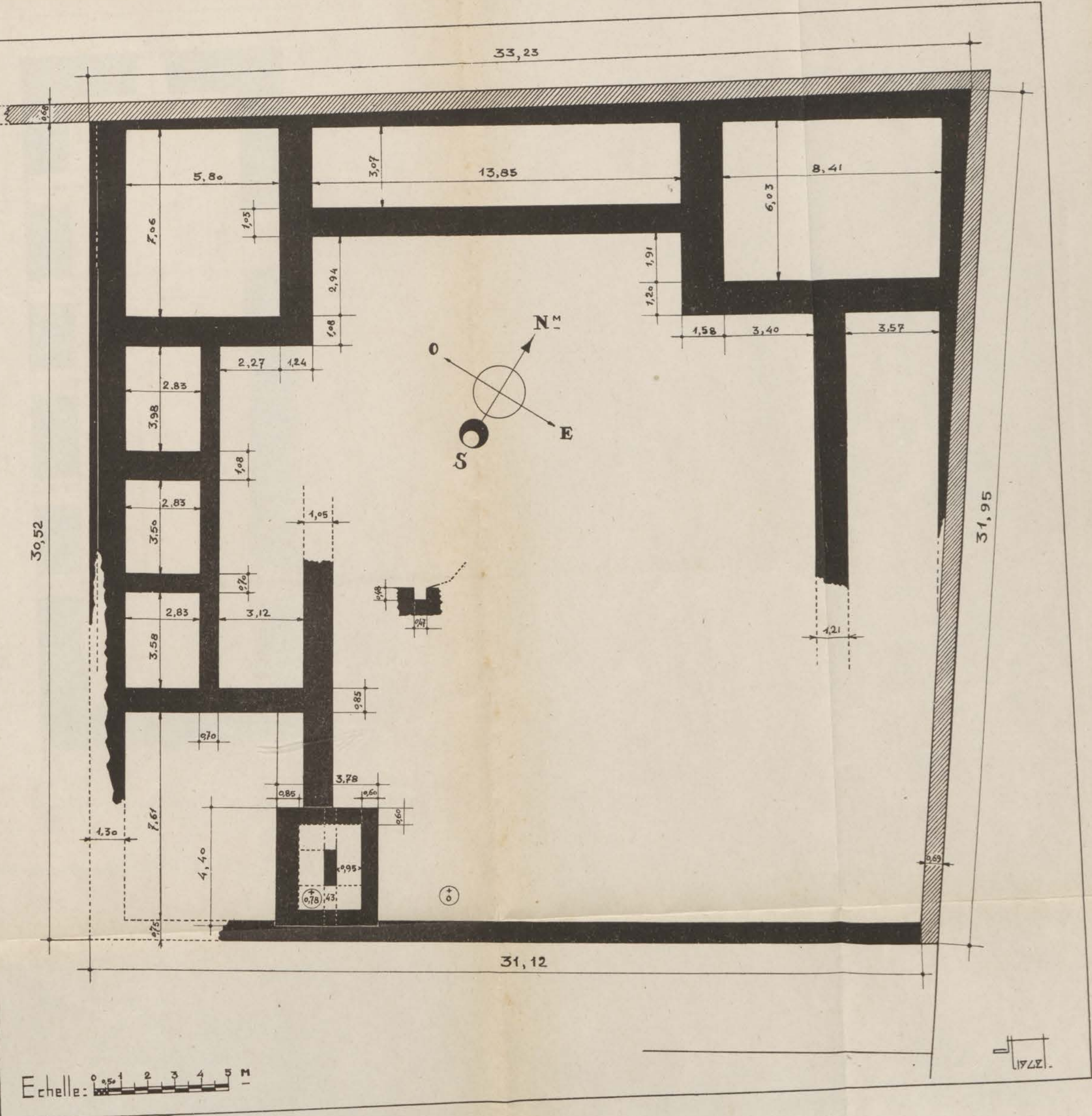
FIG. 111. — Qasba des Oudaja. Vestiges de la plate-forme du Sémaphore. Plan.
