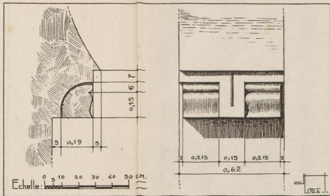
FIG. 15. — Qasba des Oudaia. Grande Porte. Surabaque des arcs.
