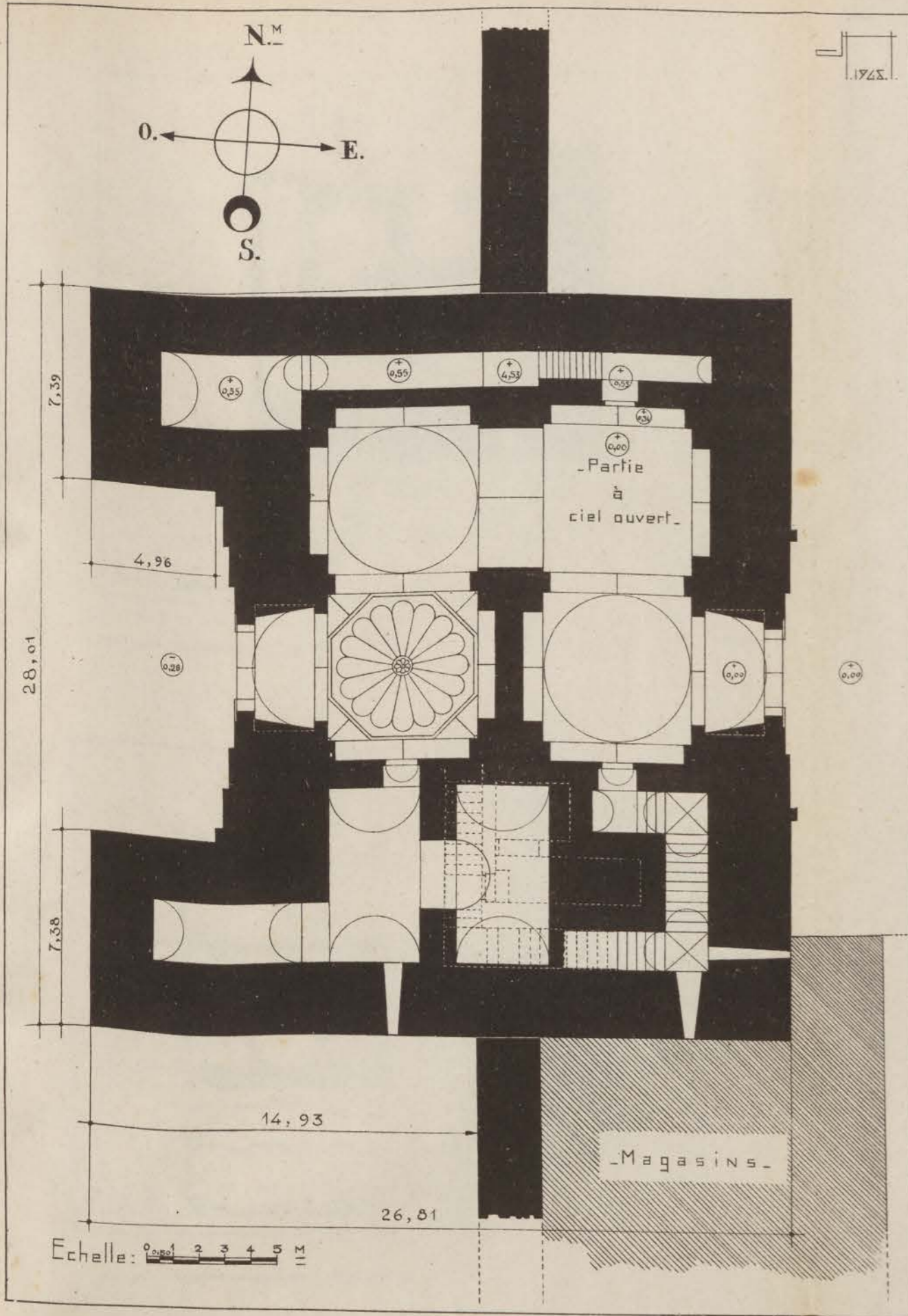
FIG. 37. — Encinte almohade de la ville de Ribat el-Fath. Bab er-Rouah. Plan du rez-de-chaussée.
