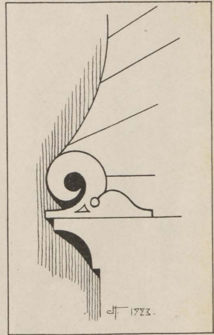
FIG. 62. — Mosquée de Hassan. Minaret. Départ d'arc au panneau inférieur de la face sud.
