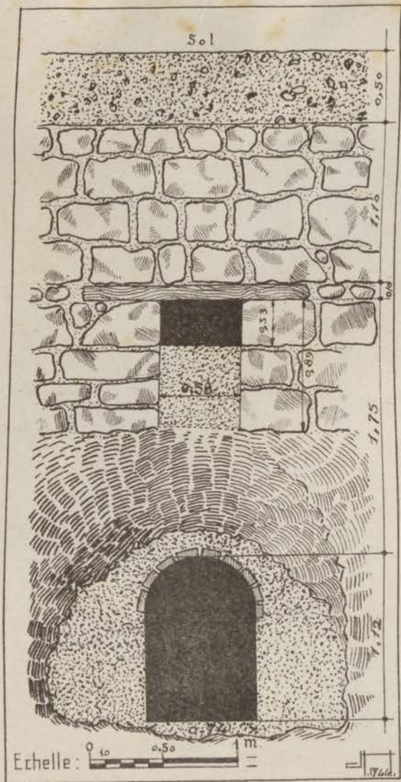
FIG. 56. — Mosquée de Hassan. Canaux souterrains partant du sahn latéral est.
