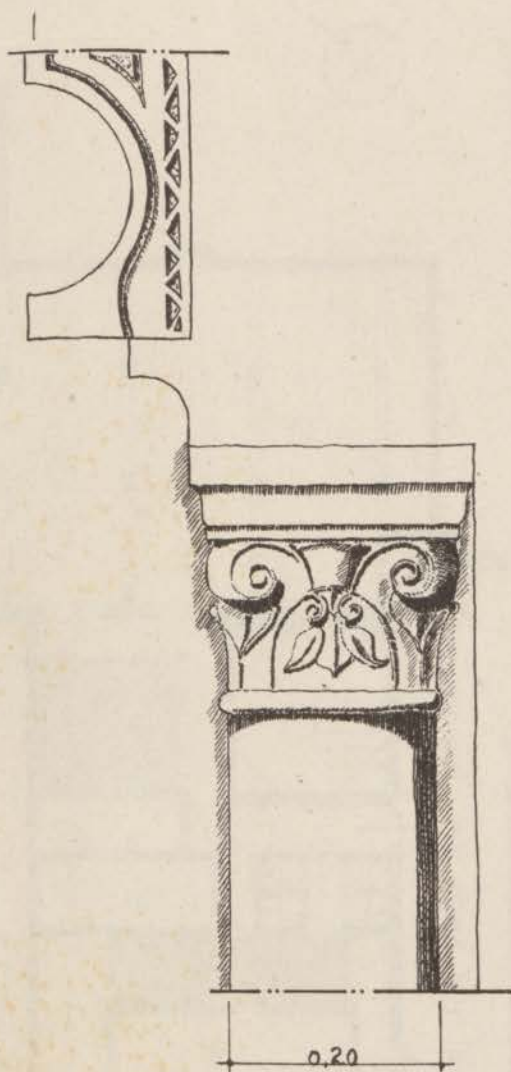
FIG. 169. — Jama en-Nekhla. Chapiteau et départ de l'arc du mihrab.
