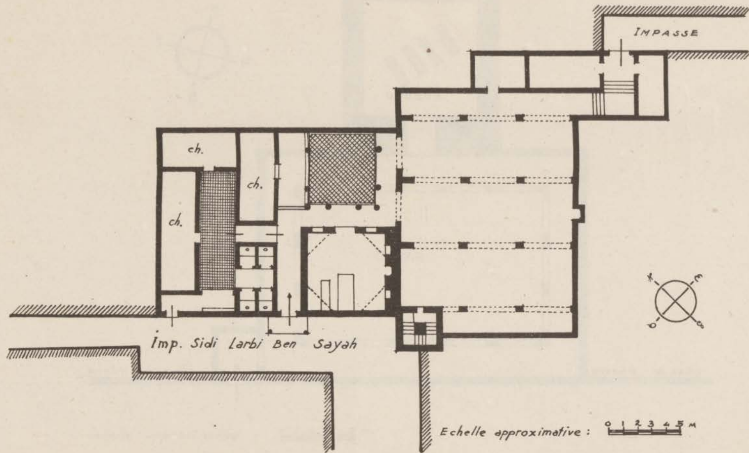
FIG. 170. — Zaouia de Sidi Larbi ben Sayah. Plan.
