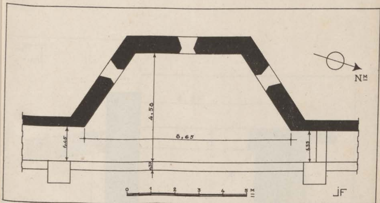
FIG. 128. — Bastion alaouite de l'enceinte almohade de la ville de Ribat el-Fath. Plan.
