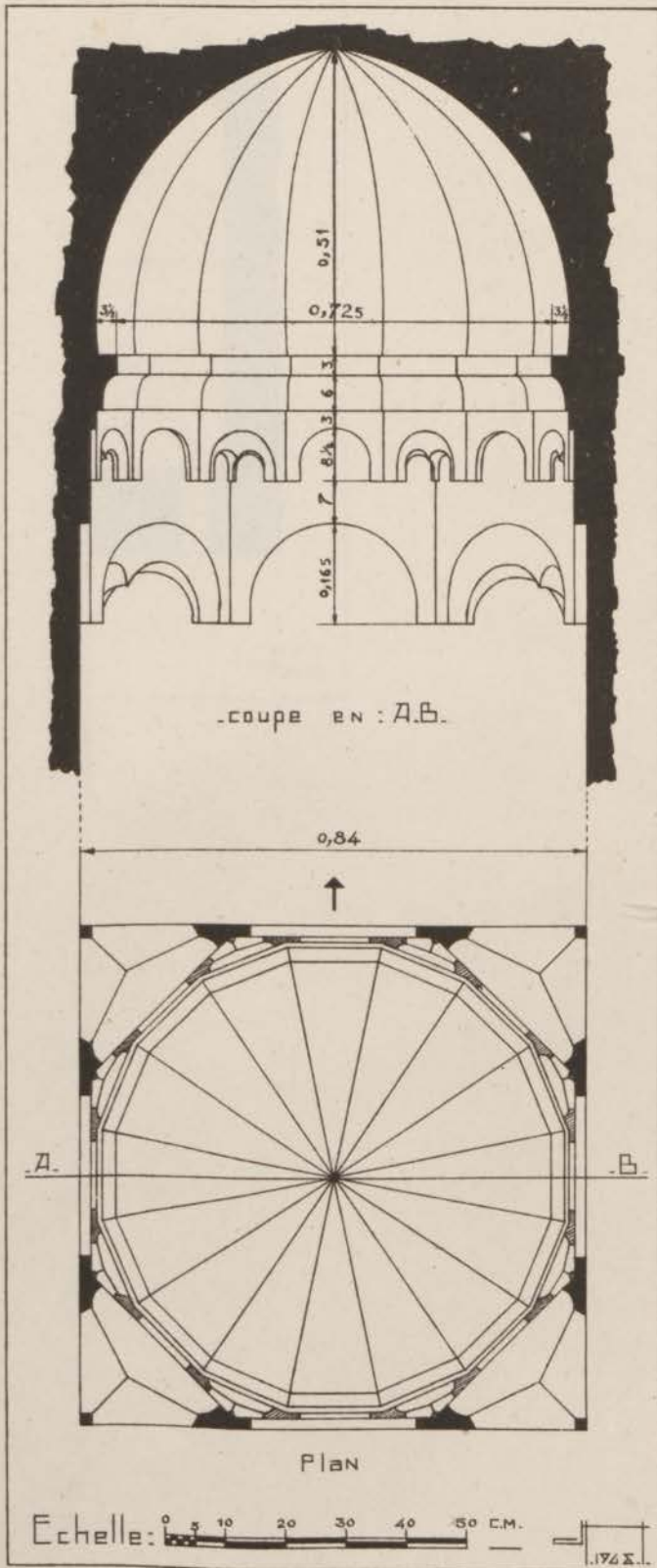
FIG. 84. — Qasba des Oudaia. Tour des Pirates. Coupole de l'escalier intérieur. Plan et coupe.
