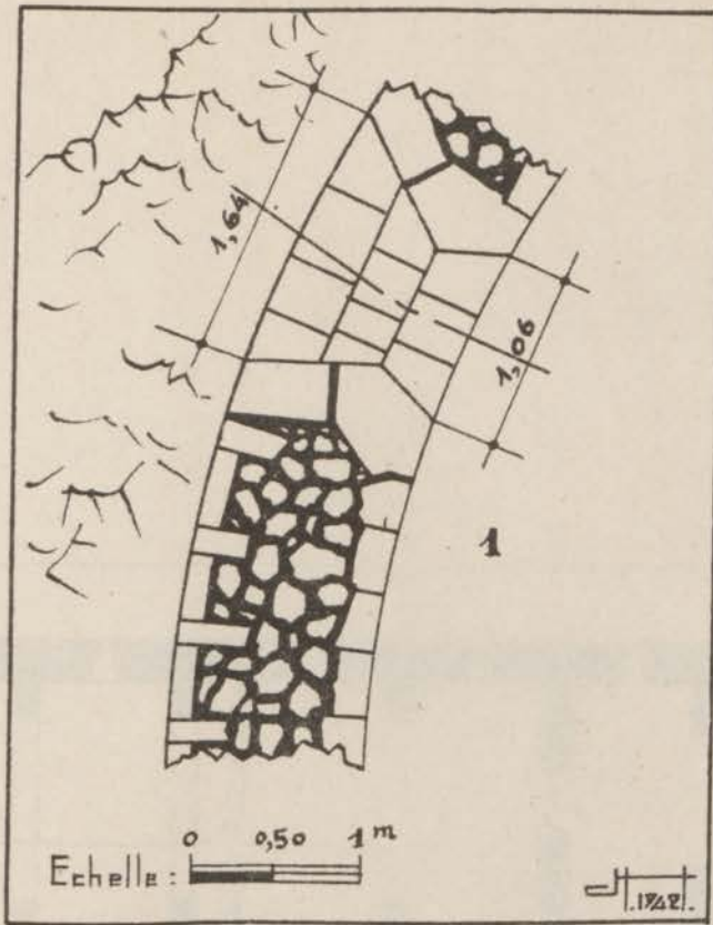
FIG. 114. — Qasba des Oudaïa. Borj circulaire. Détail de la bâtisse.
