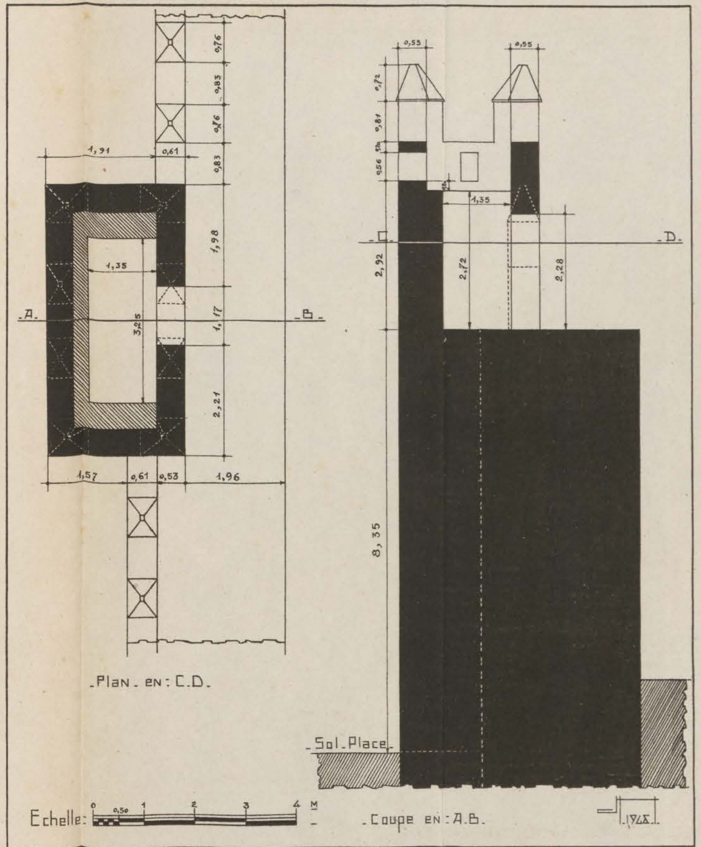
FIG. 5. — Qasba des Oudaya. Enceinte almohade. Tour barlongue, place du Souq el-Ghezal. Plan et coupe.
