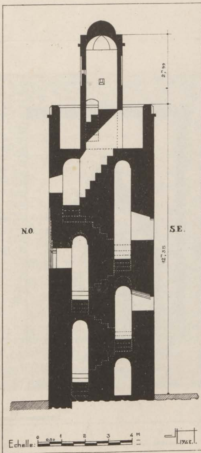
FIG. 151. — Jama Molina. Minaret. Coupe.
