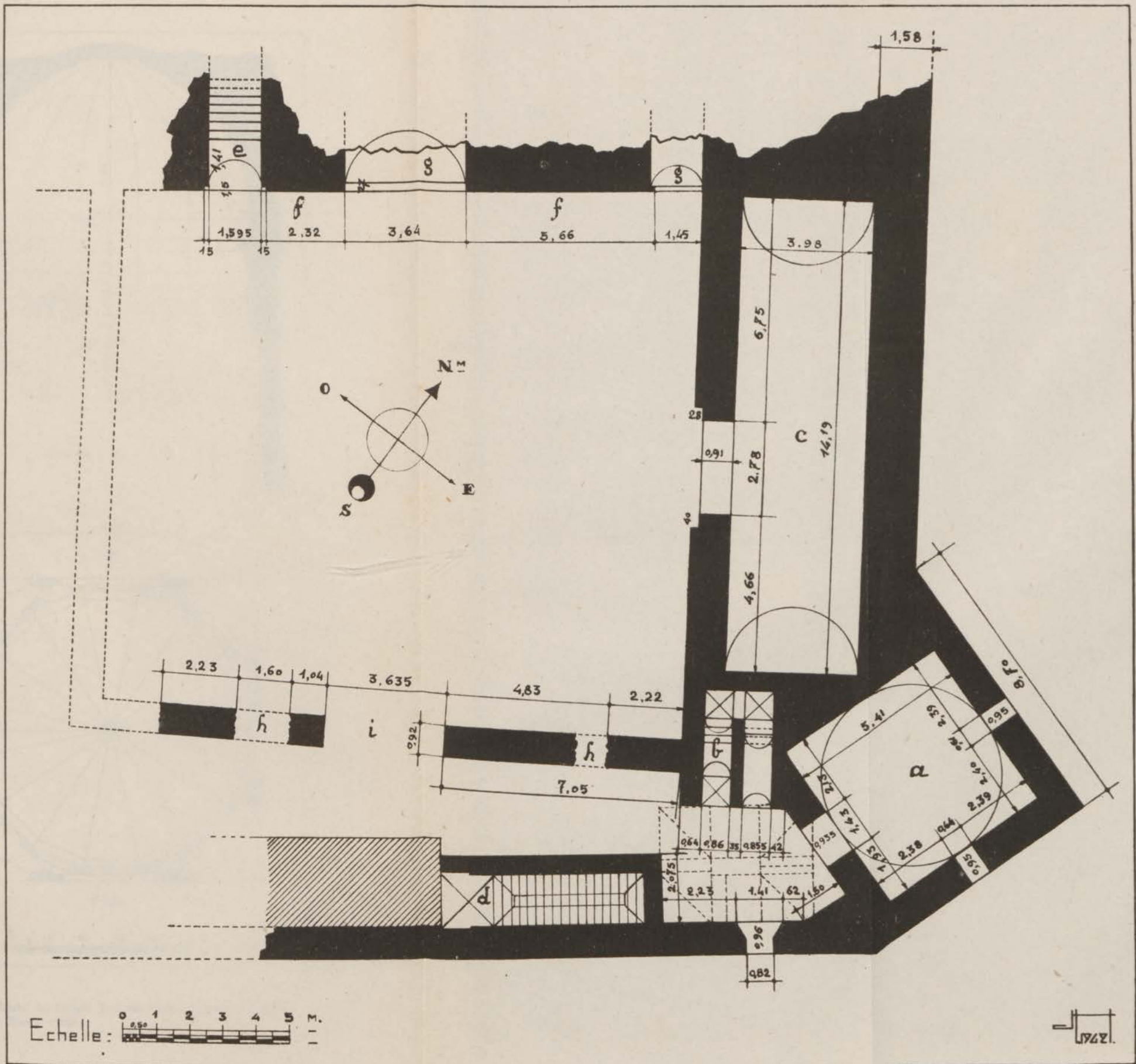
FIG. 83. — Qasba des Oudaia. Tour des Pirates, escalier des Pirates, constructions et ruines voisines. Plan d'ensemble.
