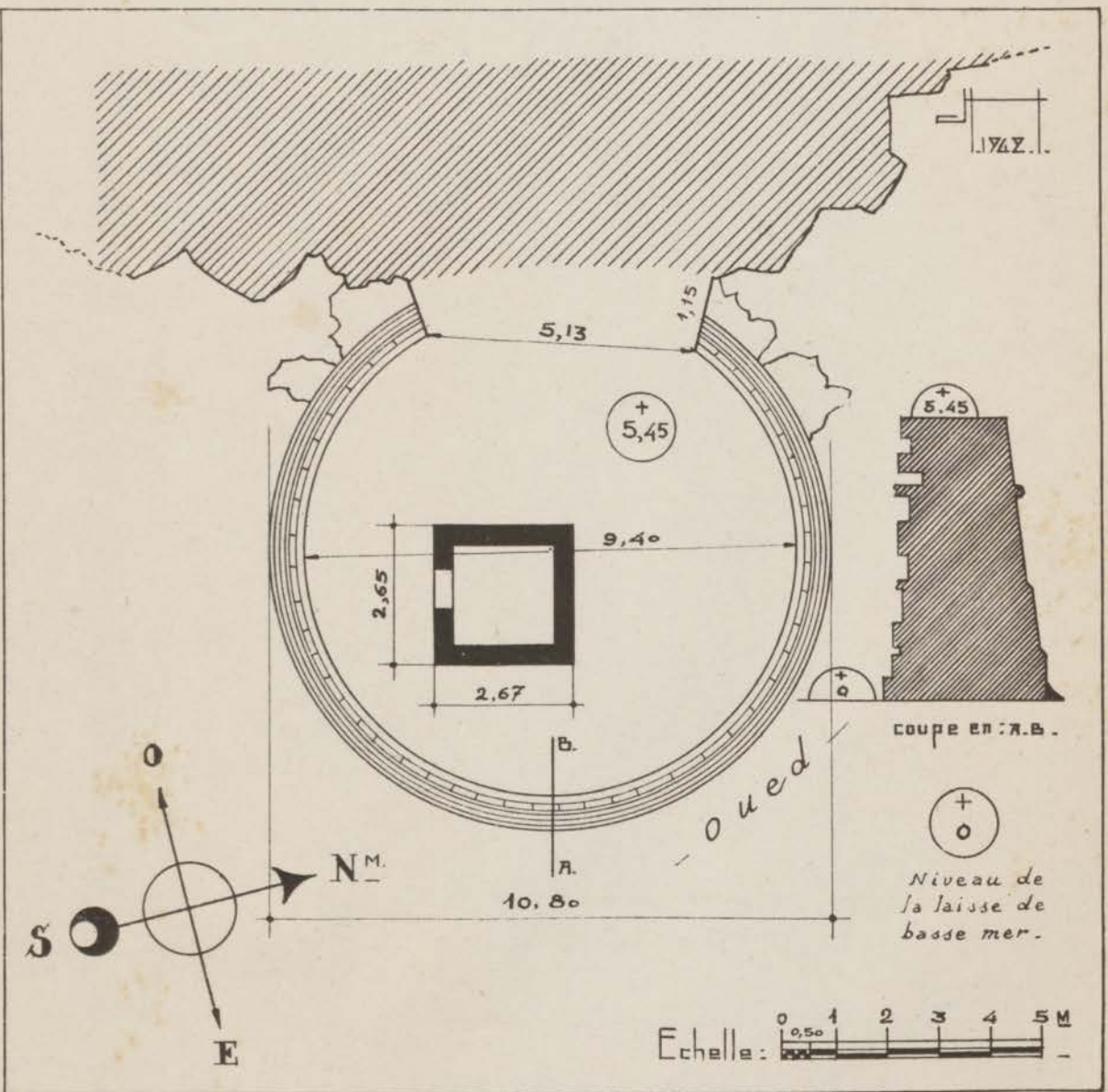
Fig. 180. — La Mdoura. Plan et coupe.
