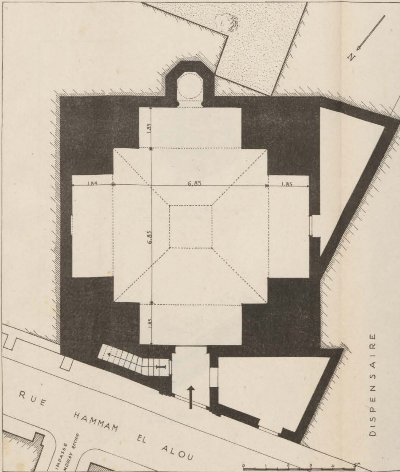
FIG. 164. — Jama el-Qoubba. Plan.
