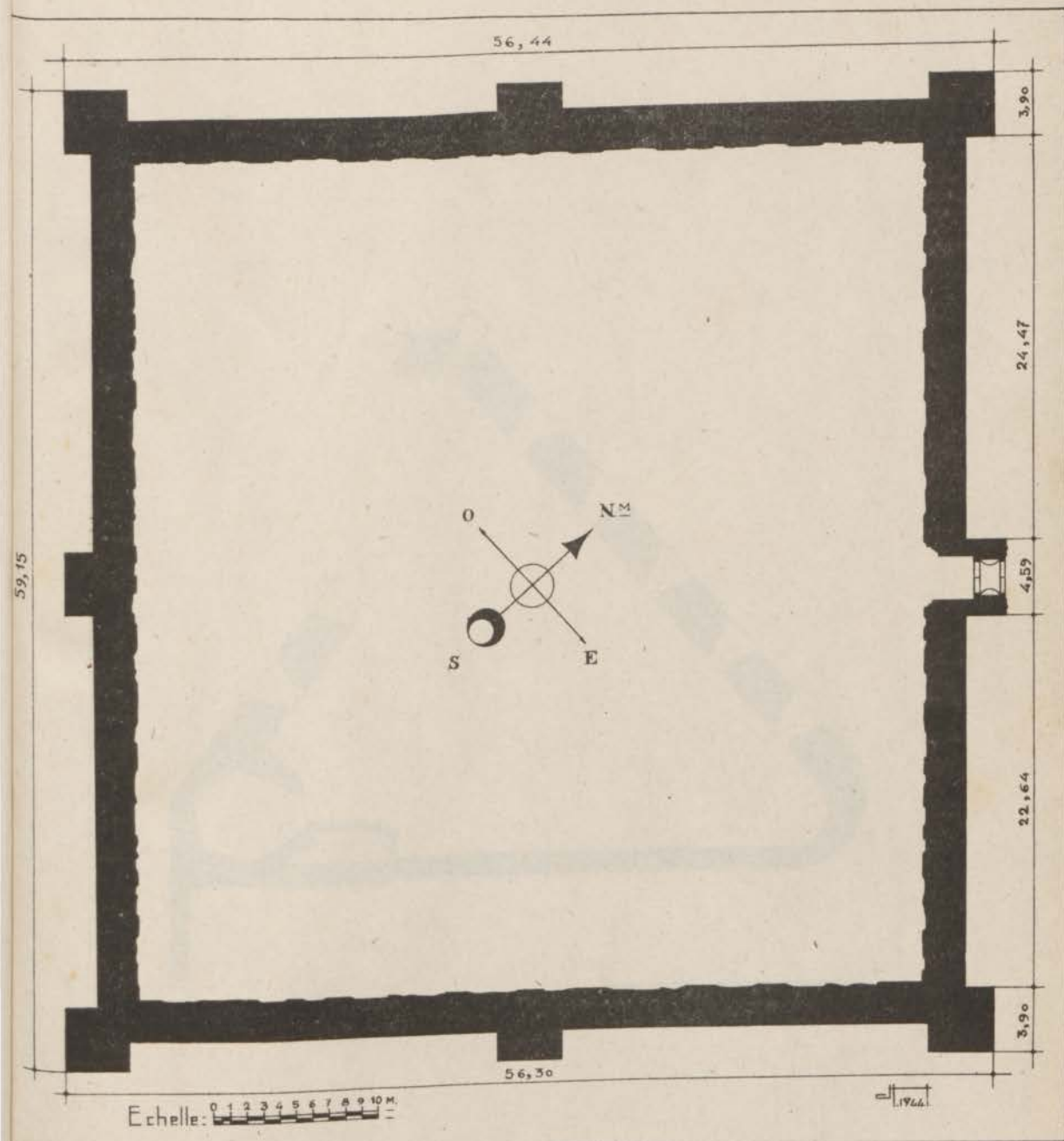
FIG. 119. — Château-neuf de Moulay er-Rechid. Plan.
