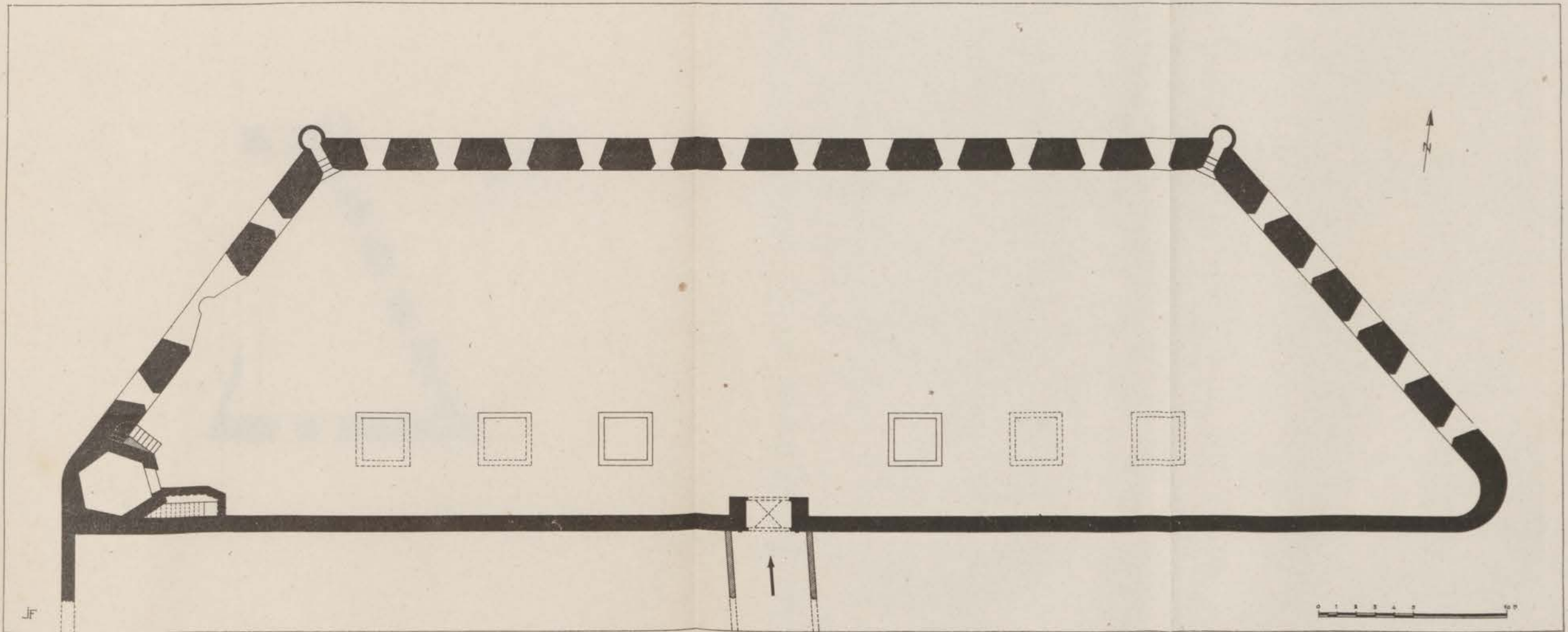
FIG. 120. — Borj es-Sirat. Plan.
