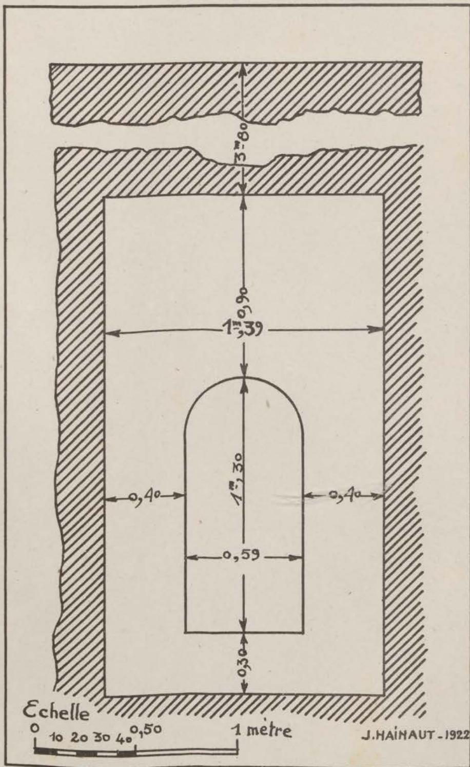
FIG. 54. — Aqueduc almohade de l'Ain Gheboula. Coupe, rue Bab Chella.
