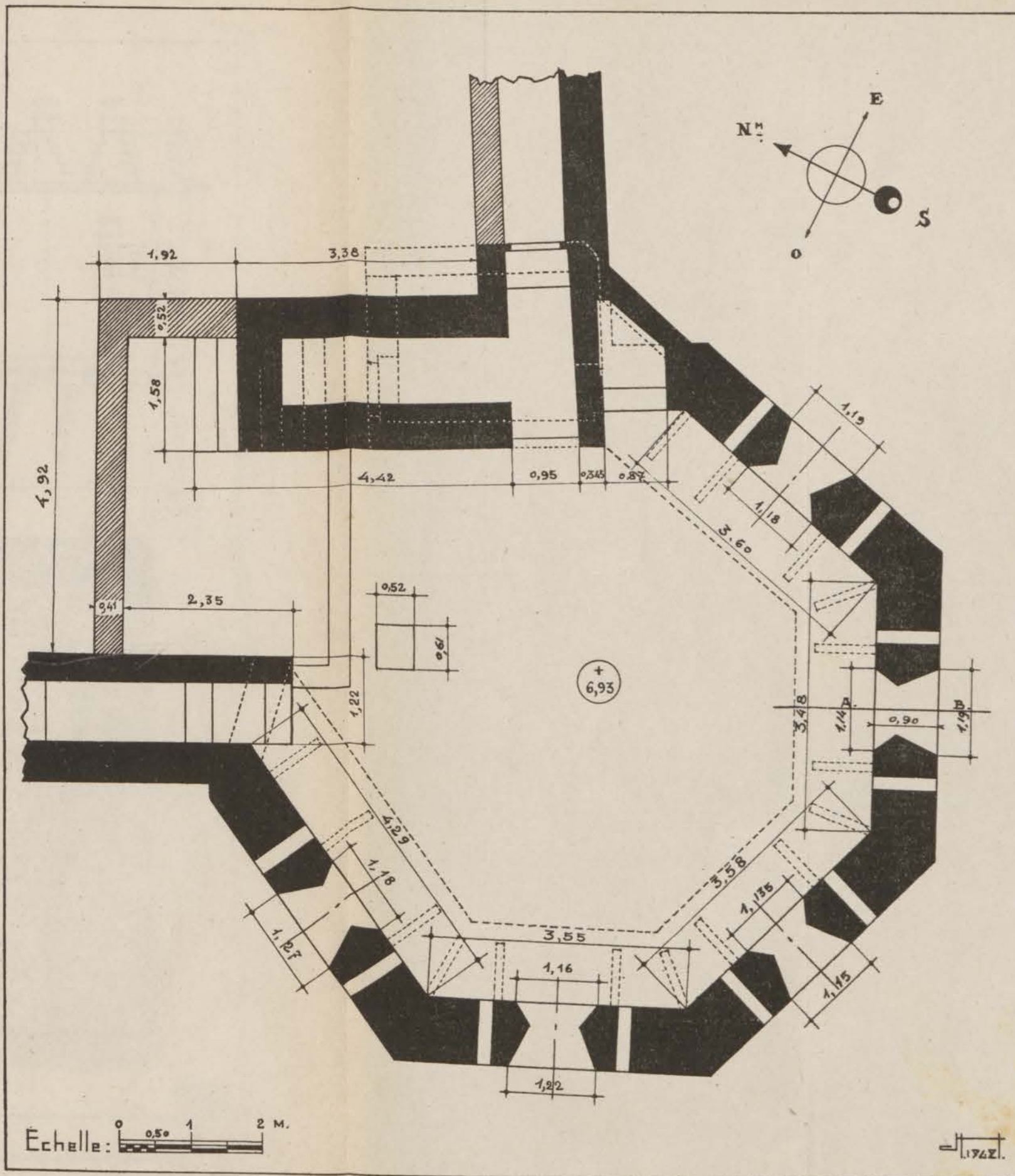
FIG. 101. — Qasba des Oudaia. Enceinte de Moulay er-Rechid. Bastion heptagonal. Plan d'ensemble.
