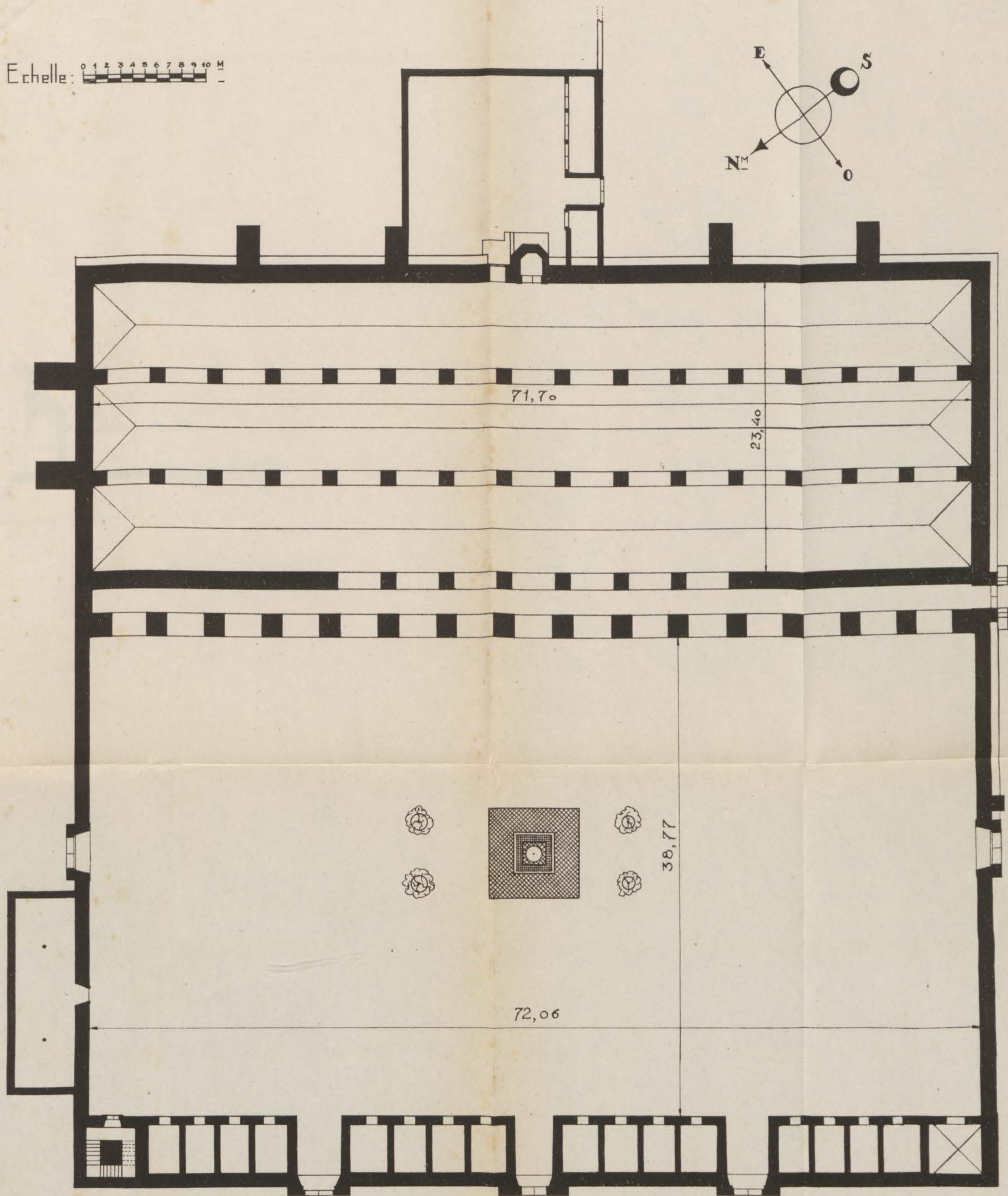
FIG. 135. — Jama es-Sounna. Plan.
