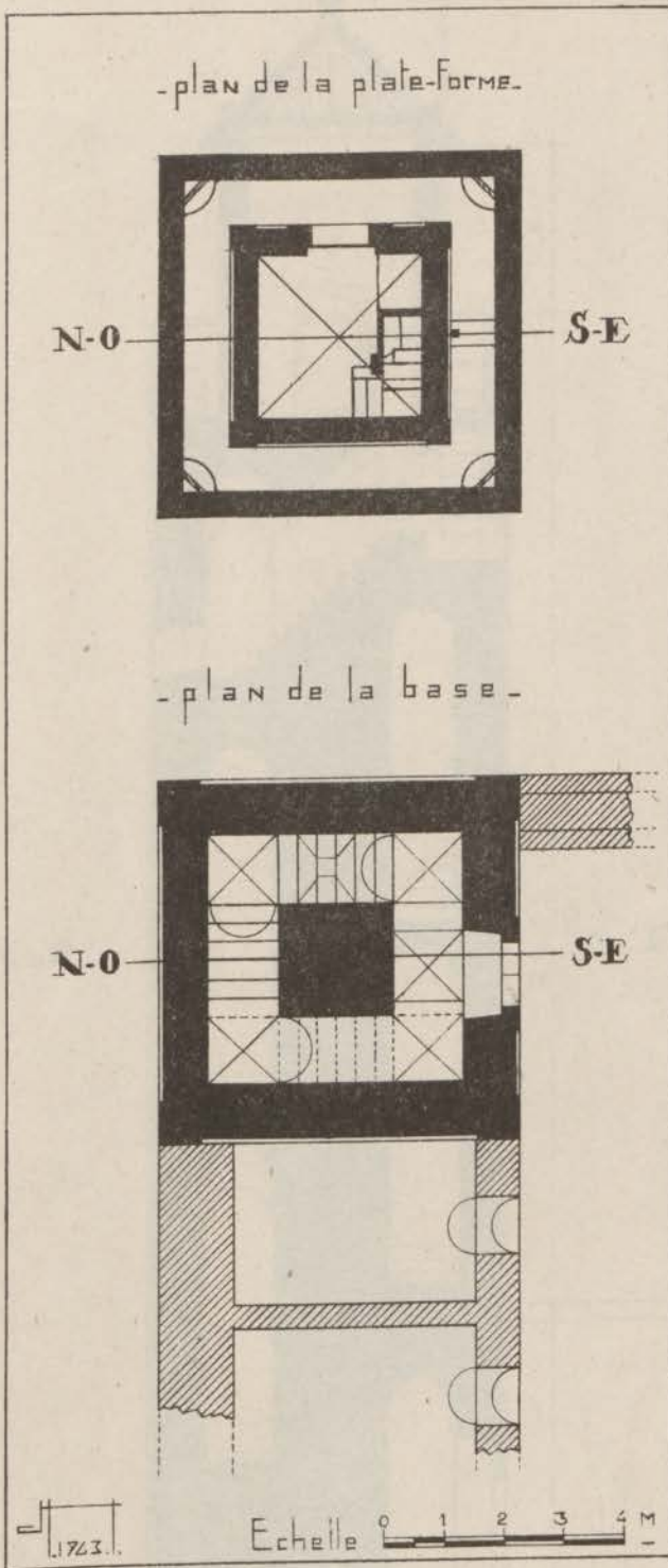
FIG. 137. — Jama es-Sounna. Minaret. Plan.
