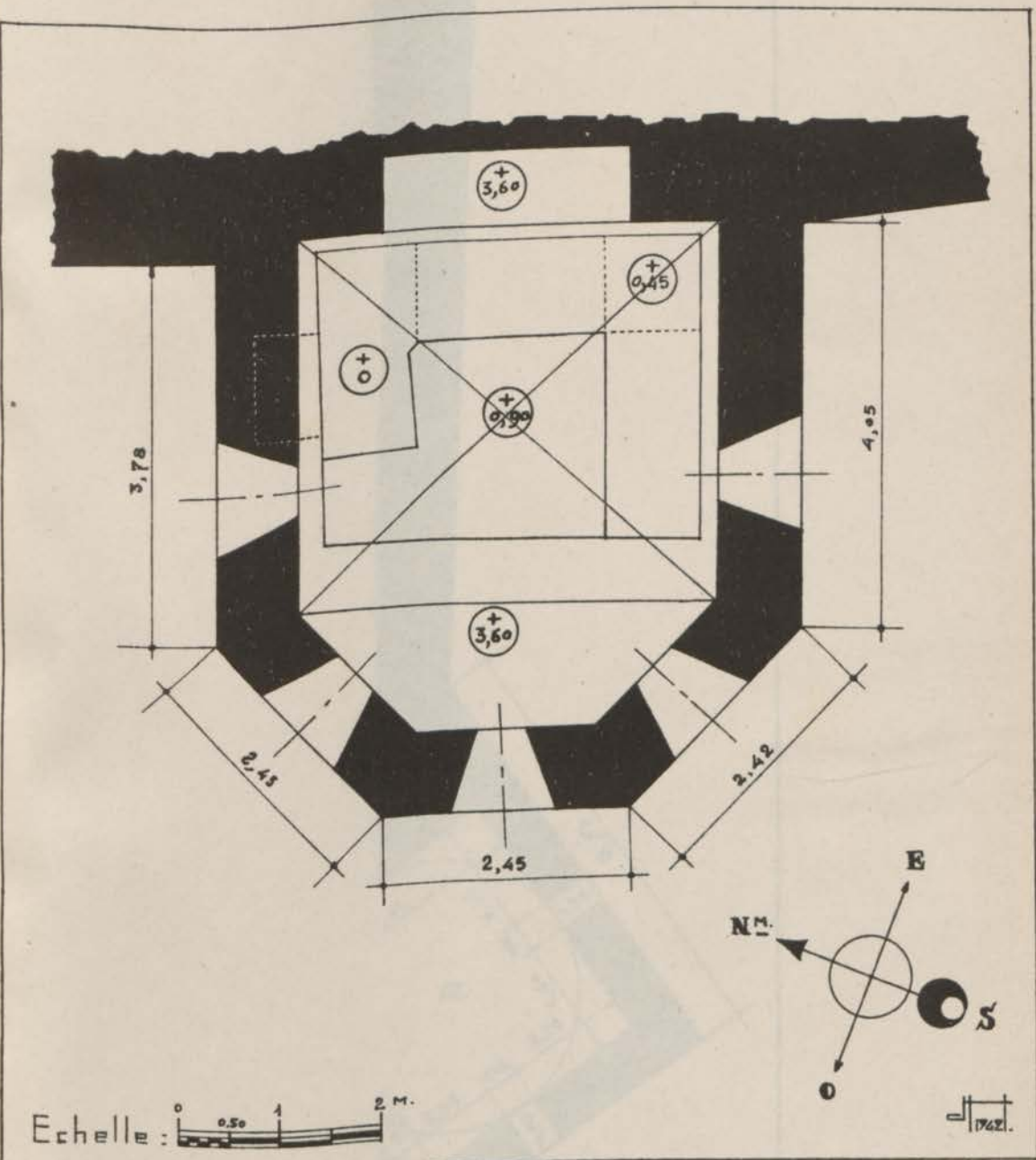
FIG. 82. — Qasba des Oudaia. Tour à pans coupés. Plan.
