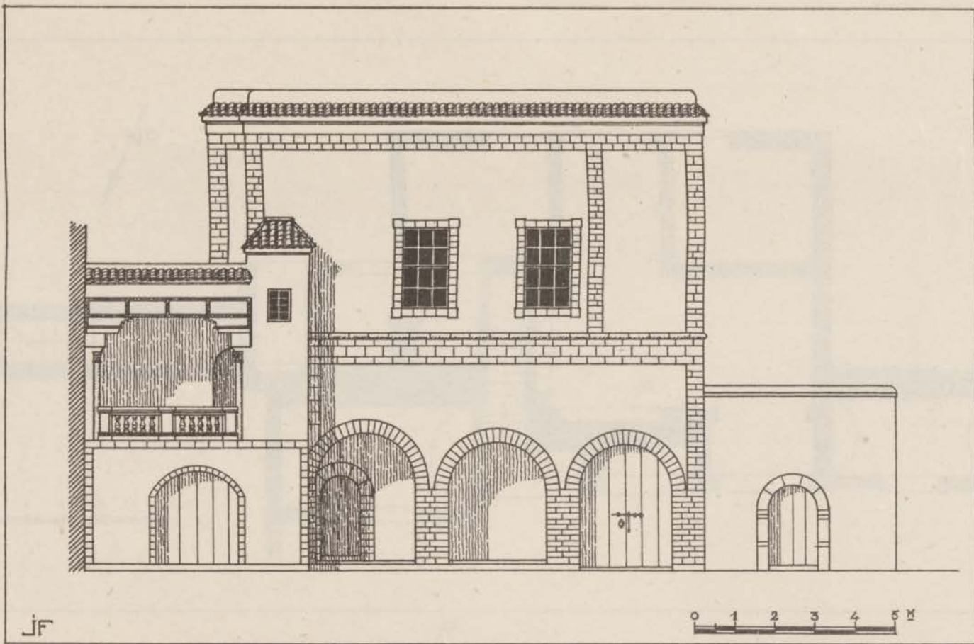
FIG. 172. — Dar Qebibat. Façade d'un pavillon.
