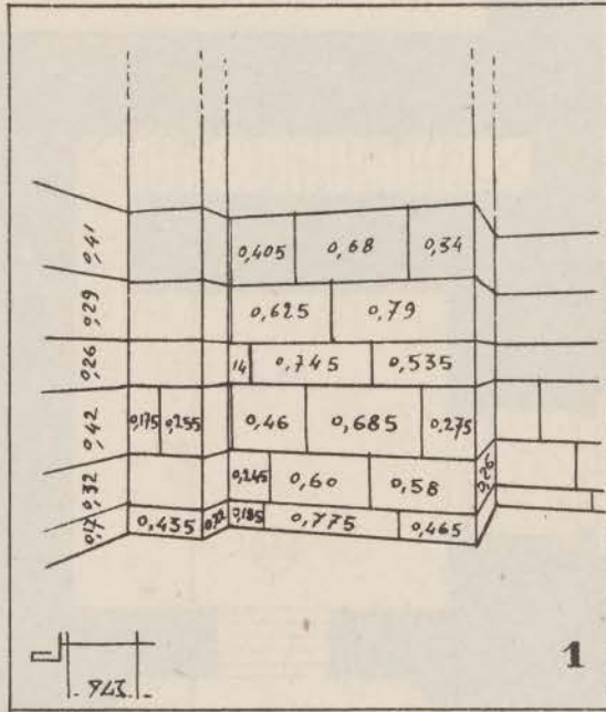
FIG. 9. — Qasba des Oudaïa. Grande Porte. Croquis coté de l'appareil, face extérieure.
