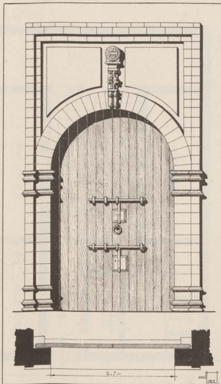
FIG. 174. — Dar Qebibat. Porte d'un pavillon.
