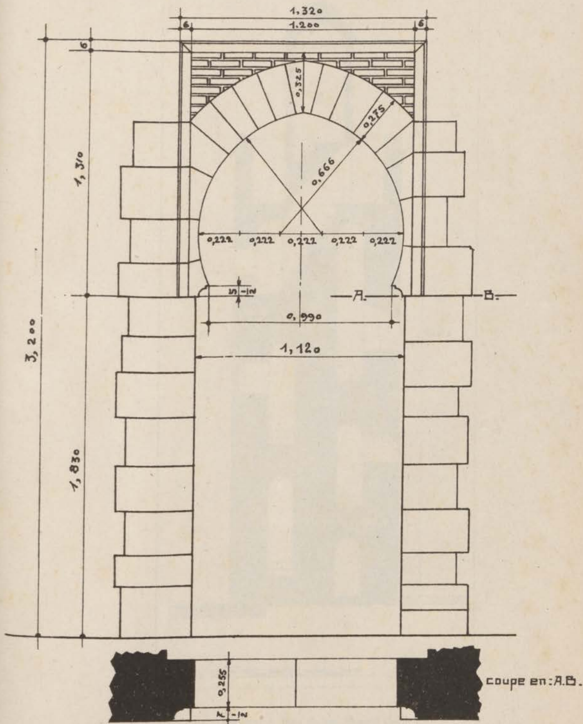
FIG. 150. — Jama Molina. Elévation du mihrab.
