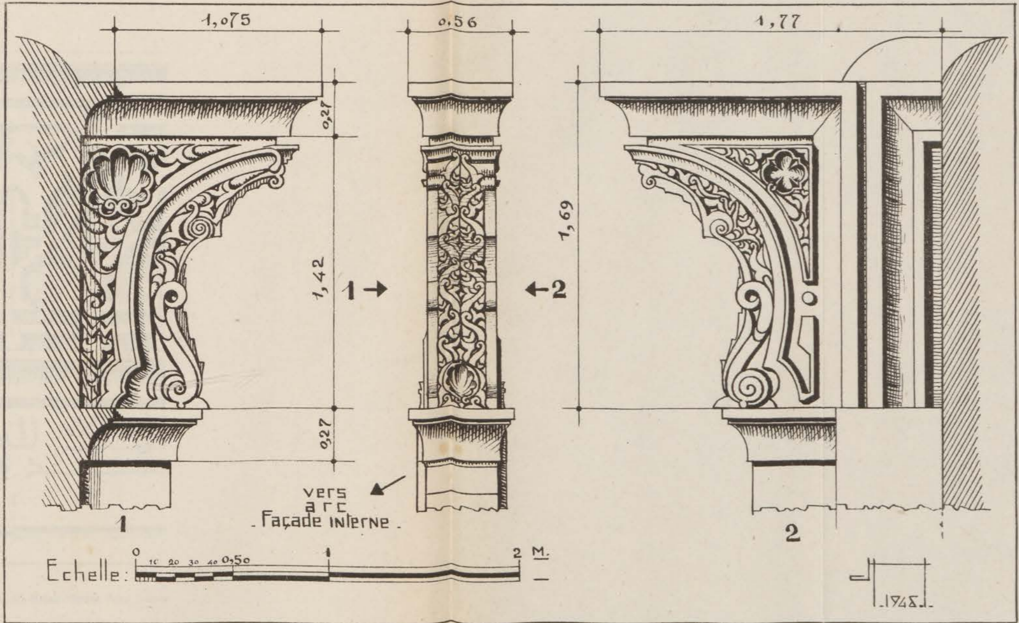
FIG. 22. — Qasba des Oudaïa. Grande Porte. Consoles de la face intérieure.
