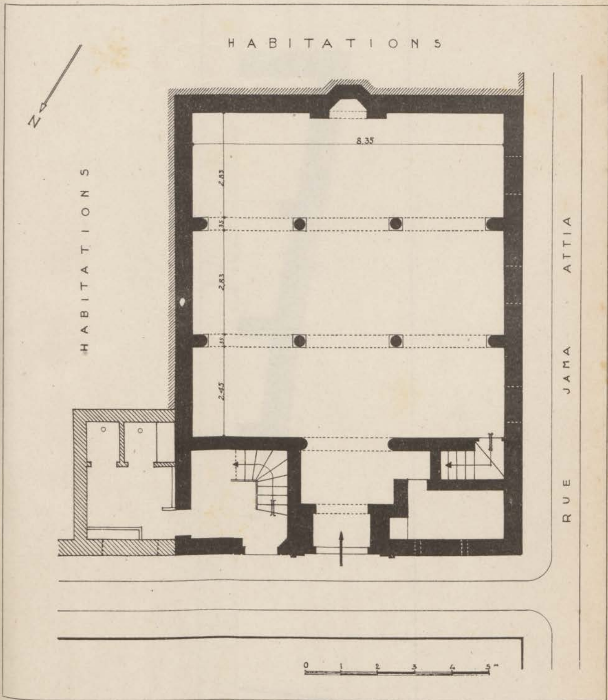
FIG. 162. — Jama Attia. Plan.
