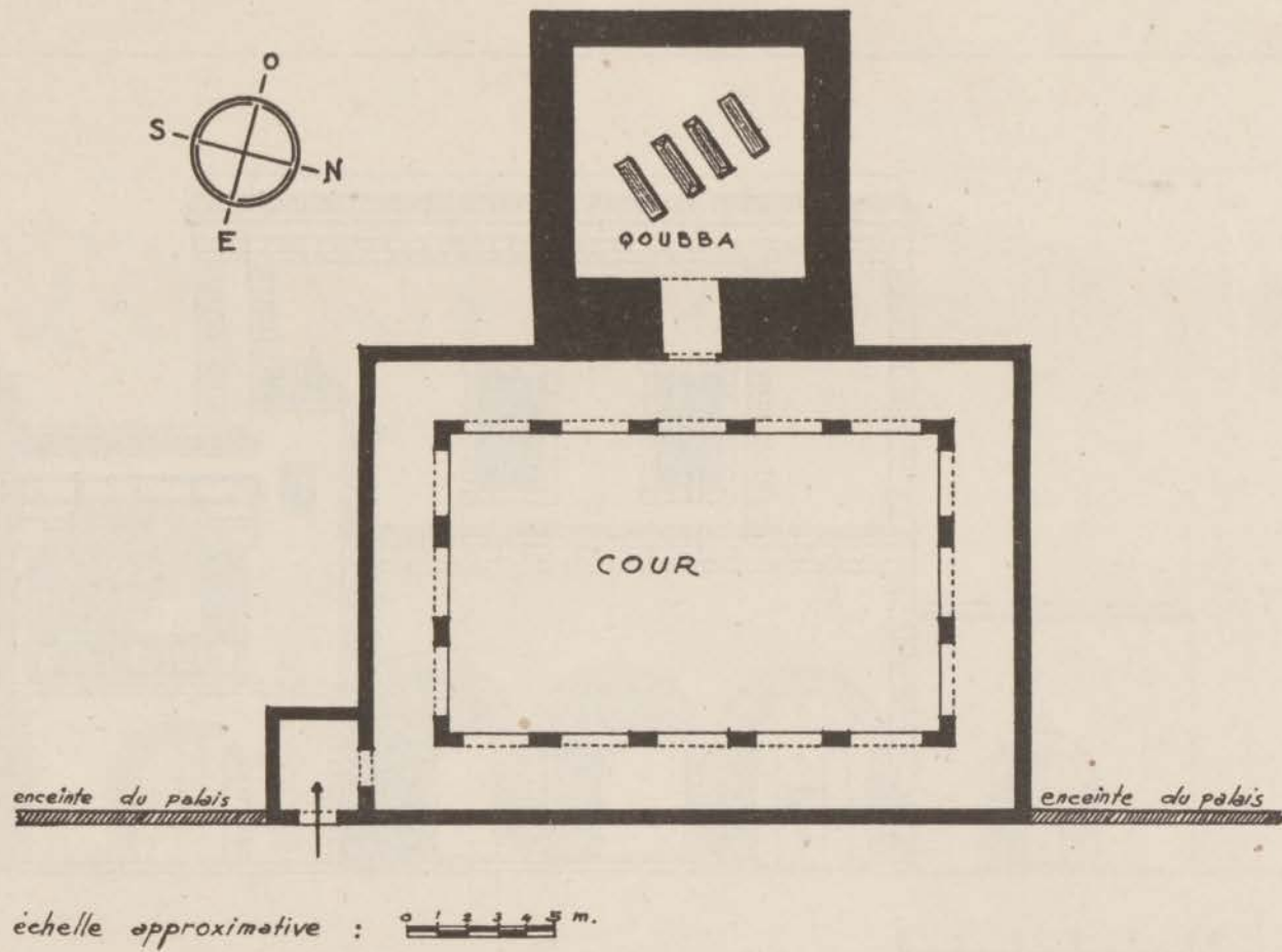
FIG. 171. — Qubba de Sidi Mohammed ben Abdallah et de Moulay Hassan. Plan.
