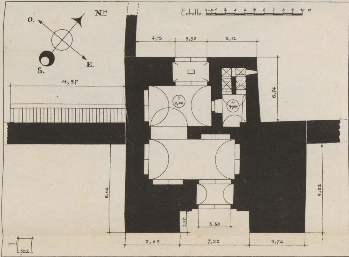
FIG. 52. — Enceinte almohade de la ville de Ribat el-Fath. Porte des Zaer. Plan du rez-de-chaussée.
