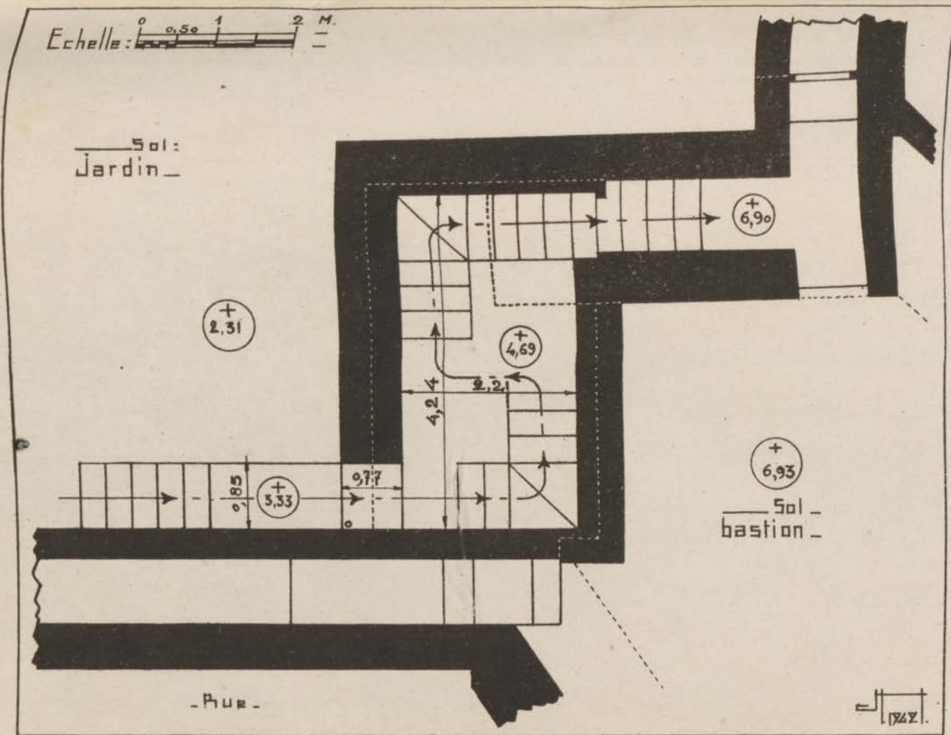
FIG. 104. — Qasba des Oudaia. Enceinte de Moulay er-Rechid. Bastion heptagonal. Plan de l'escalier intérieur d'accès.
