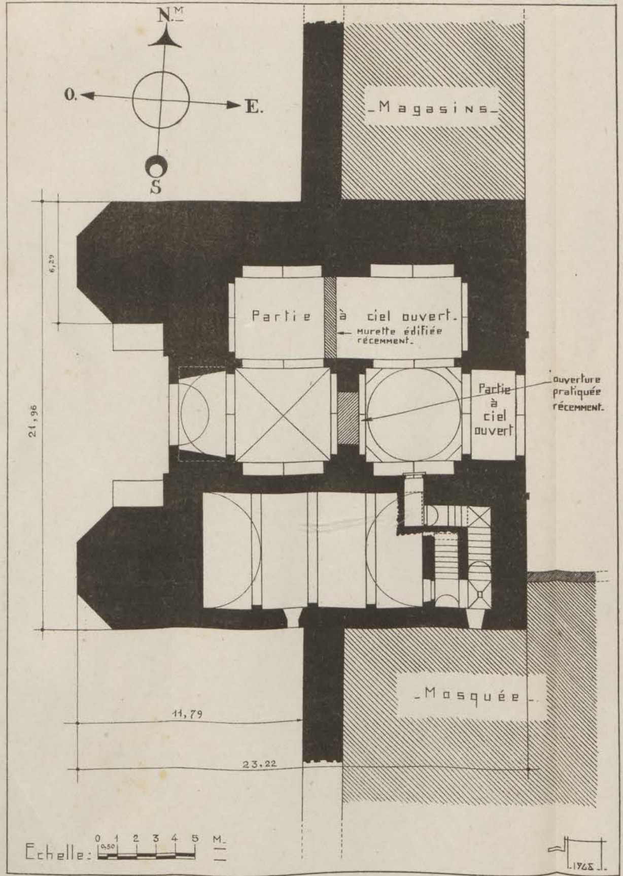
FIG. 35. — Enceinte almohade de la ville de Ribat el-Fath. Bab el-Had. Plan du rez-de-chaussée.
