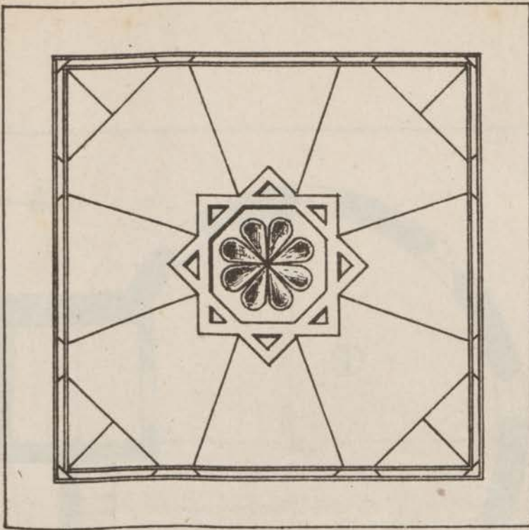
FIG. 93. — Qasba des Oudata. Escalier couvert. Coupole du palier supérieur. Plan.
