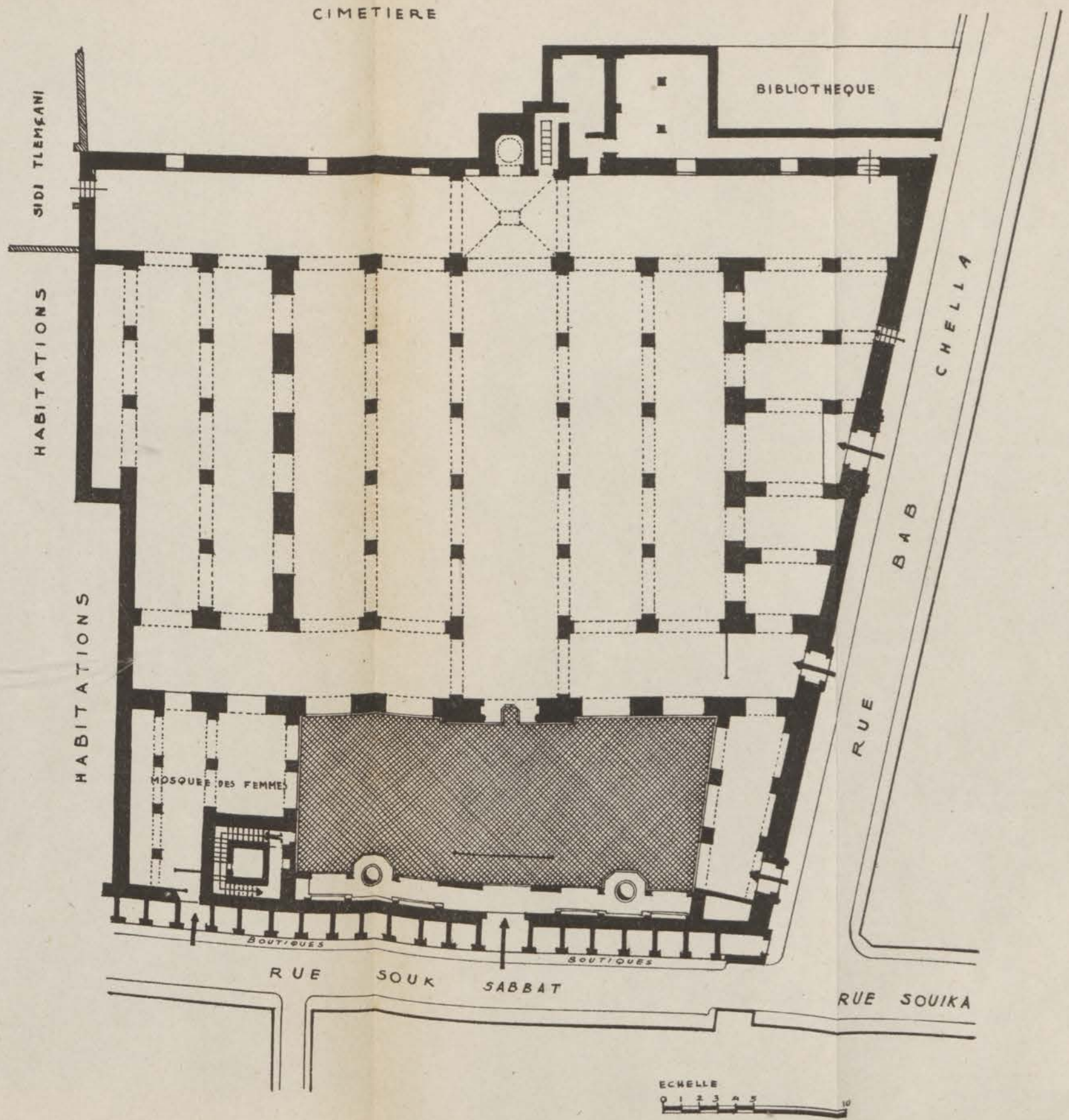
FIG. 64. — Jama el-Kébir. Plan en 1943.
