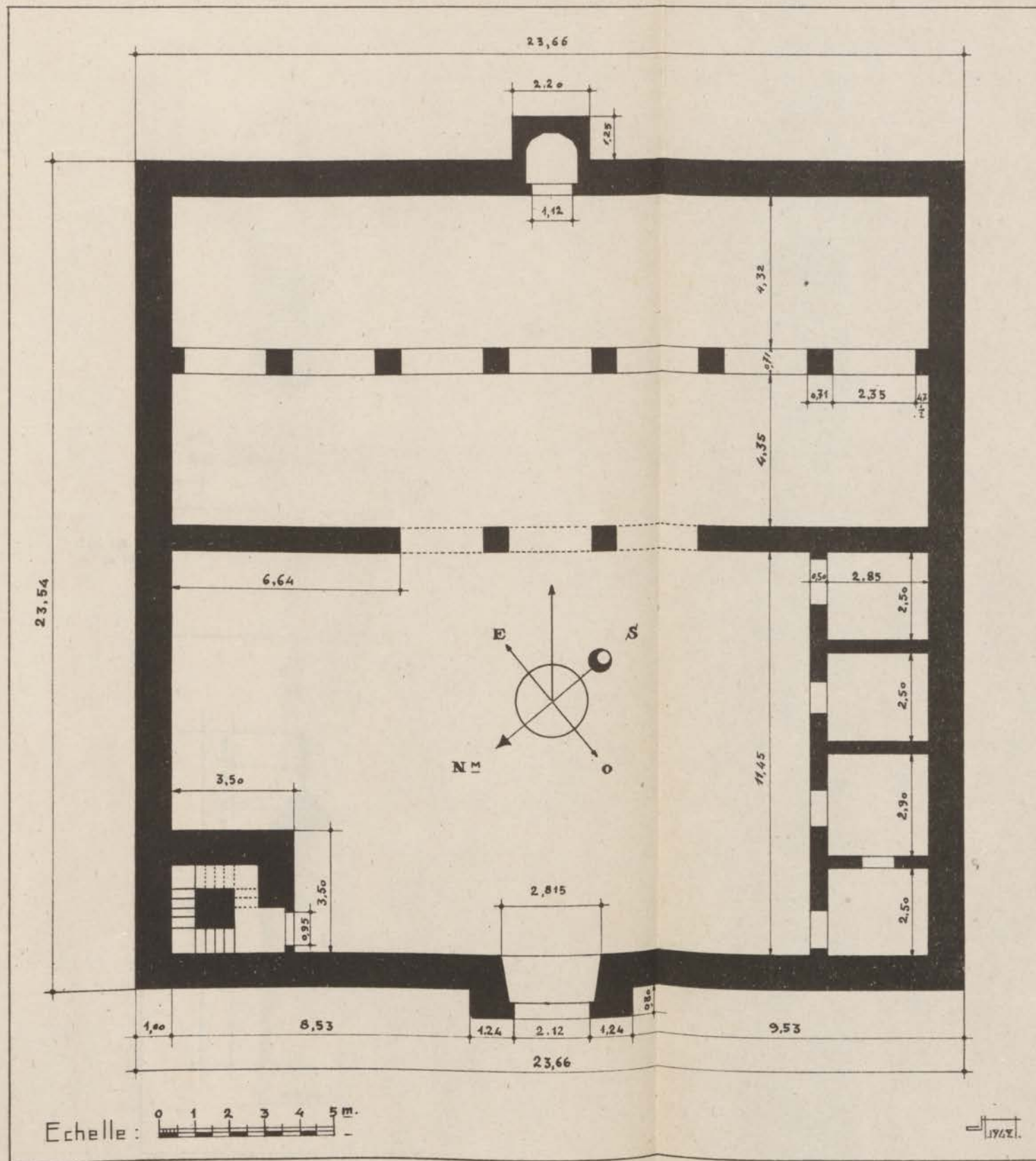
FIG. 145. — Jama Molina. Plan.
