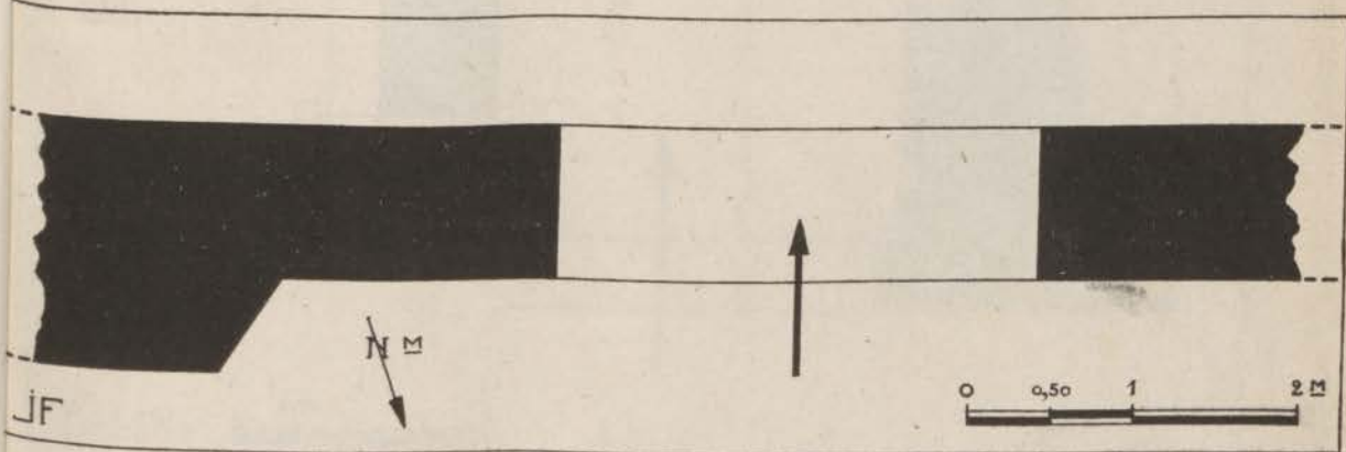
FIG. 129. — Rempart du quai Léon Petit. Bab el-Bhar. Plan.
