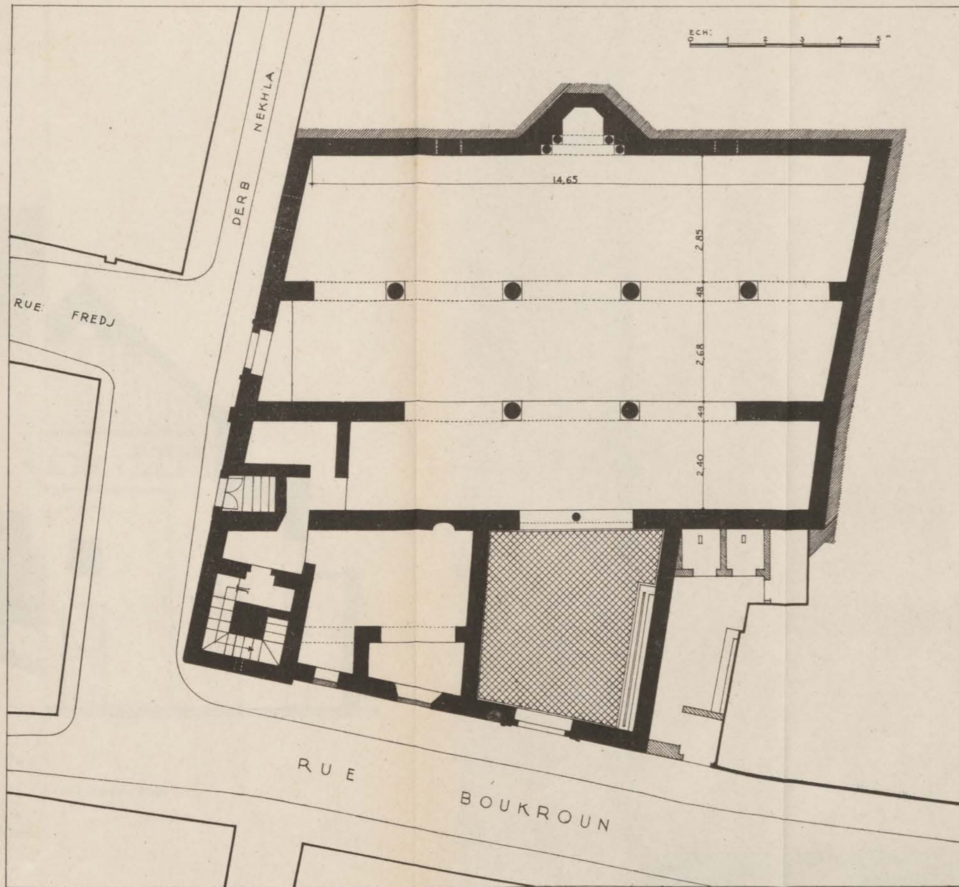
FIG. 163. — Jama en-Nekhla. Plan.
