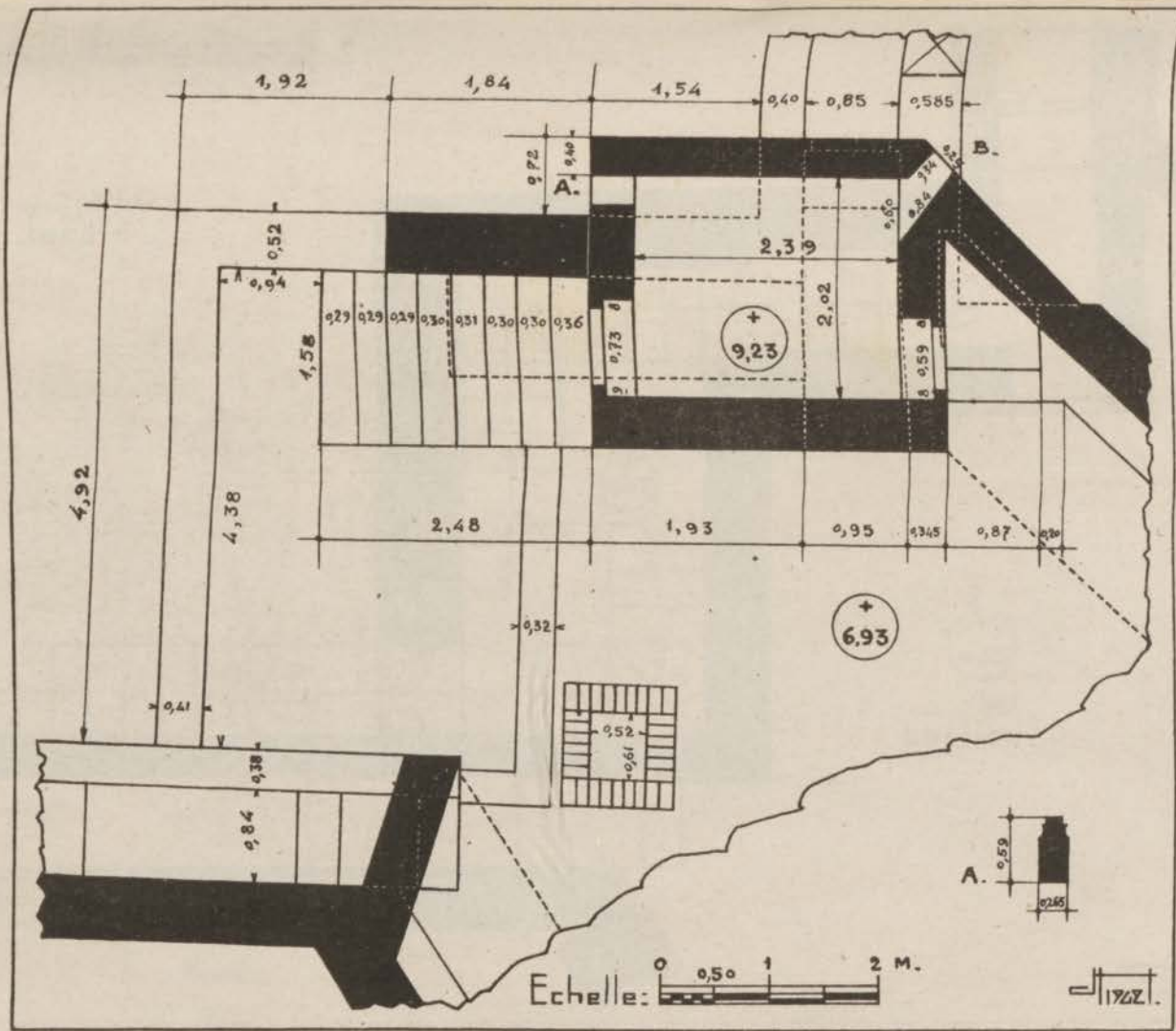
FIG. 103. — Qasba des Oudaïa. Enceinte de Moulay er-Rechid. Bastion heptagonal. Plan partiel de l'étage.
