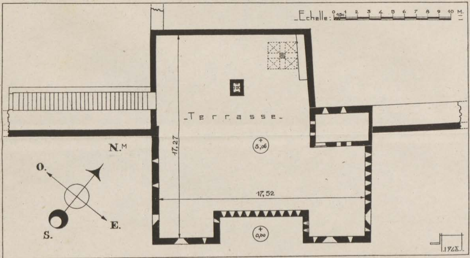
FIG. 53. — Enceinte almohade de la ville de Ribat el-Fath. Porte des Zaer. Plan de la terrasse.
