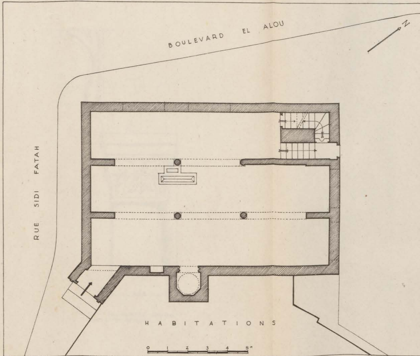
FIG. 166. — Jama Sidi Fatah. Plan.
