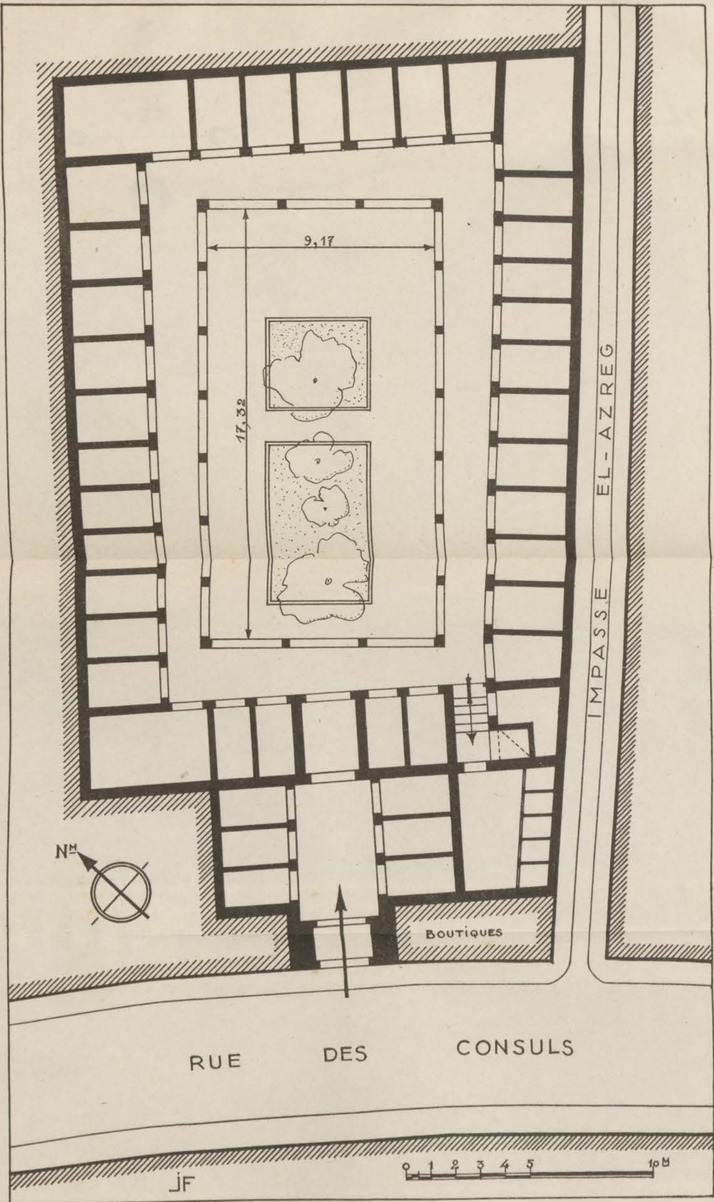
FIG. 184. — Fondouq de Ben Aicha. Plan.
