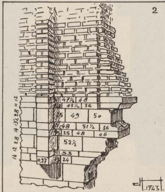
FIG. 10. — Qasba des Oudaïa. Porte du palais d'Abd el-Moumen. Croquis coté de l'appareil.
