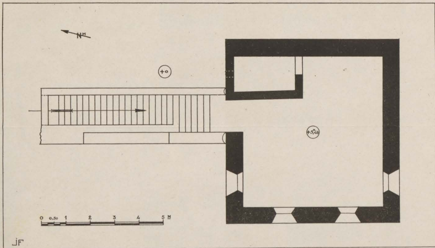
FIG. 127. — Enceinte extérieure alaouite. Bab Marrakech. Plan de la terrasse.
