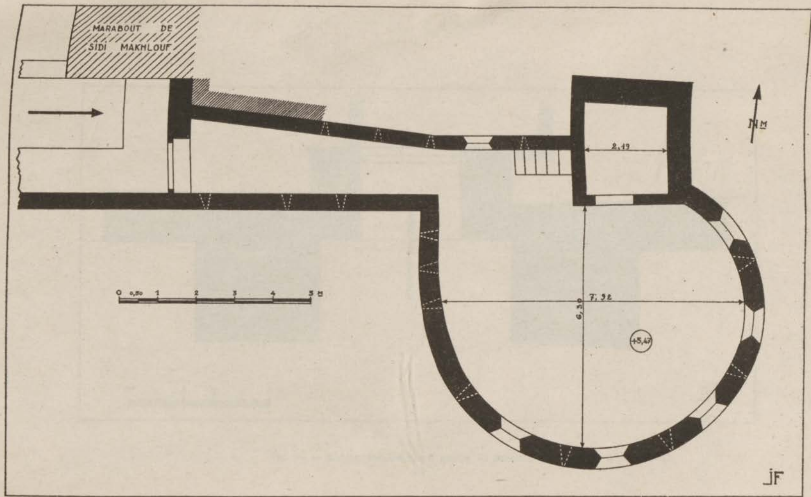
FIG. 95. — Enceinte andalouse de la médina. Barj Sidi Makhlouf. Plan.
