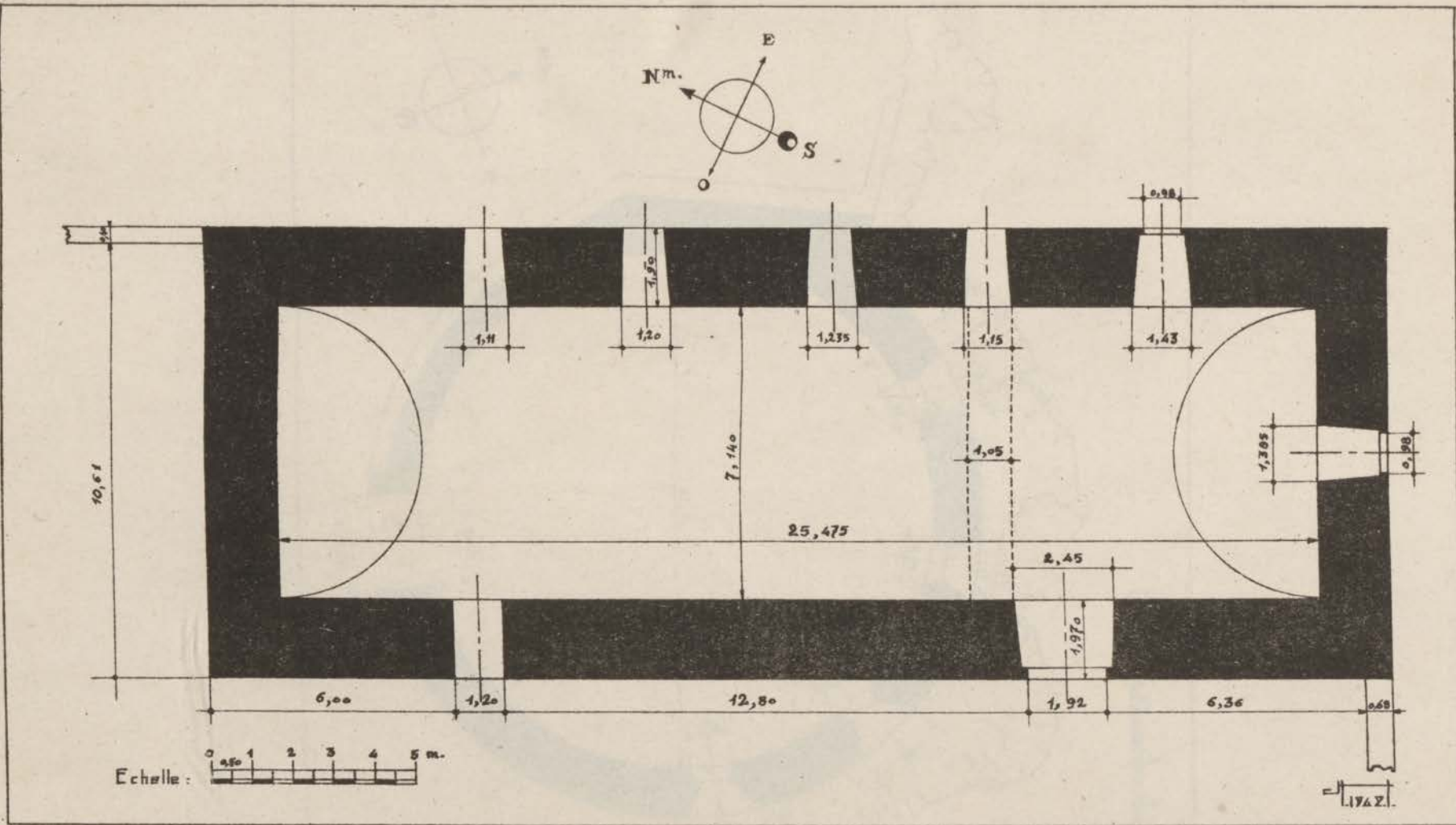
FIG. 112. — Qasba des Oudata. Entrepôt de Moulay el Yazid. Plan.
