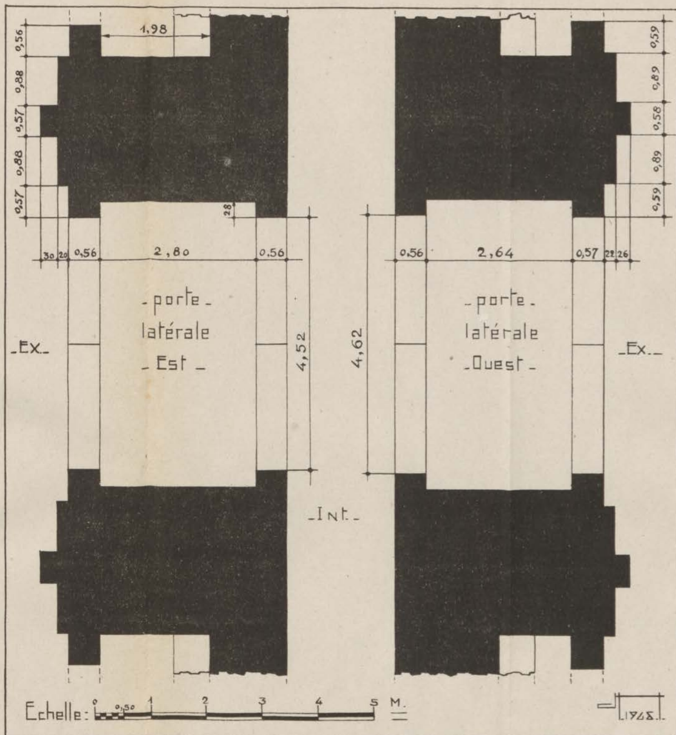
FIG. 60. — Mosquée de Hassan. Plan des portes des faces latérales du sanctuaire.
