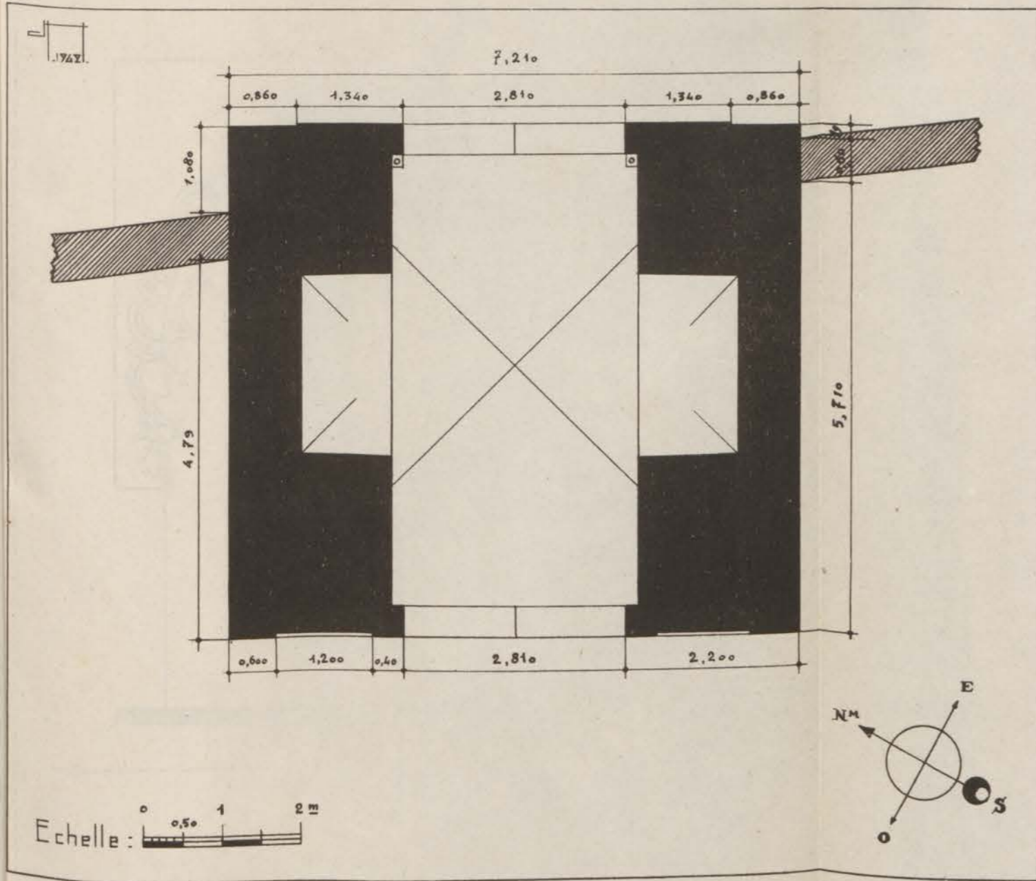
FIG. 130. — Enceinte du méchouar. Bab el-Fouqiya. Plan.
