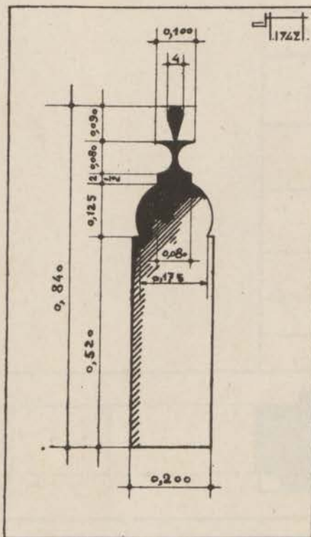
FIG. 149. — Jama Molina. Ouverture de la face sud-est.
