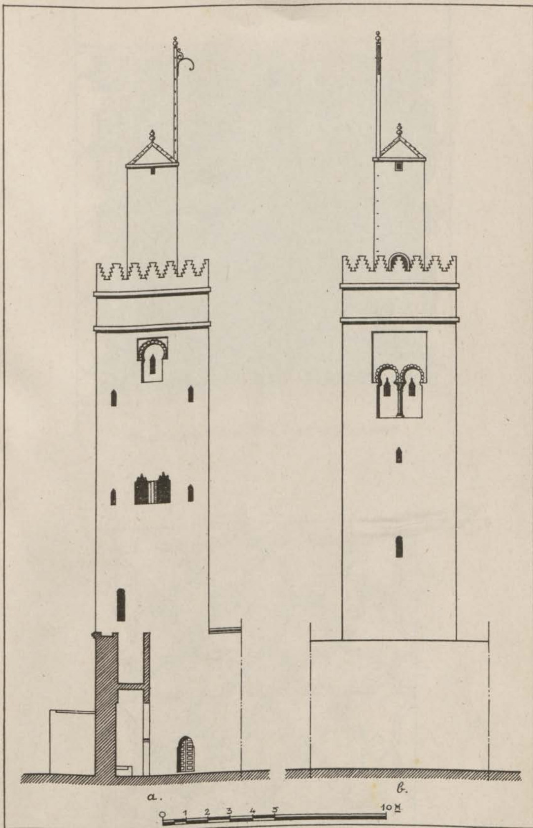
FIG. 68. — Jama el-Kebir. Minaret antérieur à 1939. Faces sud-est et sud-ouest. Elévation.
