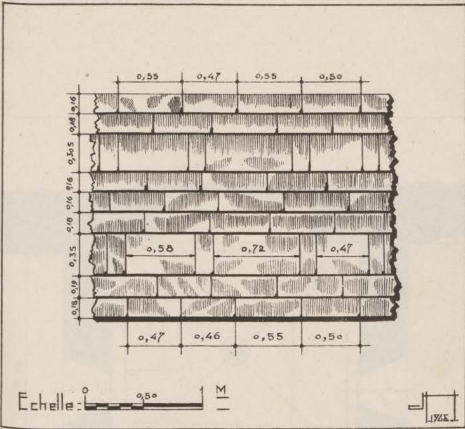
FIG. 80. — Qasba des Oudaïa. Muraille nord-est de l'anse du café maure. Croquis coté de l'appareil.
