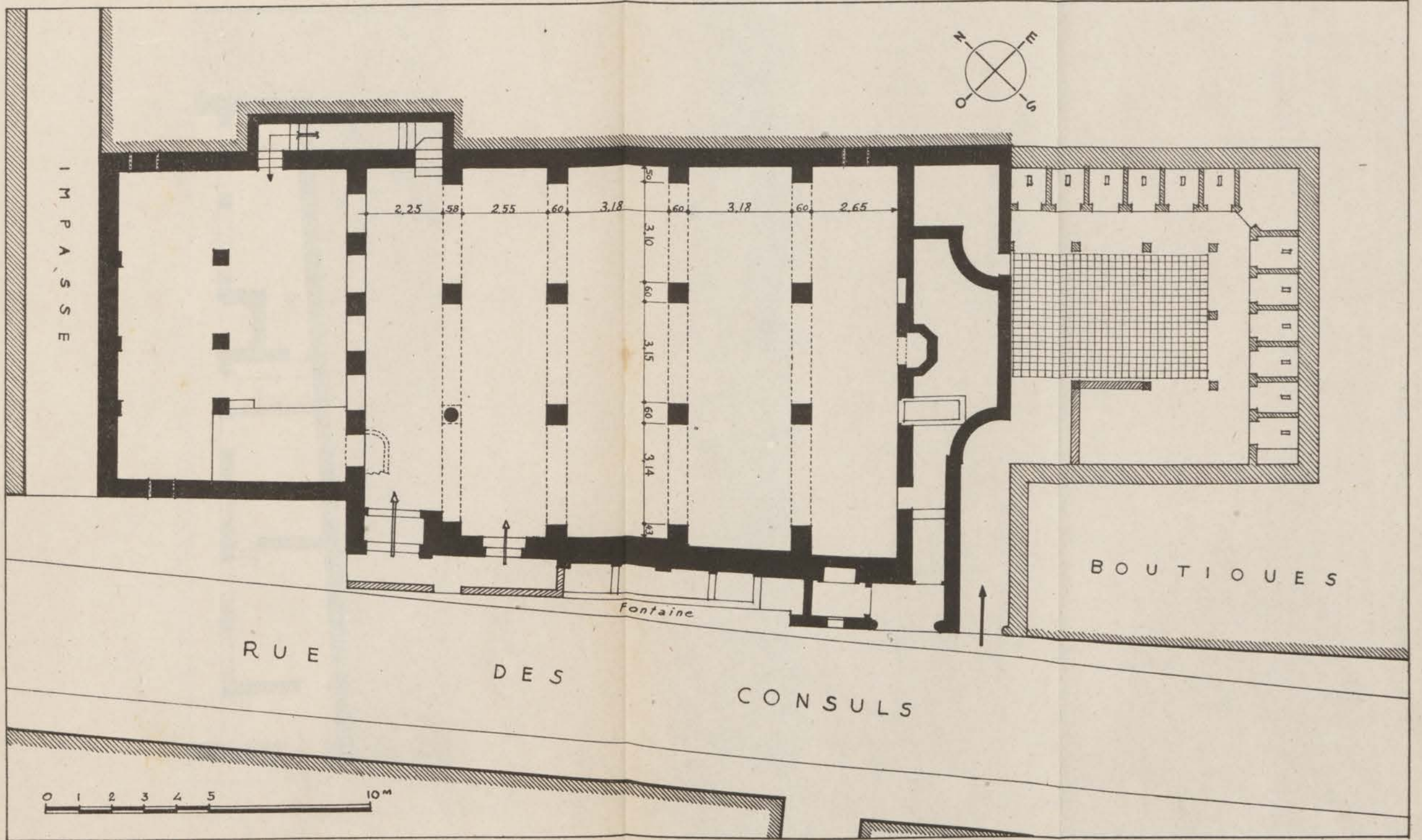
FIG. 158. — Jama el-Guezzarin. Plan.
