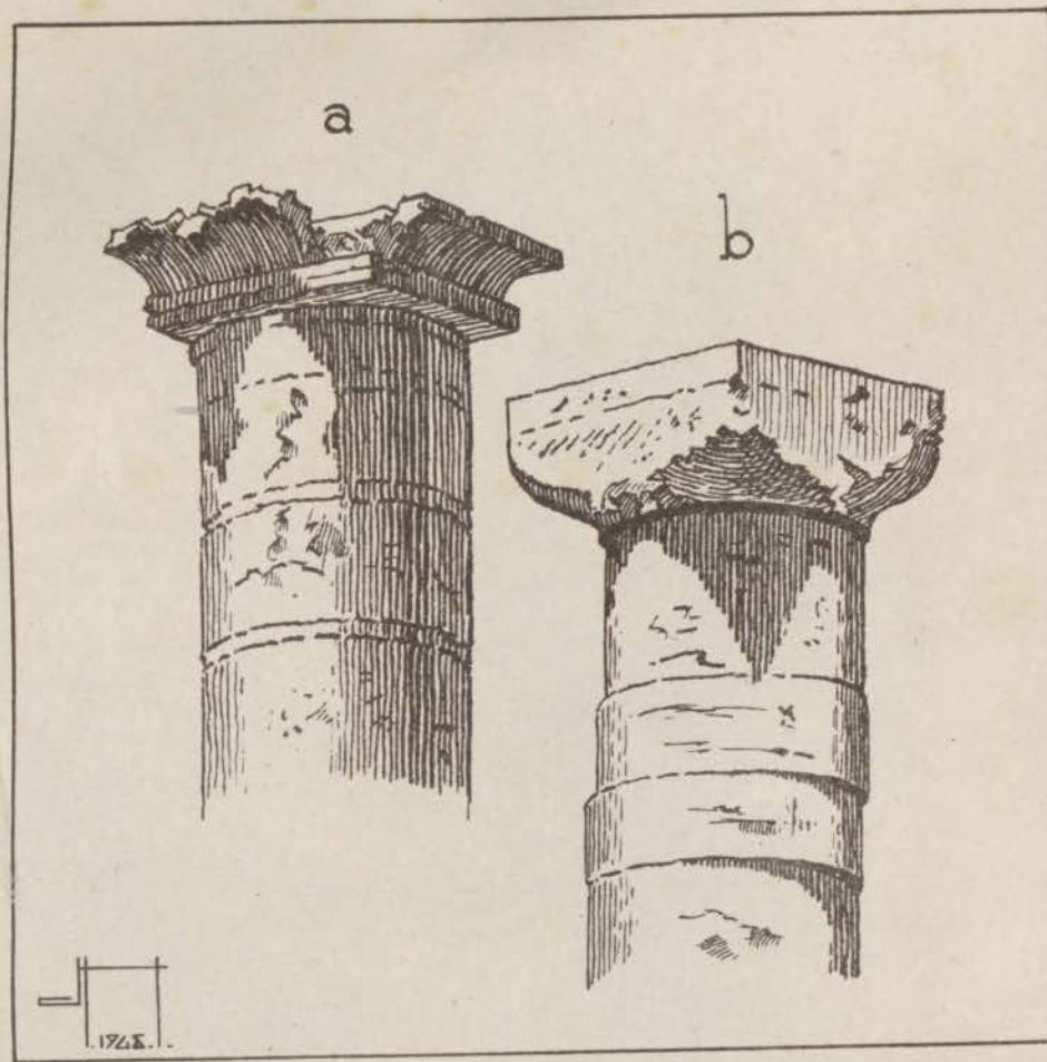
FIG. 57. — Mosquée de Hassan. Chapiteaux de la salle de prières : a, des colonnes du double portique de la qibla ; b, des autres colonnes.
