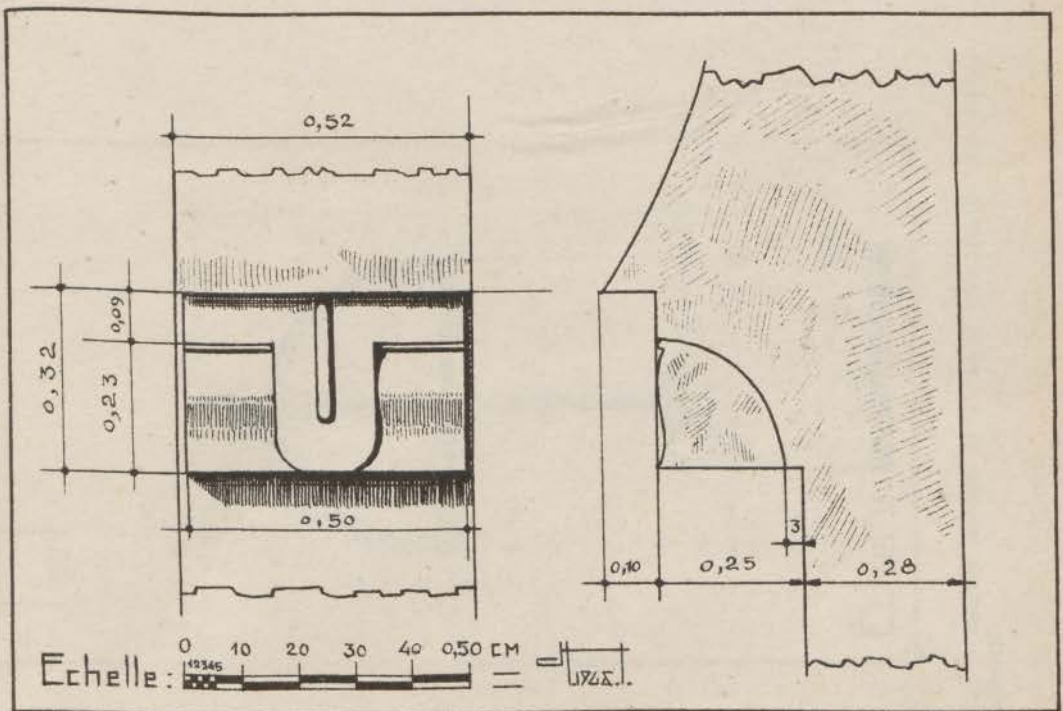
FIG. 40. — Enceinte almohade de la ville de Ribat el-Fath. Bab er-Rouah. Surabaque des arcs des vestibules.
