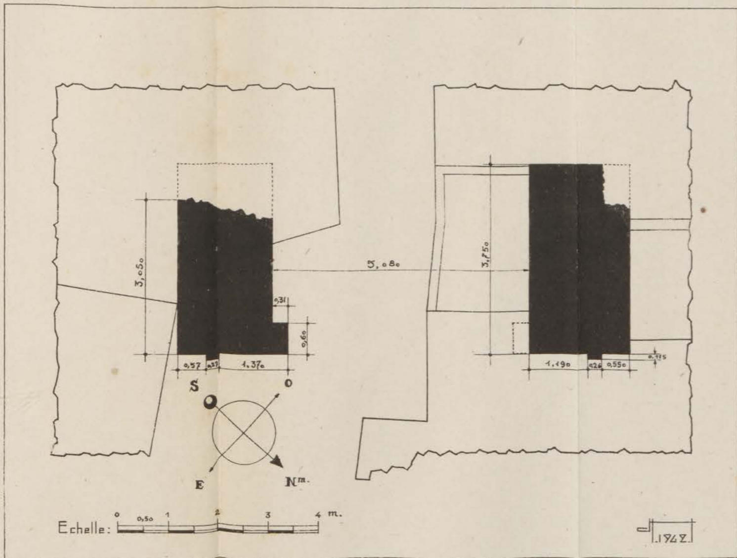
FIG. 27. — Qasba des Oudata. Porte du palais d'Abd el-Moumen. Plan.
