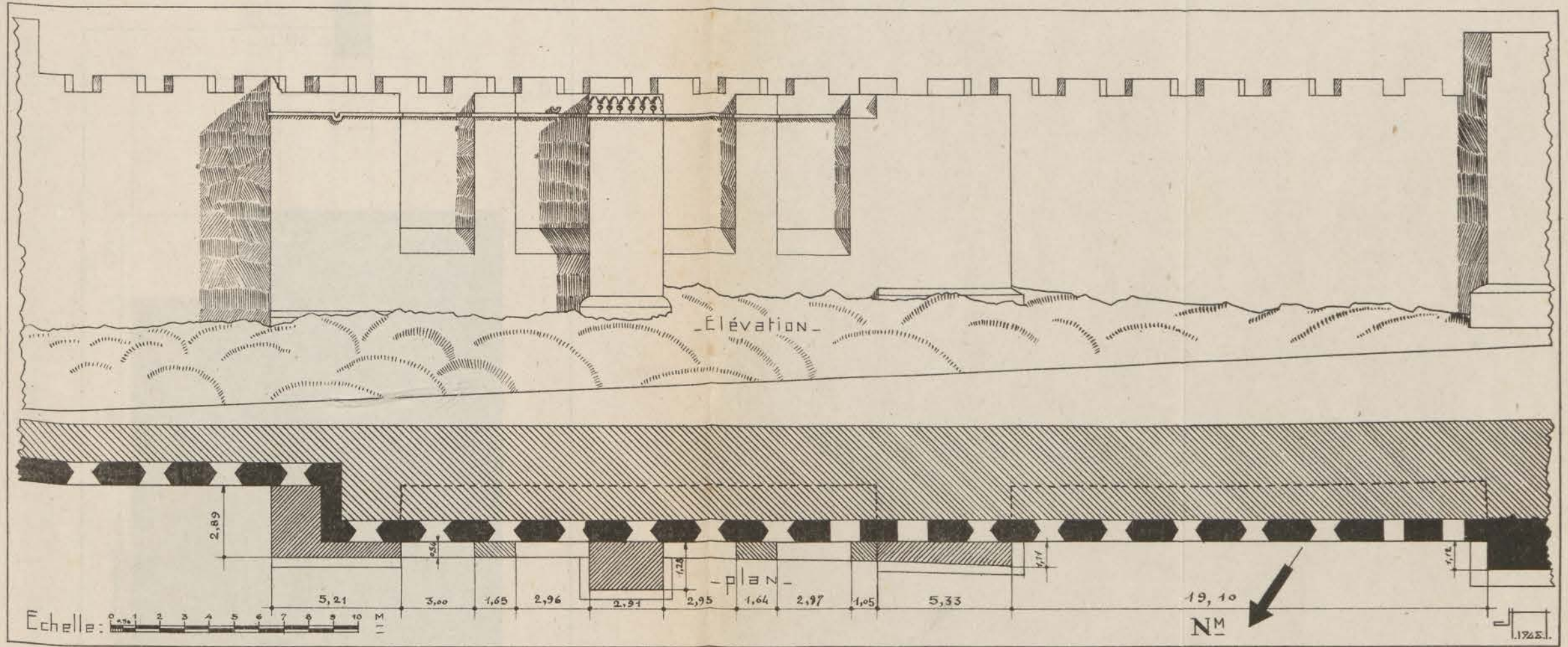
FIG. 3. — Qasba des Oudala. Encinte almohade, face nord-ouest. Elévation et plan de la partie centrale.
