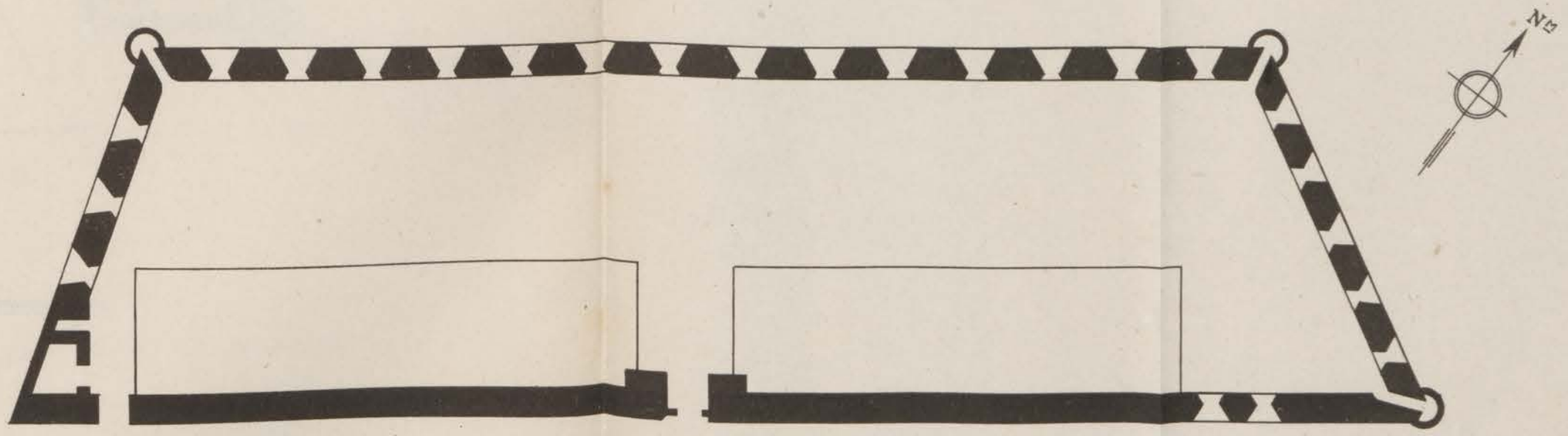
FIG. 121. — La sqala. Plan.
