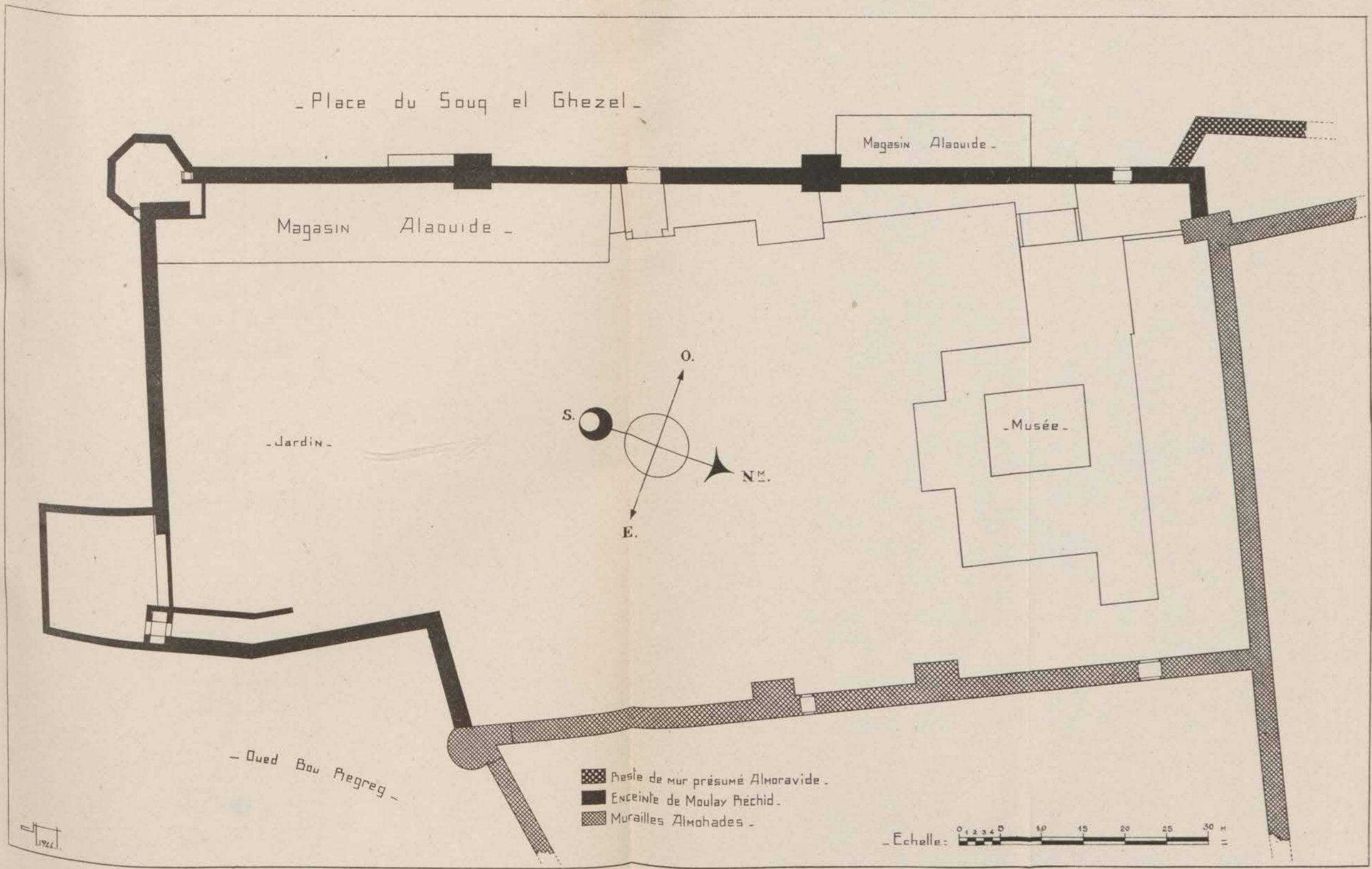
FIG. 97. — Qasba des Oudala. Enceinte de Moulay er-Rechid. Plan d'ensemble.
