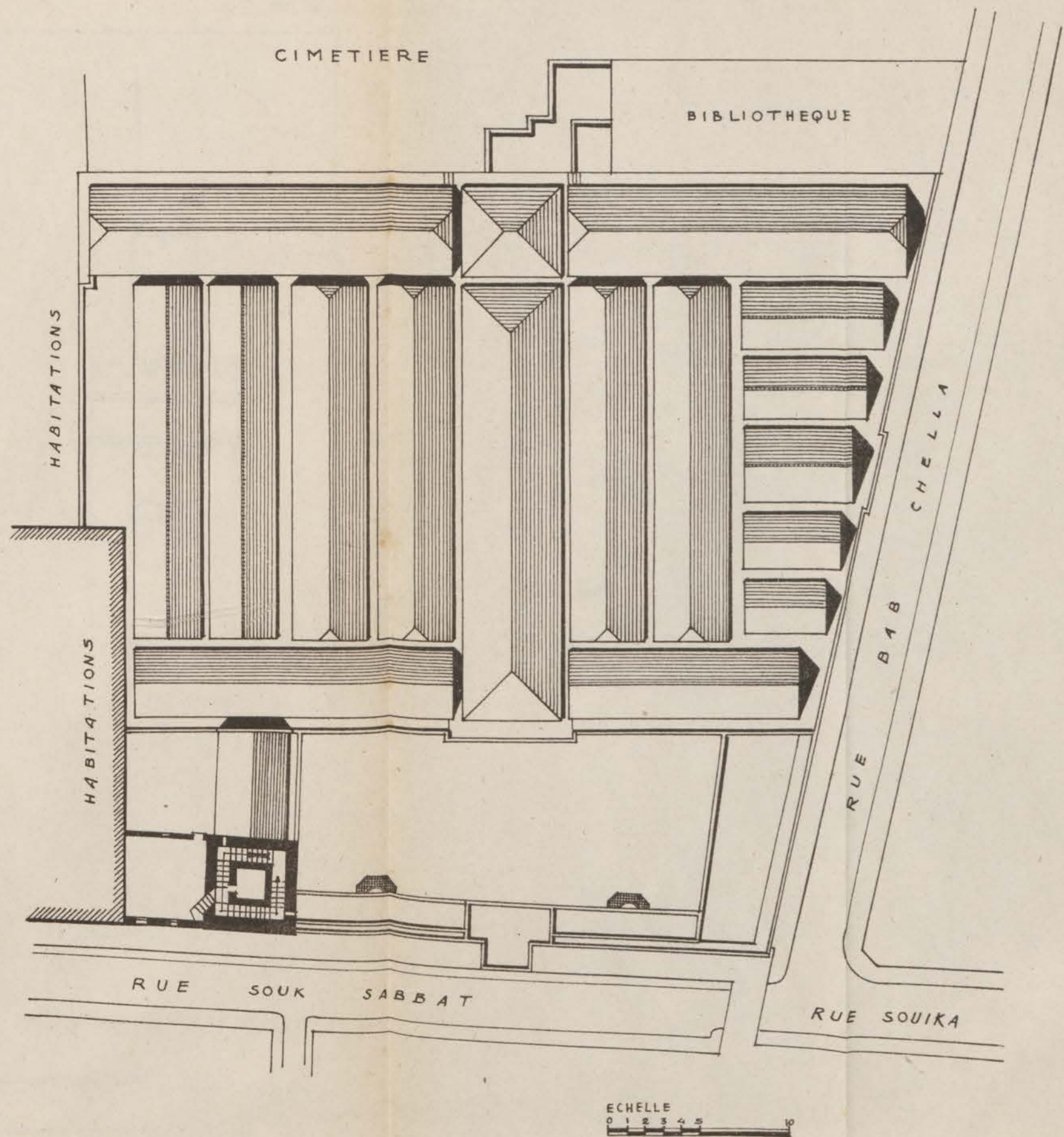
FIG. 67. — Jama el-Kebir. Plan des toitures.
