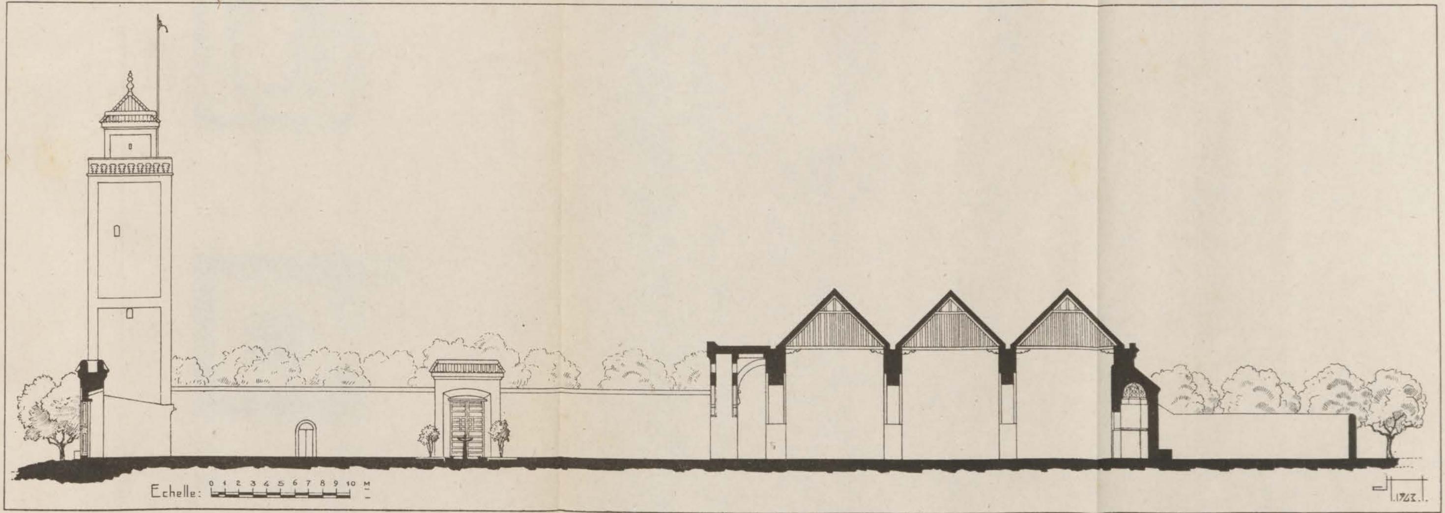
FIG. 136. — Jama es-Sounna. Coupe longitudinale.
