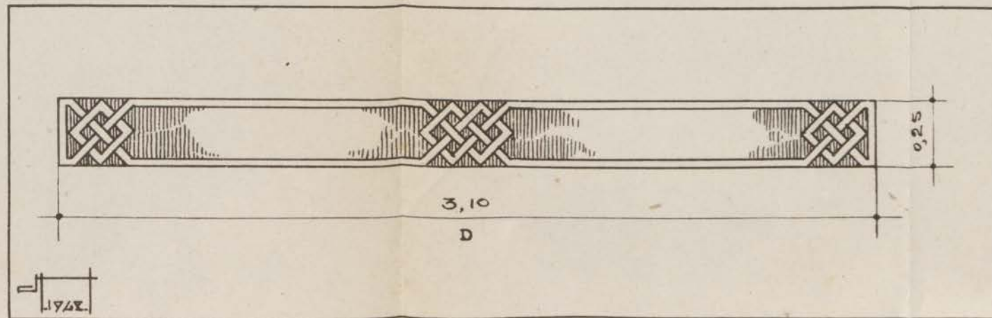
FIG. 88. — Qasba des Oudaia. Escalier des Pirates. Décor de la voûte en arc de cloître, au-dessus de la partie droite du départ.
