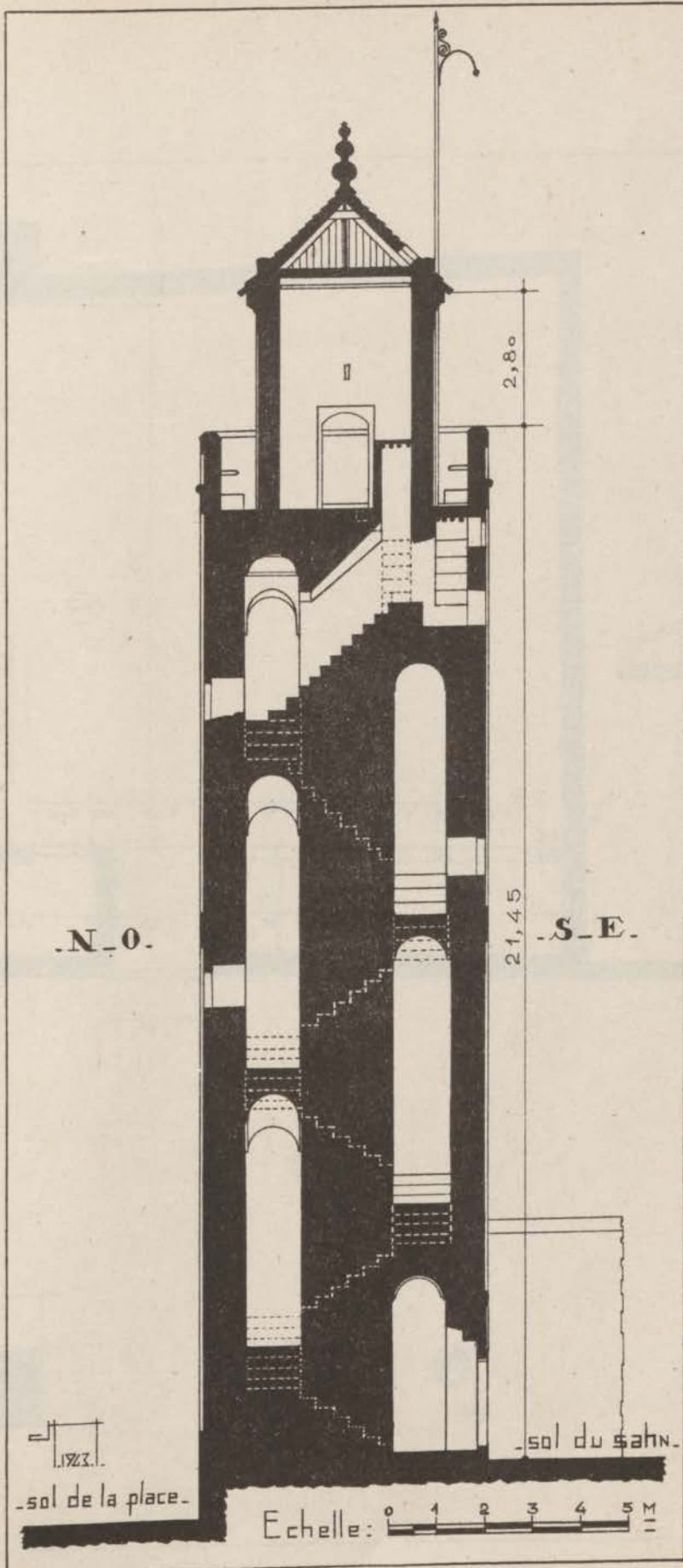
FIG. 138. — Jama es-Sounna. Minaret. Coupe.
