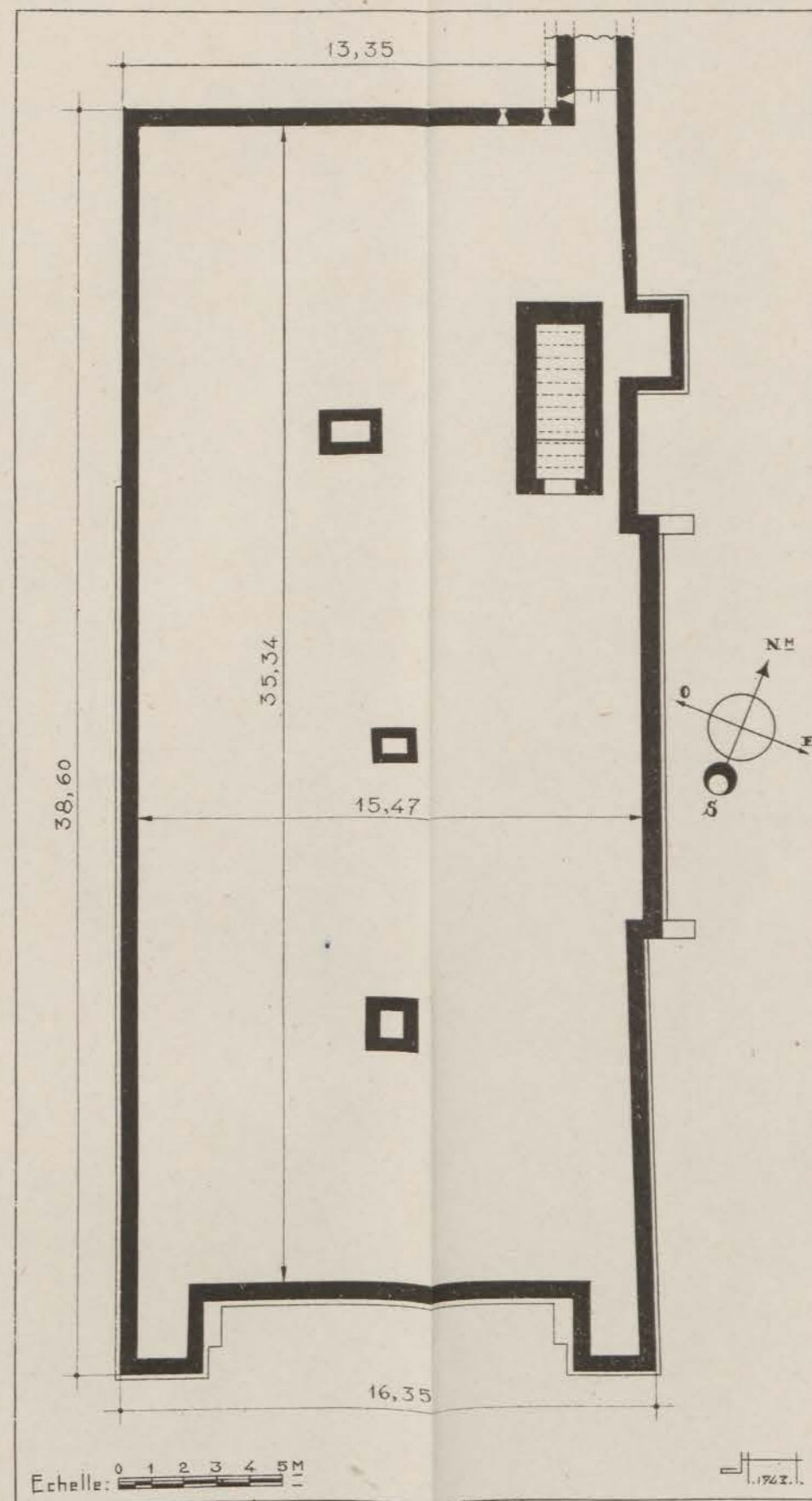
FIG. 14. — Qasba des Oudaïa. Grande porte. Plan de la terrasse.
