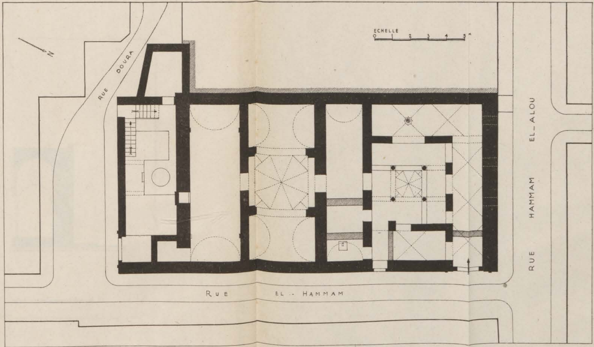
FIG. 75. — Hammam el-Jdid. Plan.
