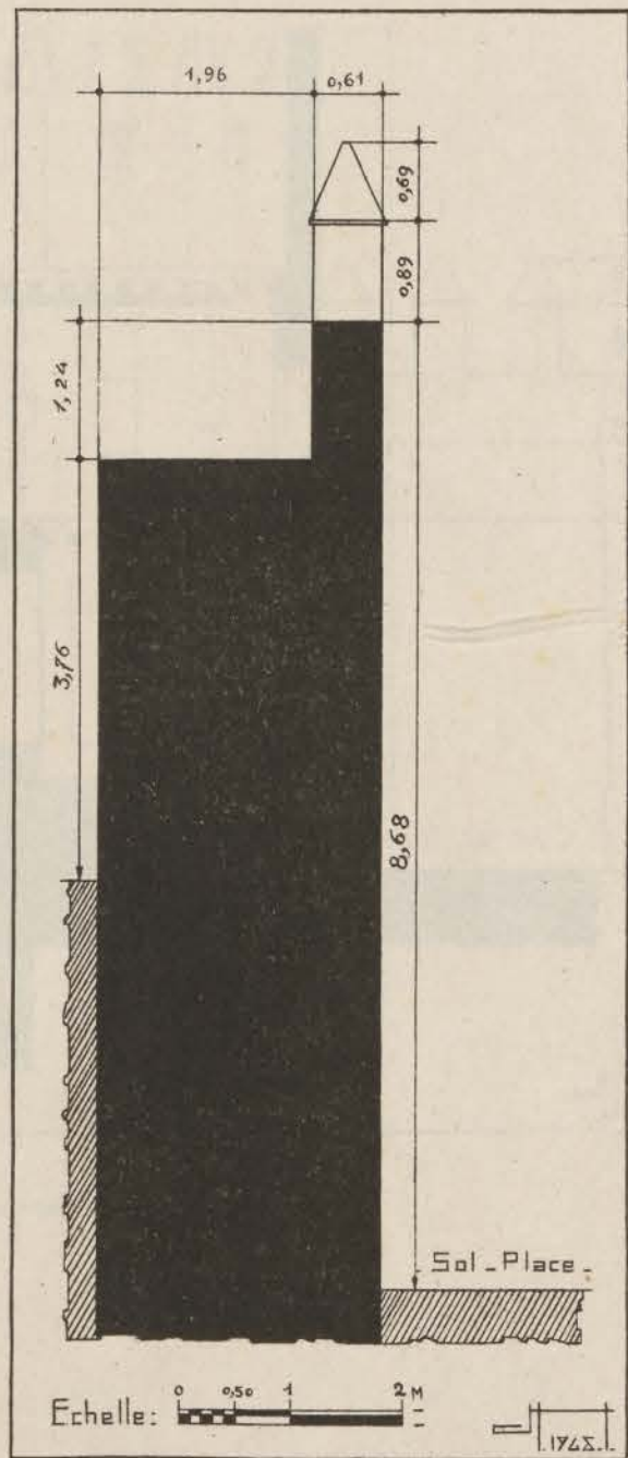
FIG. 4. — Qasba des Oudaya. Enceinte almohade. Coupe, place du Souq el-Ghezal.
