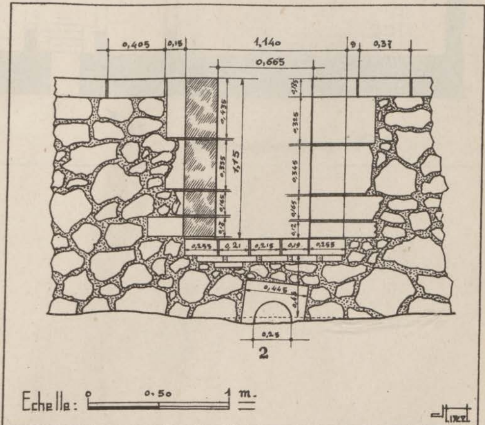
FIG. 115. — Qasba des Oudaïa. Borj circulaire. Détail de la bâtisse.
