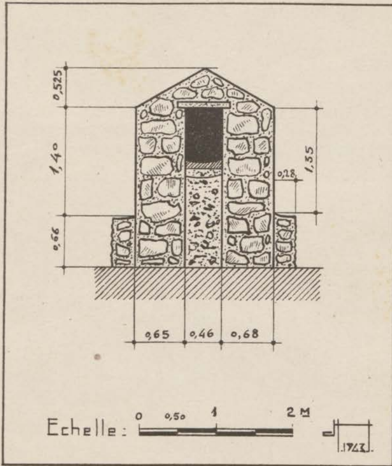
FIG. 181. — Aqueduc de l'Ain Ahig. Coupe.
