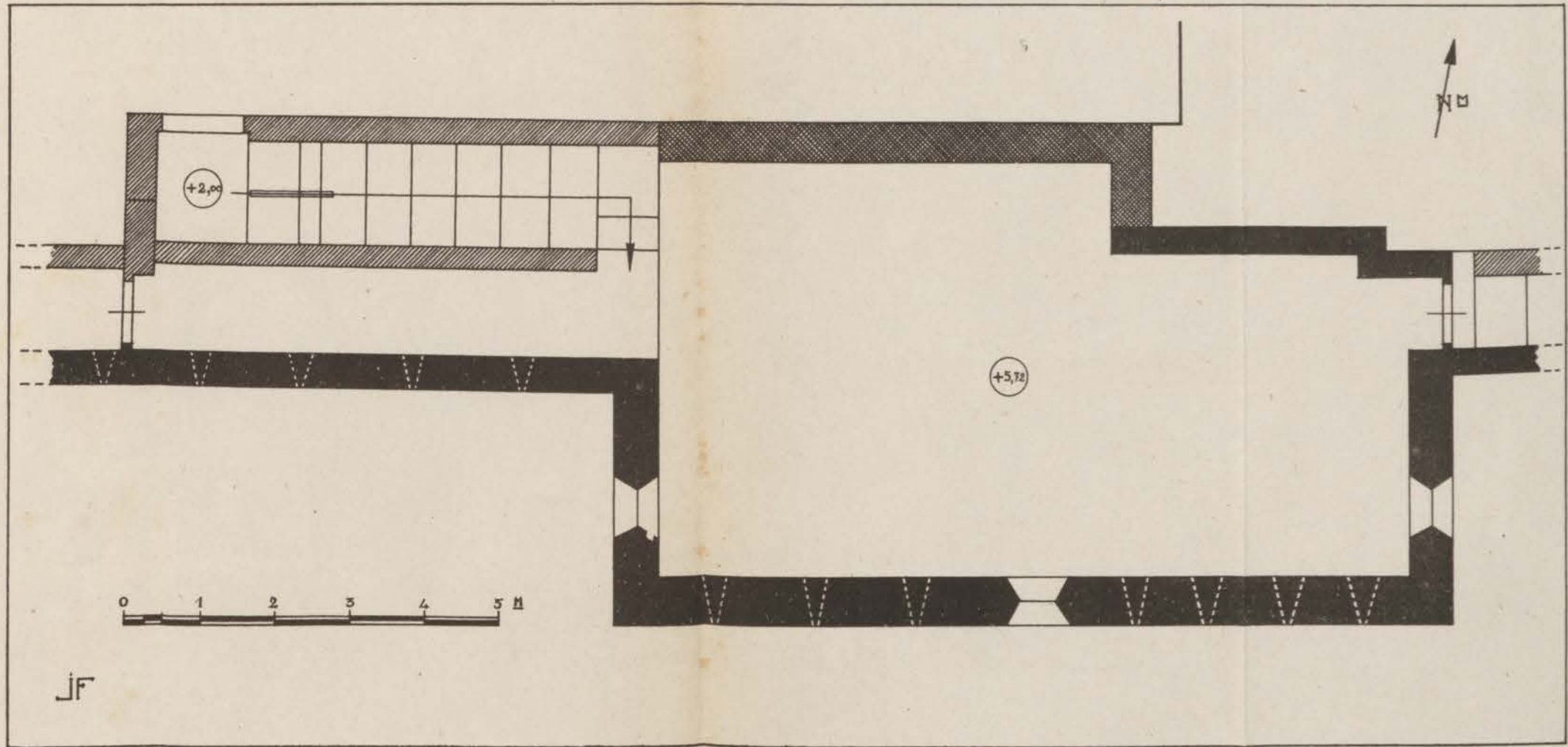
FIG. 134. -- Bab Chella, porte alaouite de l'enceinte andalouse de la médina. Plan de la terrasse.
