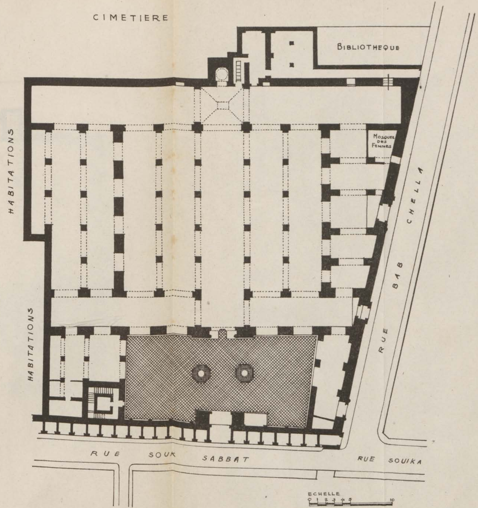
Fig. 71. — Jama el-Kebir. Plan en 1937.
