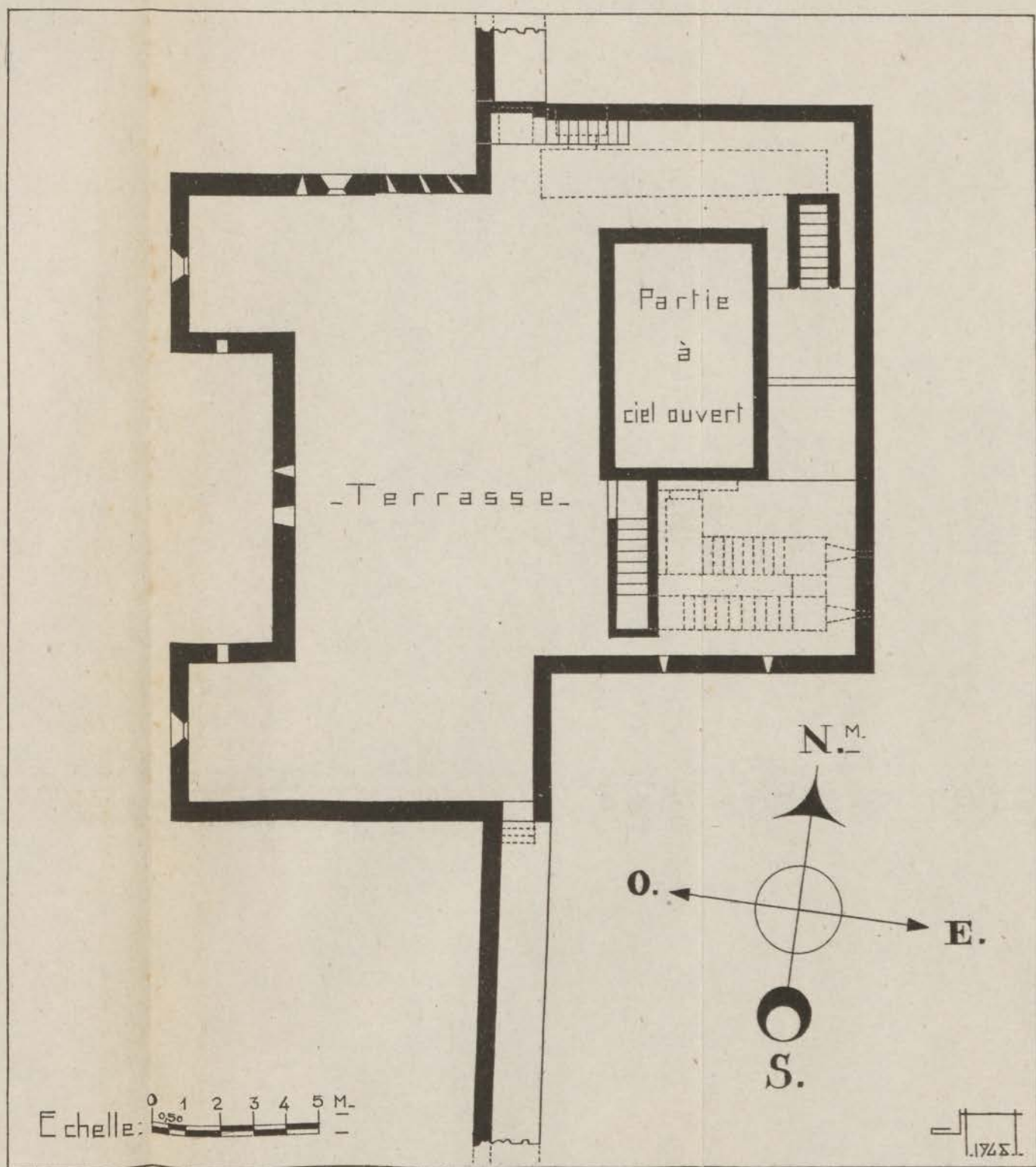
FIG. 34. — Enceinte almohade de la ville de Ribat el-Fath. Bab el-Alou. Plan de la terrasse.
