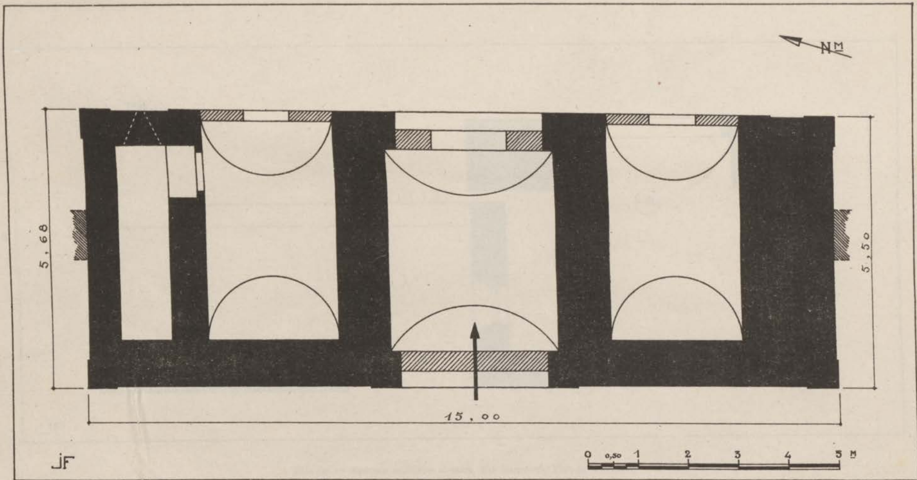
FIG. 125. — Enceinte extérieure alaouite. Bab Qebibat. Plan.
