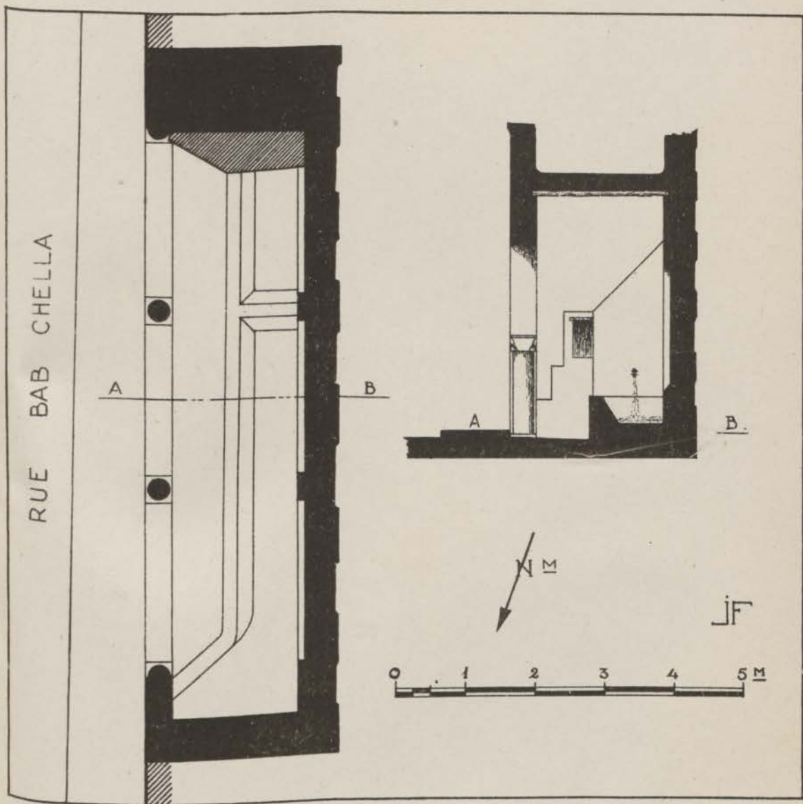
FIG. 73. — Fontaine mérinite, rue Bab Chella. Plan et coupe.
