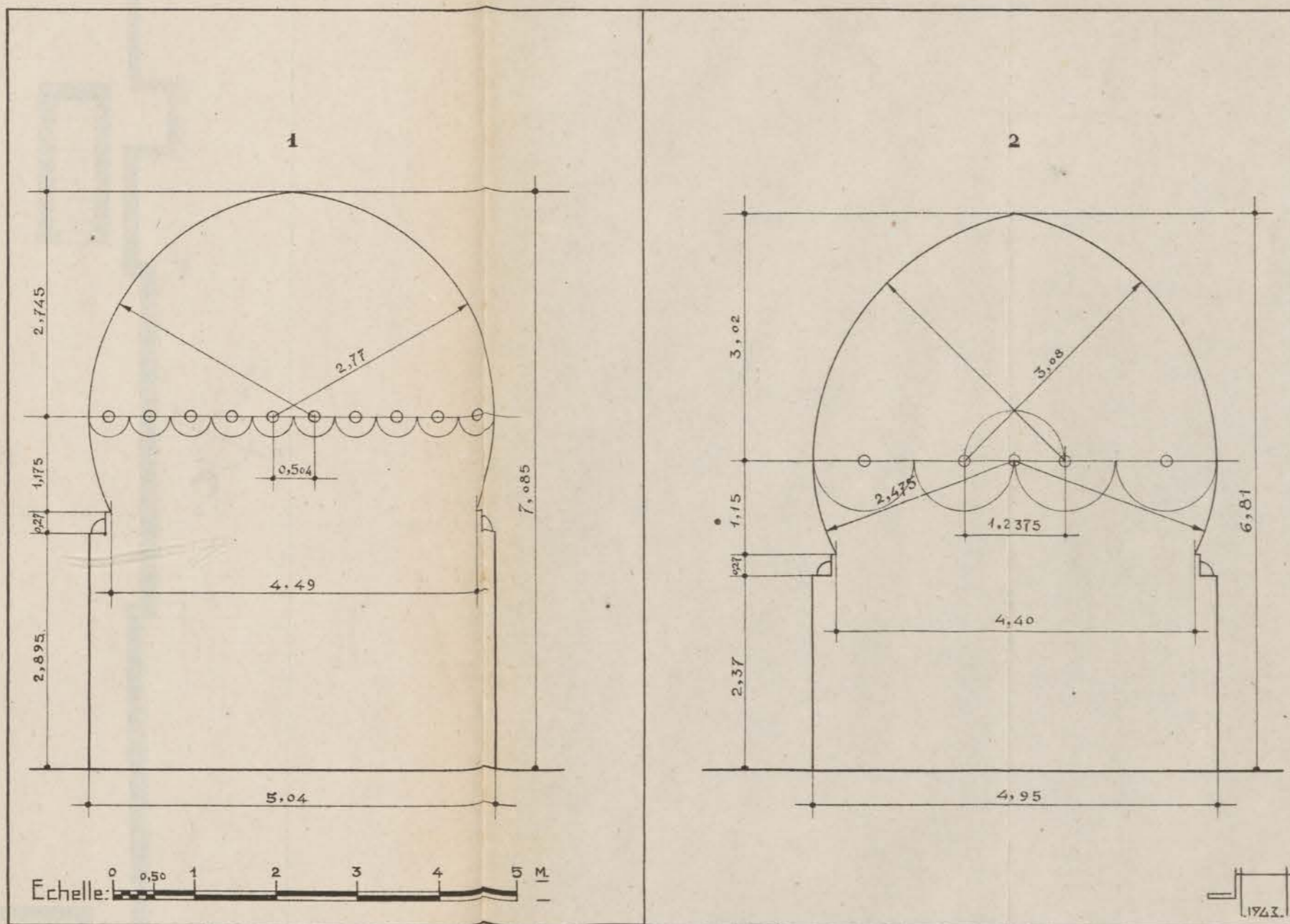
FIG. 12. — Qasba des Oudala. Grande porte. Formule des arcs des baies d'accès. 1, face extérieure ; 2, face intérieure.
