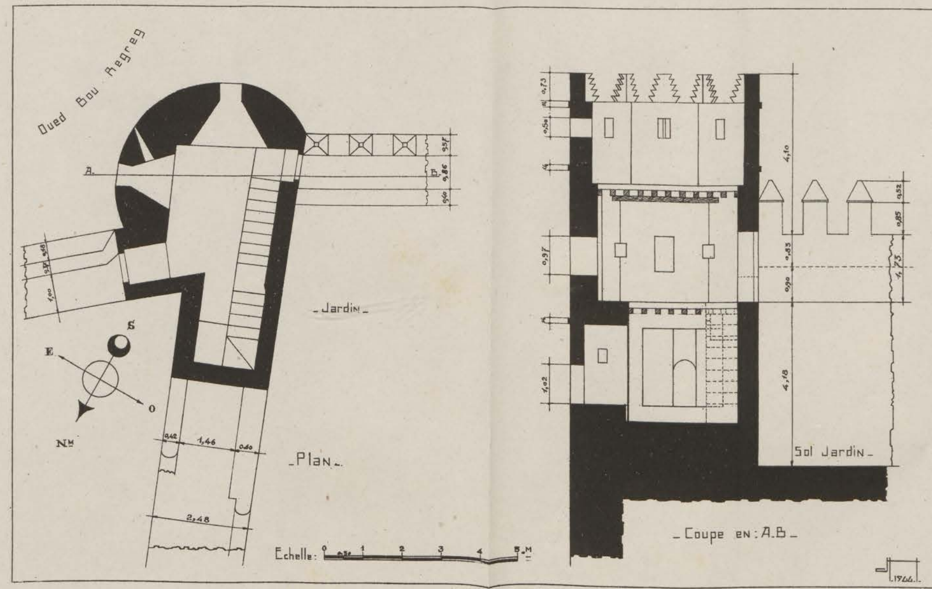
FIG. 7. — Qasba des Oudaia. Enceinte almohade. Tour de l'Est. Plan et coupe.
