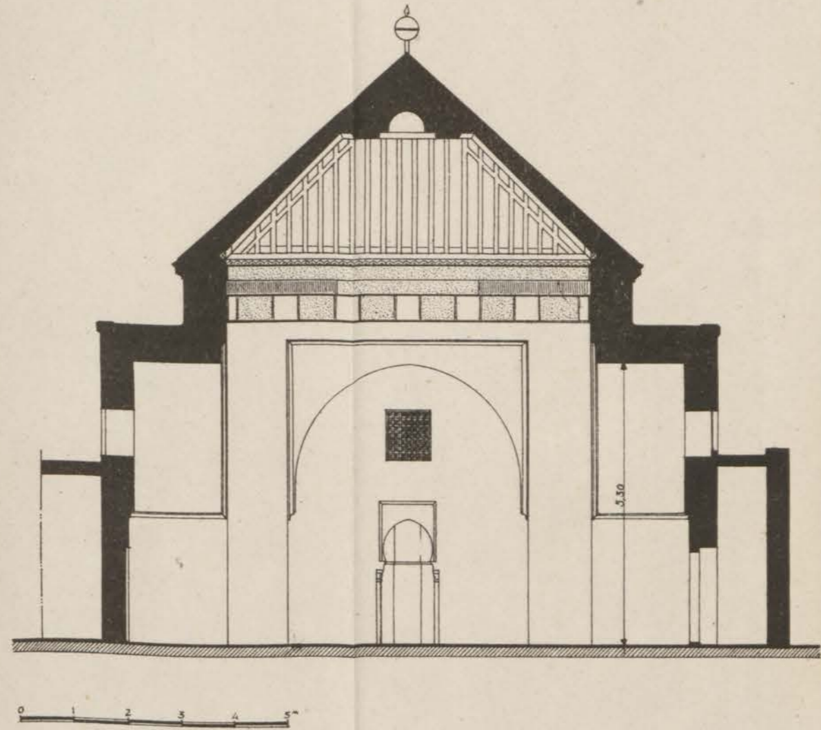
FIG. 165. — Jama el-Qoubba. Coupe.
