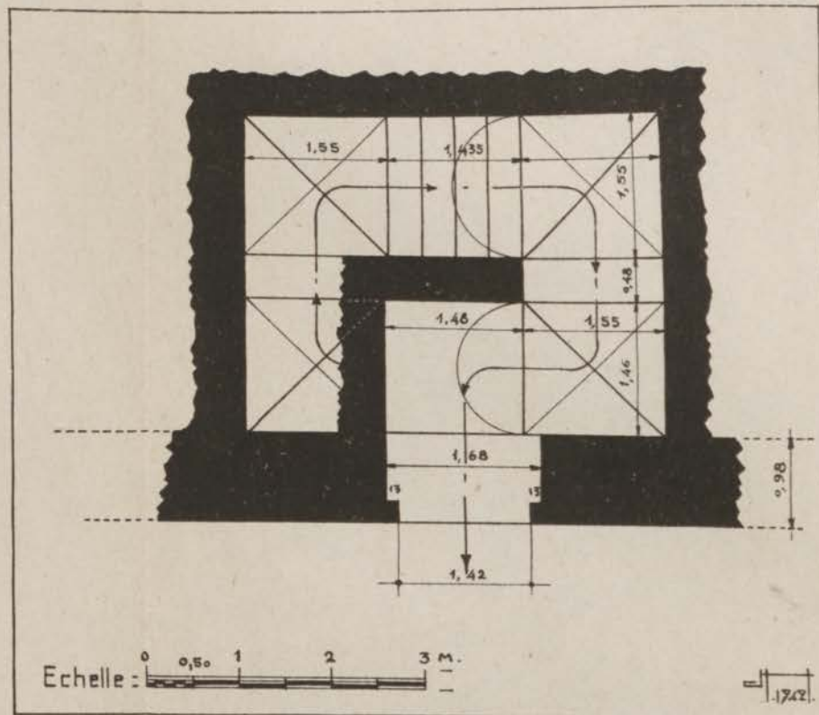
Fig. 86. — Qasba des Oudaia. Escalier des Pirates. Plan de la partie inférieure et de l'arrivée sur l'oued.
