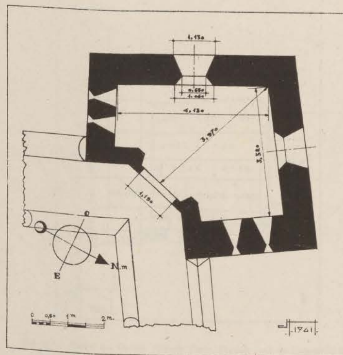
FIG. 6. — Qasba des Oudaia. Enceinte almohade. Tour d'angle ouest. Plan.
