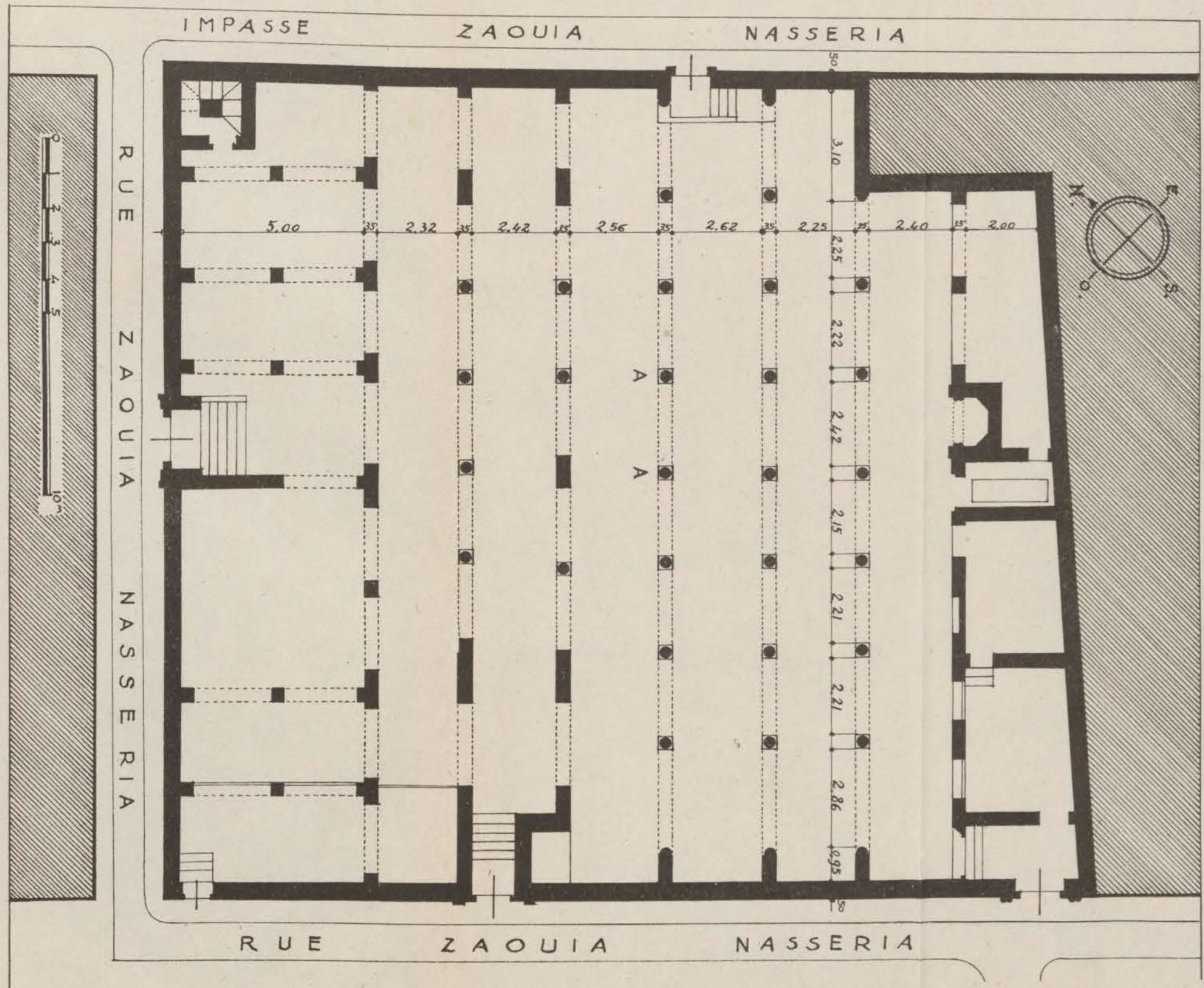
Fig. 159. — Jama Naçiriya. Plan.
