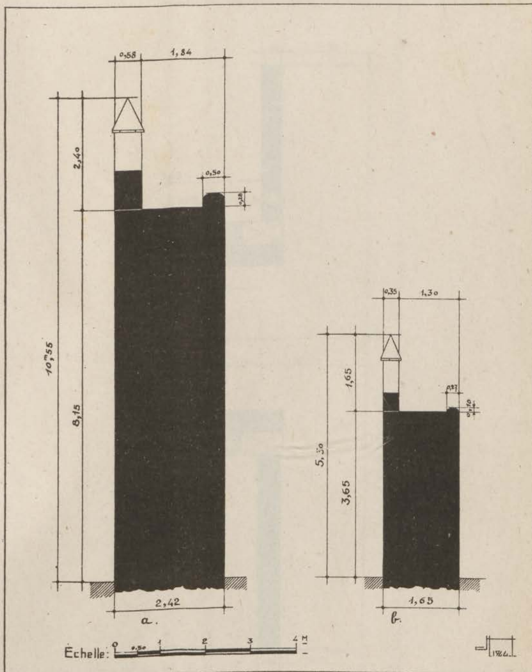
FIG. 31. — Enceintes de Rabat. Coupe : a, enceinte almohade de la ville de Ribat el-Fath ; b, enceinte andalouse de la médina, boulevards Joffre et Galliéni.
