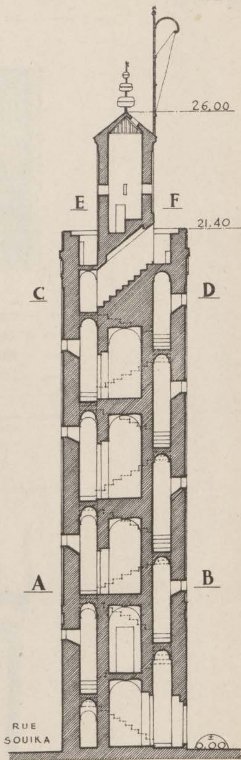
COUPE SUIVANT 1 - 2
