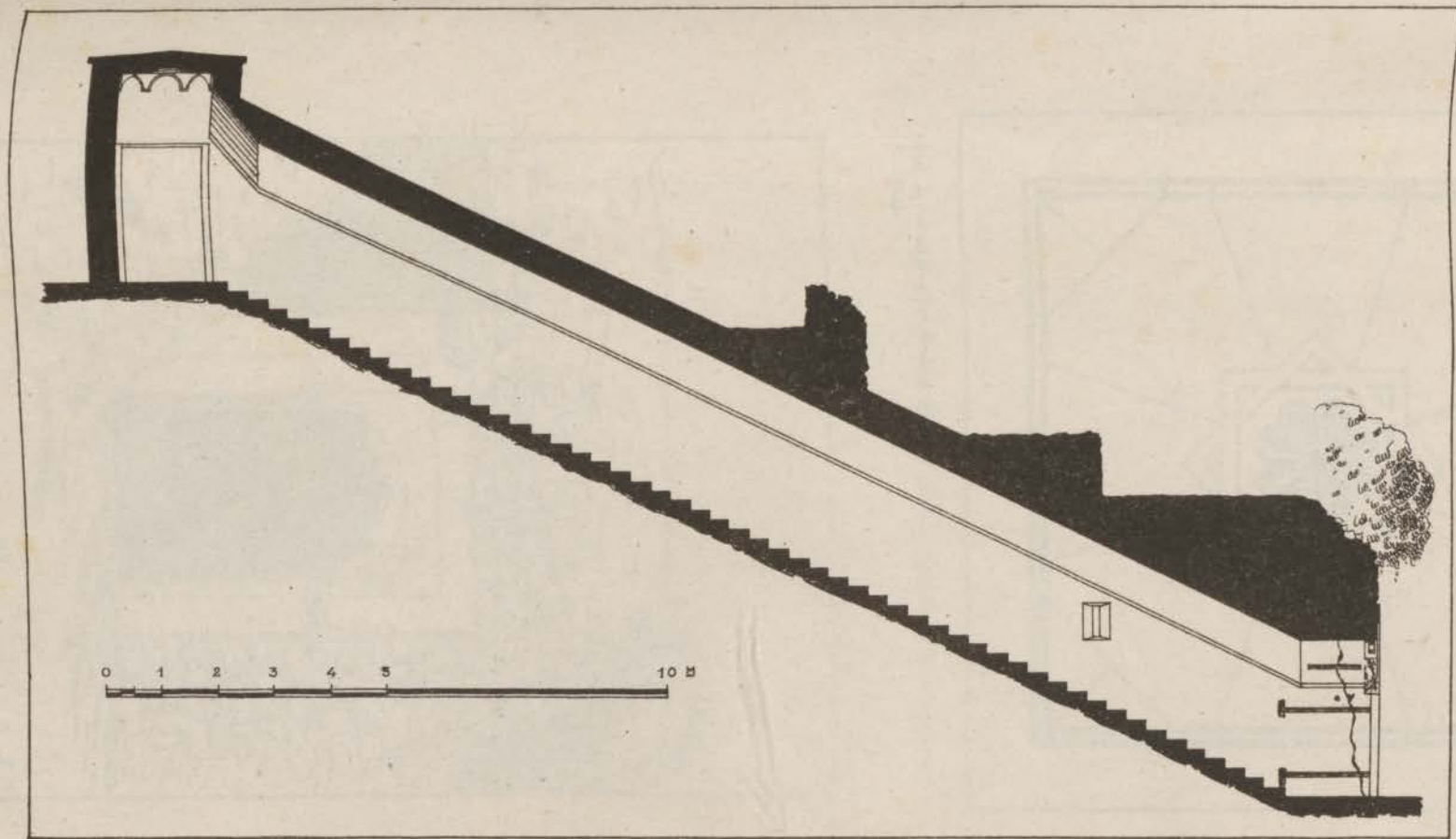
FIG. 92. — Qasba des Oudaïa. Escalier couvert. Coupe.
