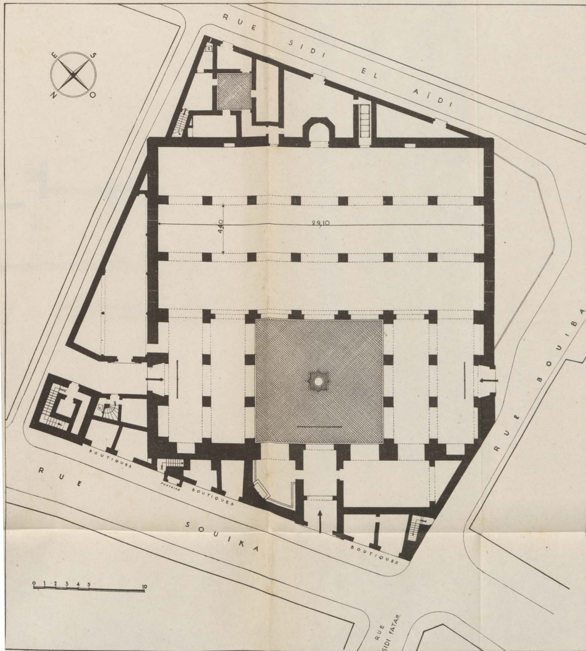
FIG. 153. — Jama Moulay Sliman. Plan.
