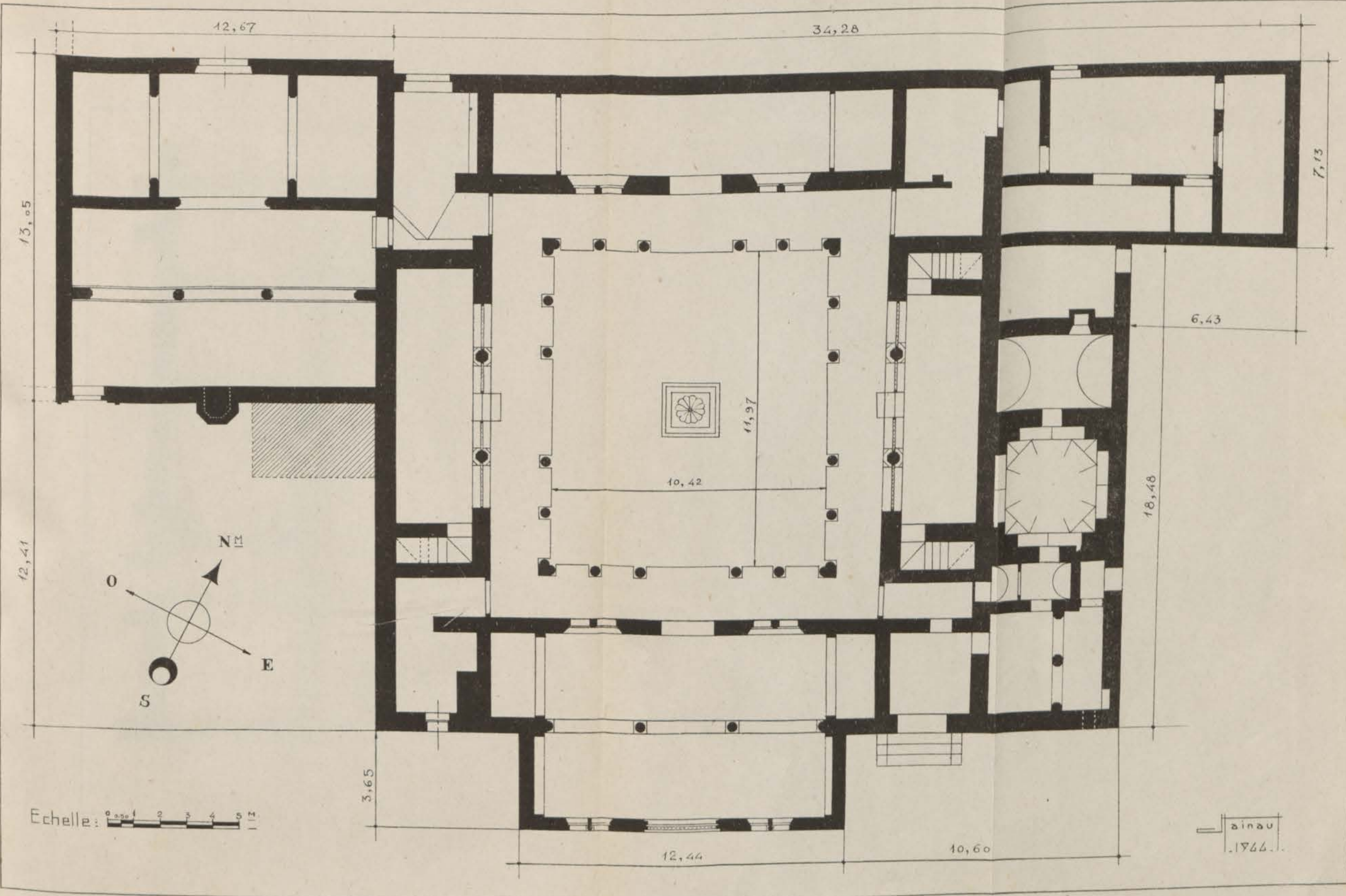
FIG. 108. — Qasba des Oudaia. Bâtiment du musée. Plan actuel.
