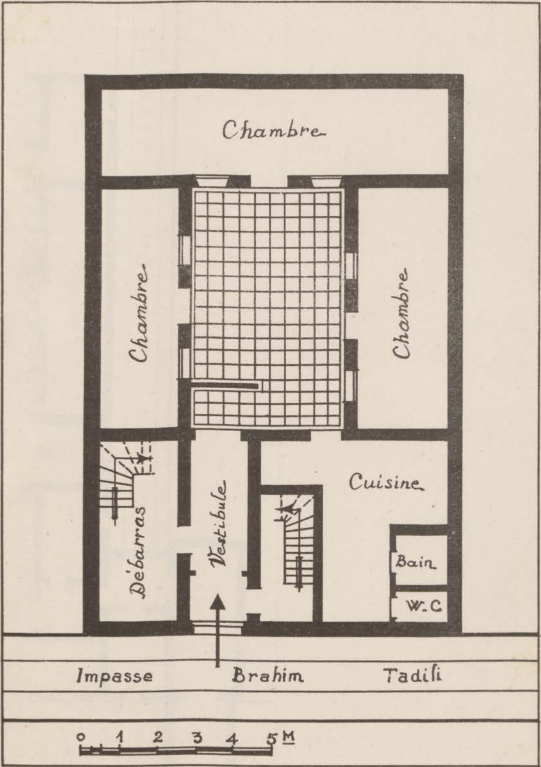
FIG. 175. — Maison d'habitation. Plan.
