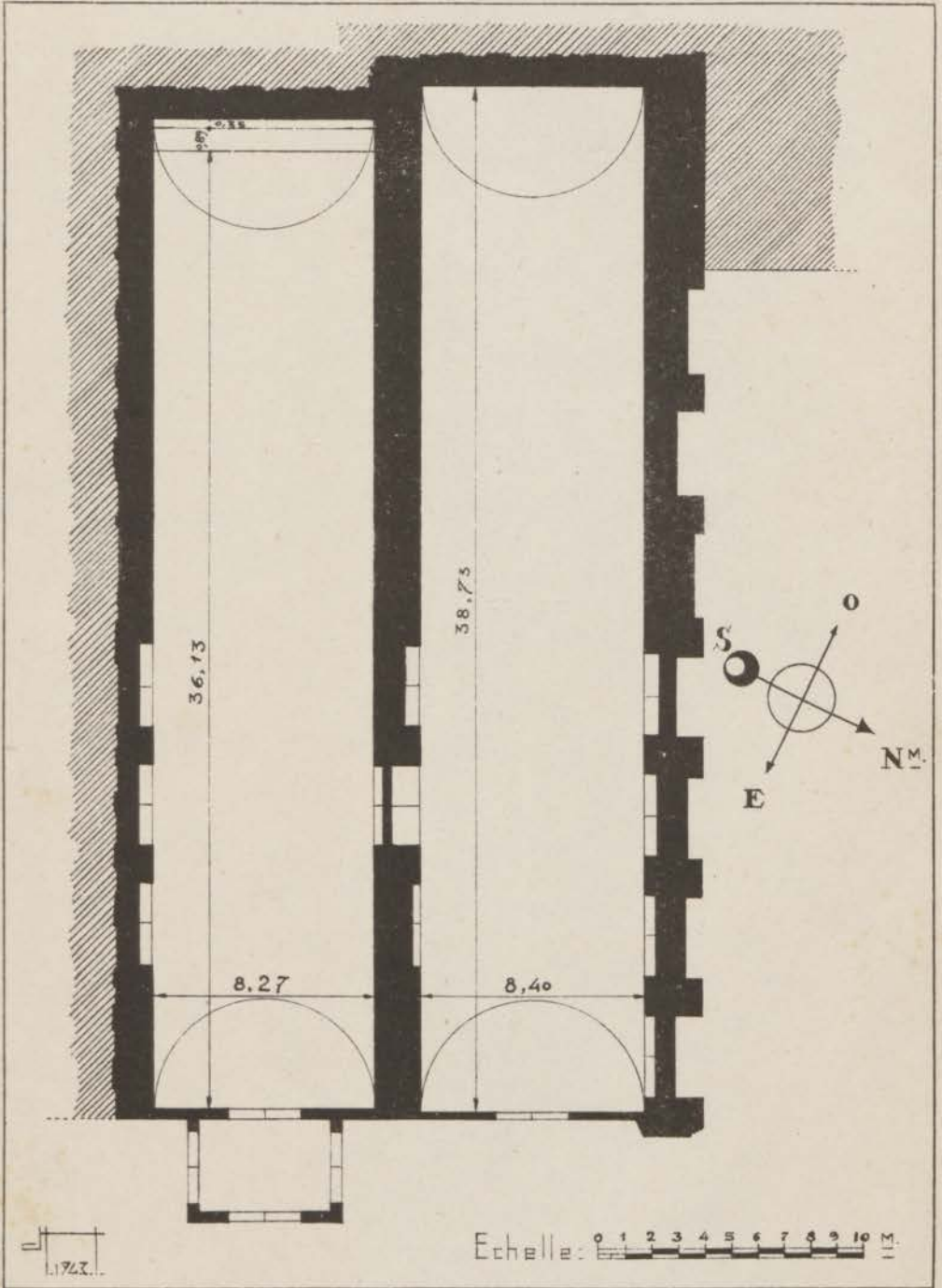
FIG. 178. — Magasins de Sidi Mohammed ben Abdallah. Plan.
