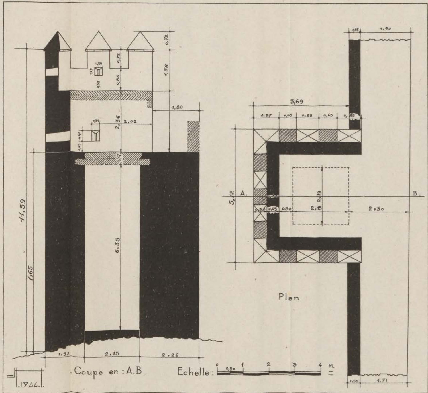
Fig. 32. — Encinte almohade de la ville de Ribat el-Fath. Tour, boulevard Reine (la cinquième à l'est de la porte des Zaer). Coupe et plan.
