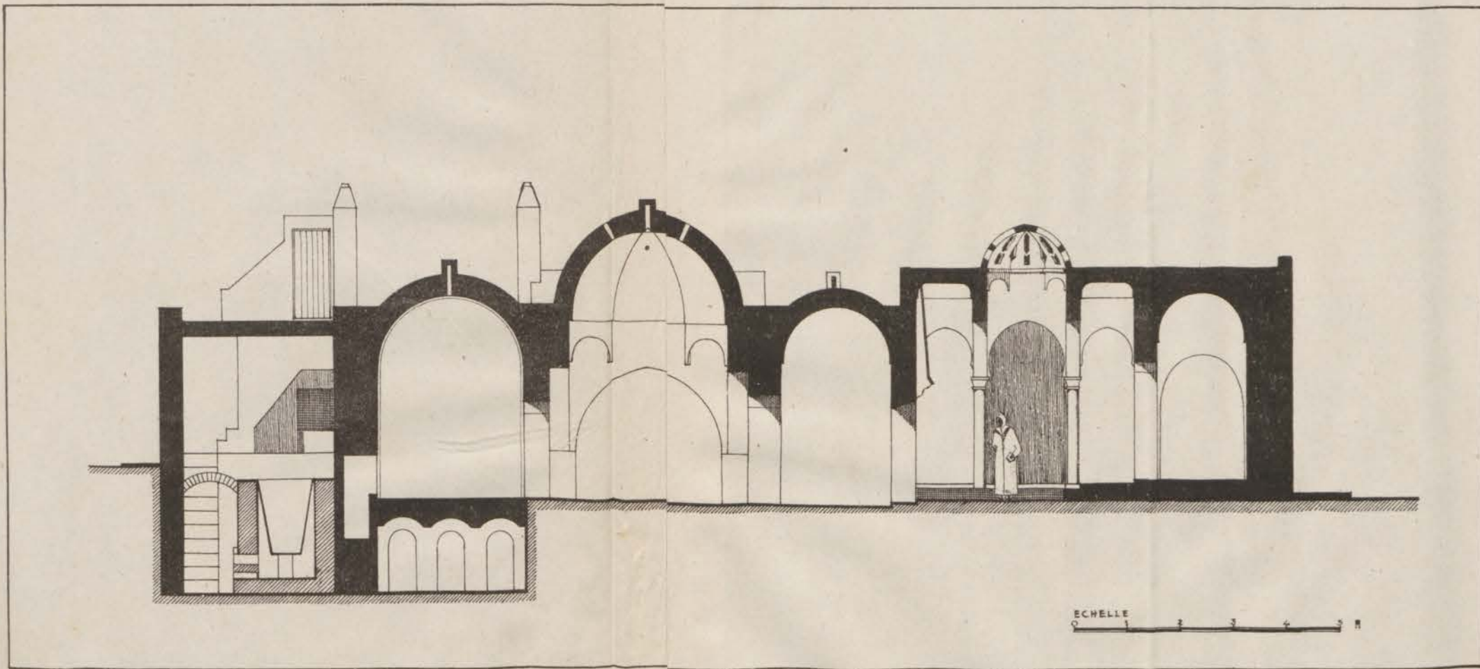
FIG. 76. — Hammam el-Jdid. Coupe.
