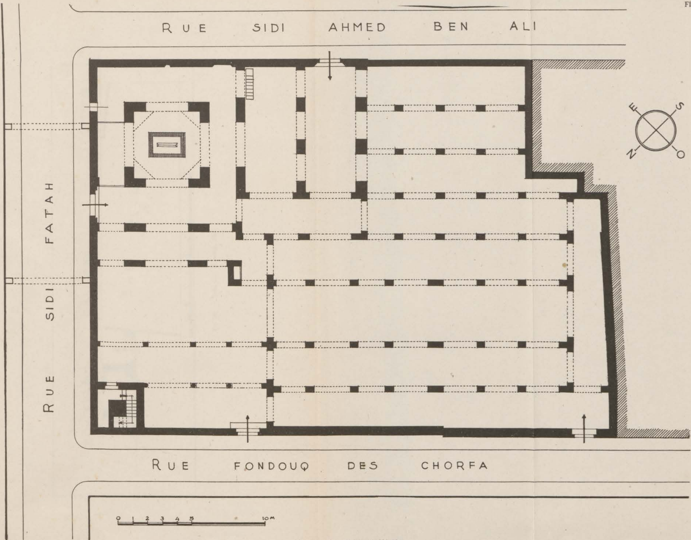
FIG. 160. — Jama Moulay el-Mekki. Plan.
