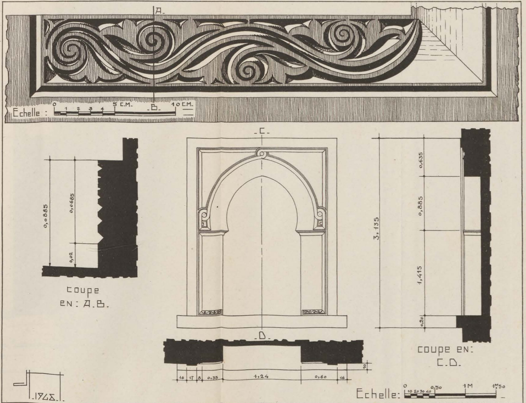
FIG. 30. — Qasba des Oudaïa. Arcade aveugle du rempart, entre la grande Porte et la tour à pans coupés. Plan, coupe, élévation et détail du décor.
