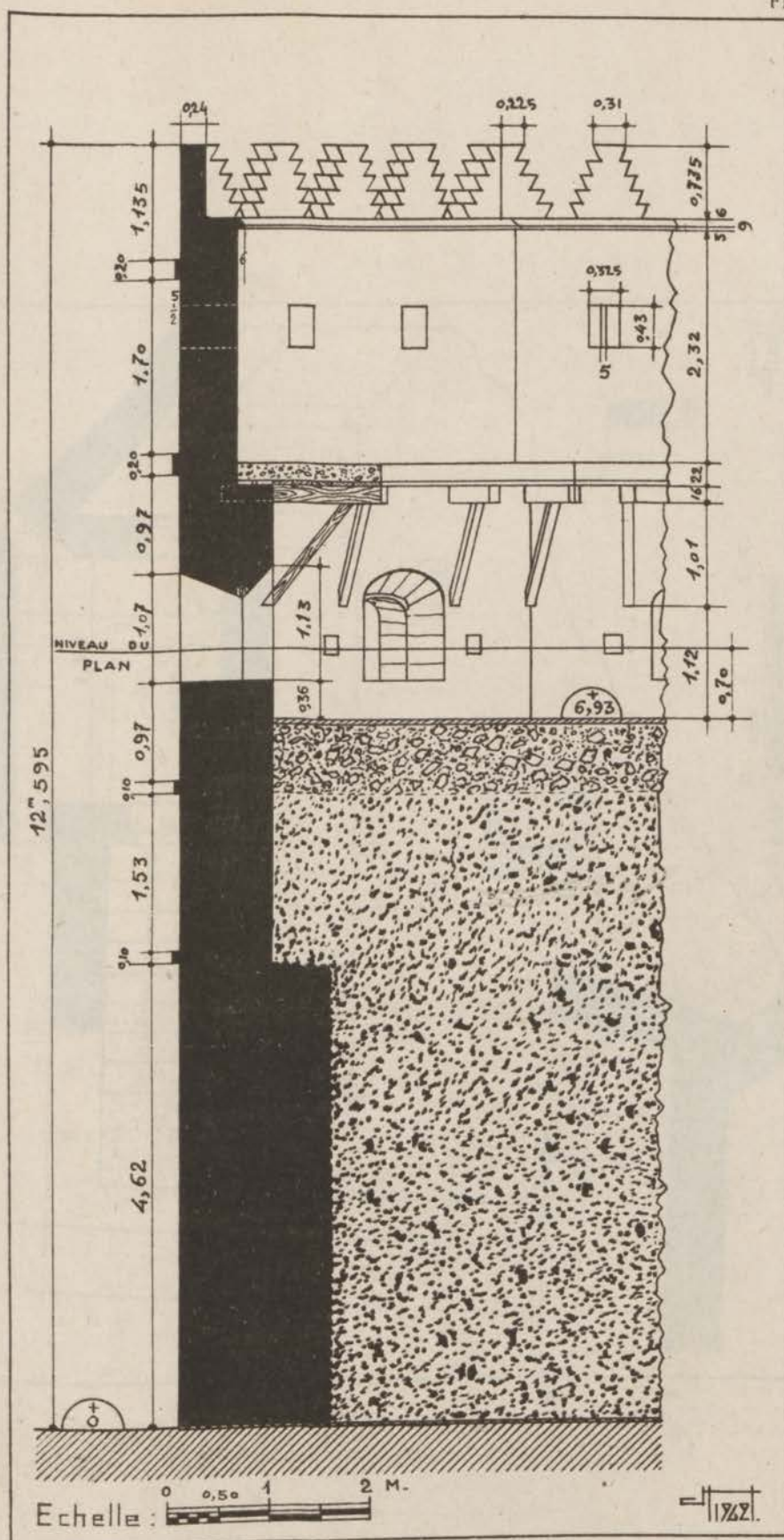
FIG. 102. — Qasba des Oudaïa. Enceinte de Moulay er-Rechid. Bastion heptagonal. Coupe.
