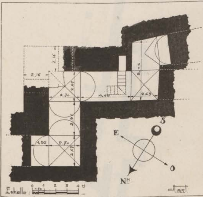
FIG. 78. — Qasba des Oudaia. Souterrain, au-dessous de la propriété du pacha de Marrakech. Plan.
