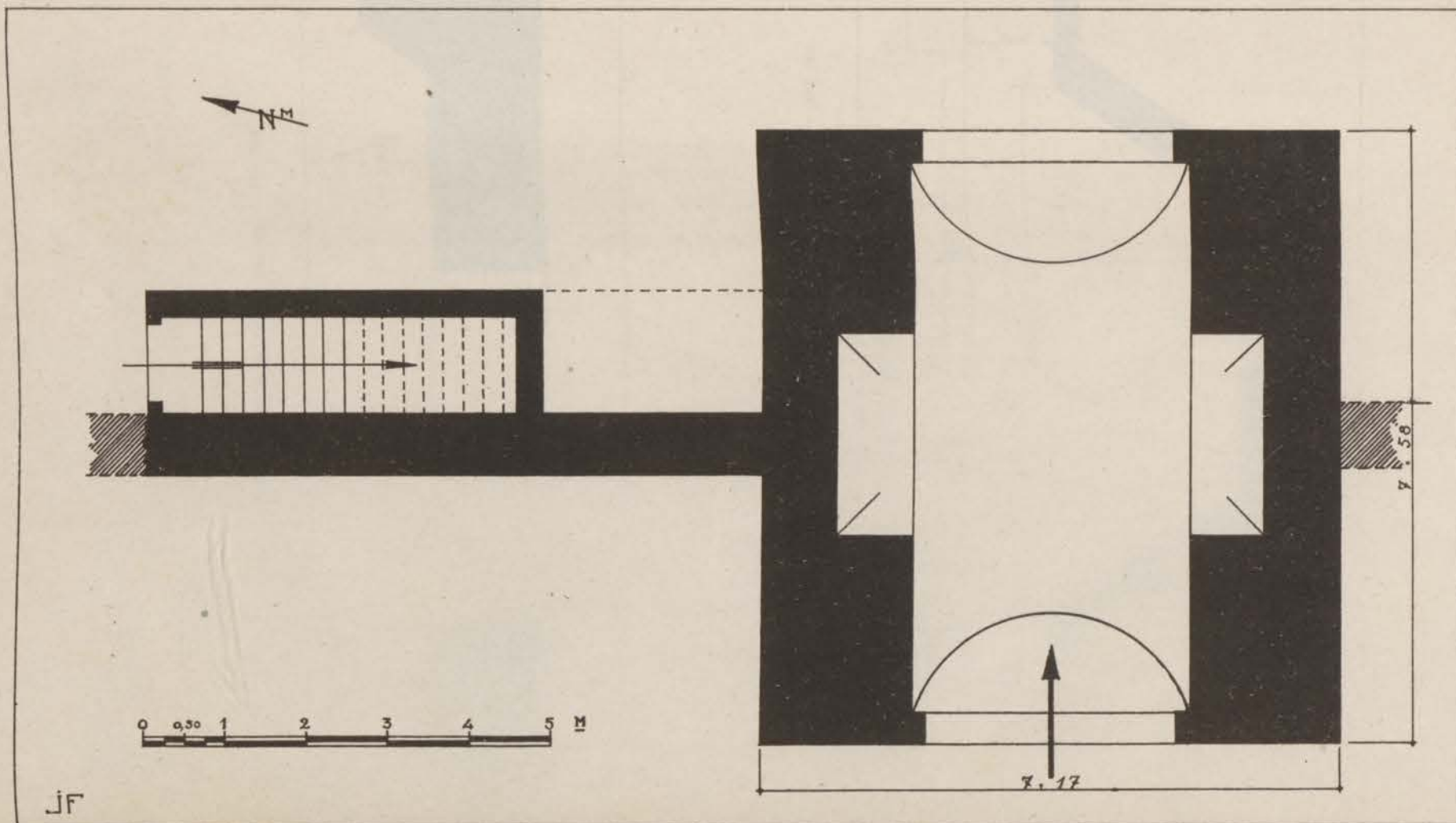
FIG. 126. — Enceinte extérieure alaouite. Bab Marrakech. Plan du rez-de-chaussée.
