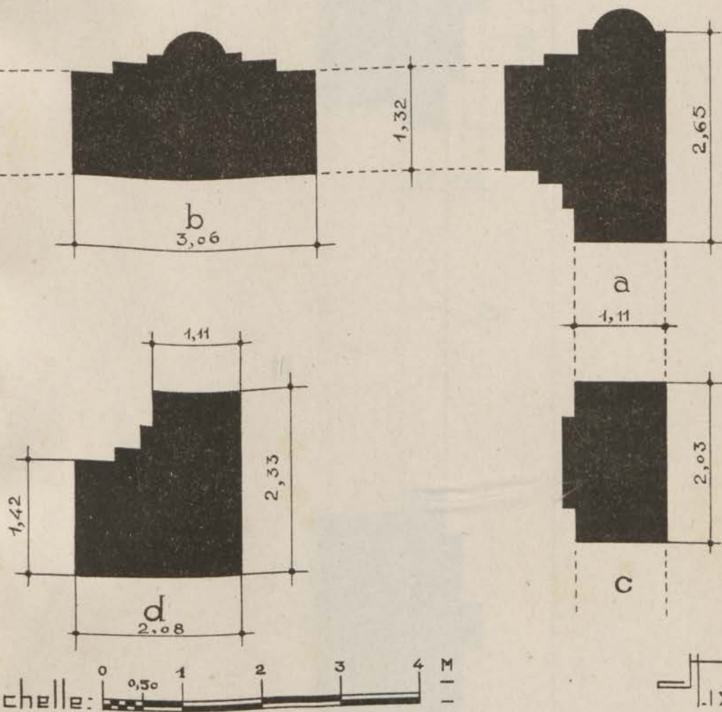
Fig. 59. — Mosquée de Hassan. Plan des piliers bordant les citernes du grand sahn. a, angles sud-est et sud-ouest ; b, face sud ; c, faces est et ouest ; d, angles nord-ouest et nord-est.
