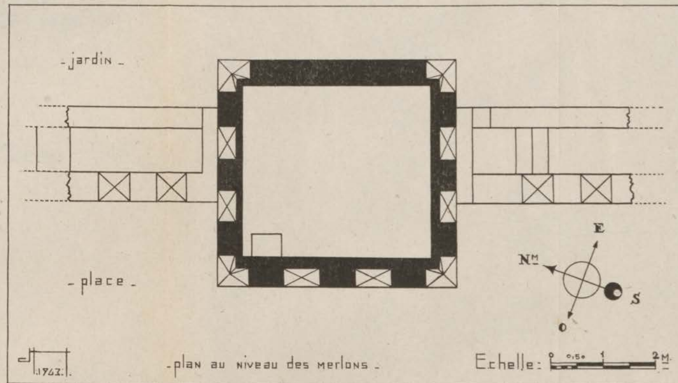
FIG. 99. — Qasba des Oudaia. Encinte de Moulay er-Rechid. Plan d'une tour au niveau des merlons.
