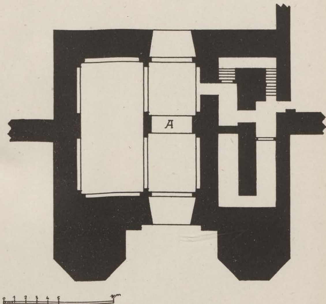
FIG. 51. — Enceinte almohade de la ville de Ribat el-Fath. Porte incluse dans le palais du Sultan. Plan.
