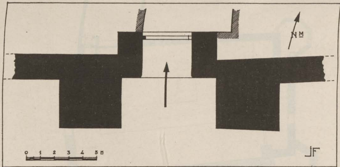
FIG. 96. — Enceinte andalouse de la médina. El Bououtba. Plan.
