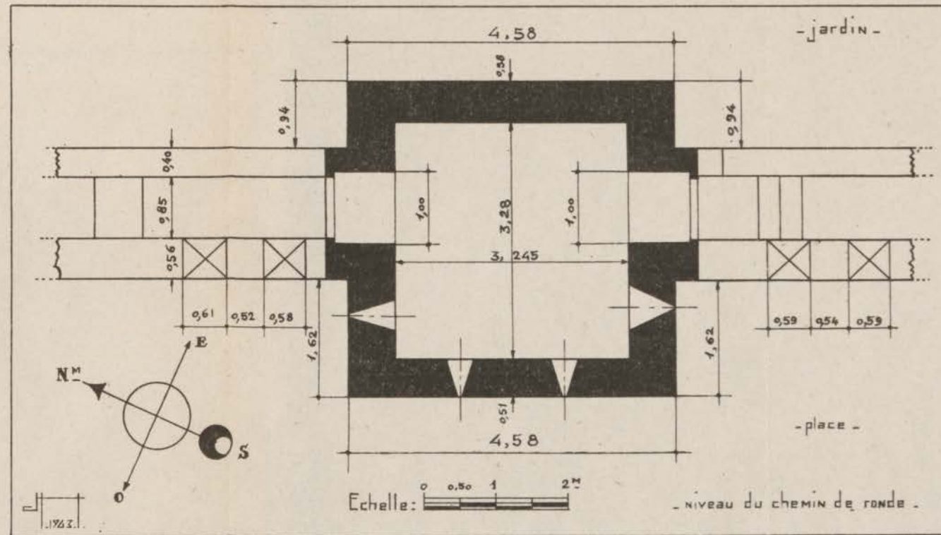
FIG. 98. — Qasba des Oudaia. Encinte de Moulay er-Rechid. Plan d'une tour, au niveau du chemin de ronde.
