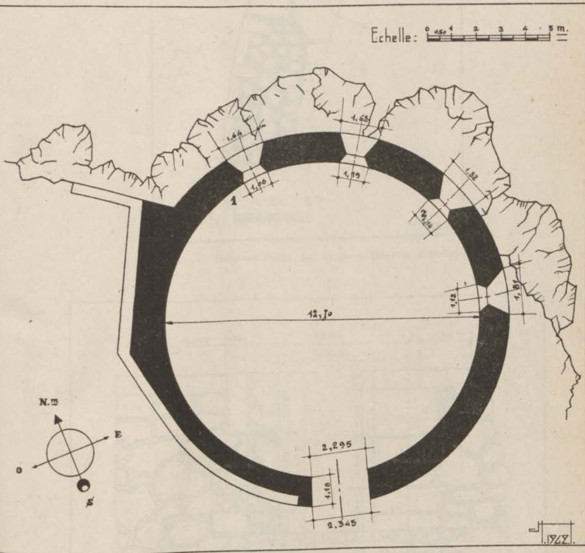
FIG. 113. — Qasba des Oudaia. Borj circulaire. Plan.
