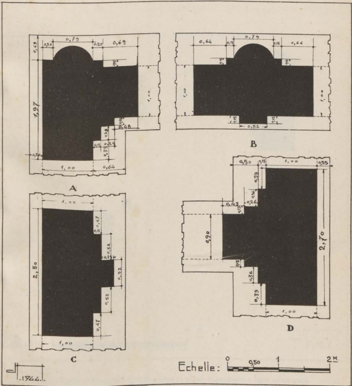
FIG. 58. — Mosquée de Hassan. Plan des piliers bordant les sahs latéraux. A, angle II-14; B, faces nord; C, faces latérales; D, angle V-6.
