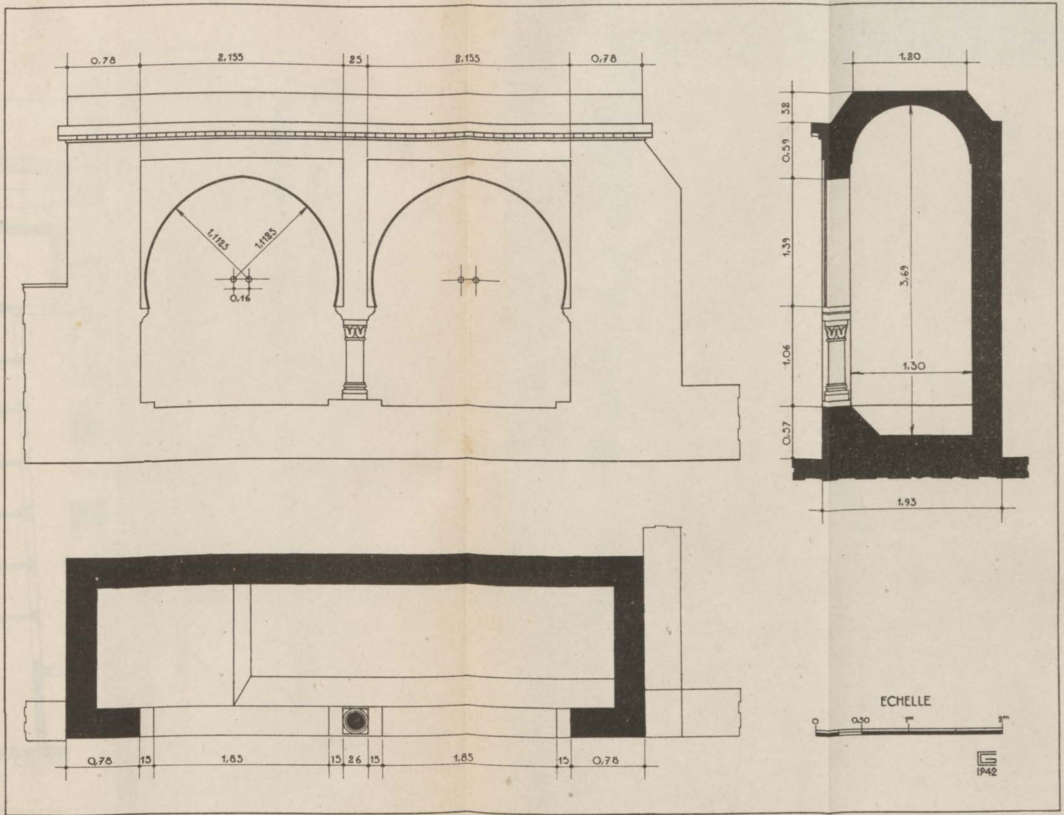
FIG. 183. — Fontaine du Foyer scolaire. Plan, coupe et élévation.
